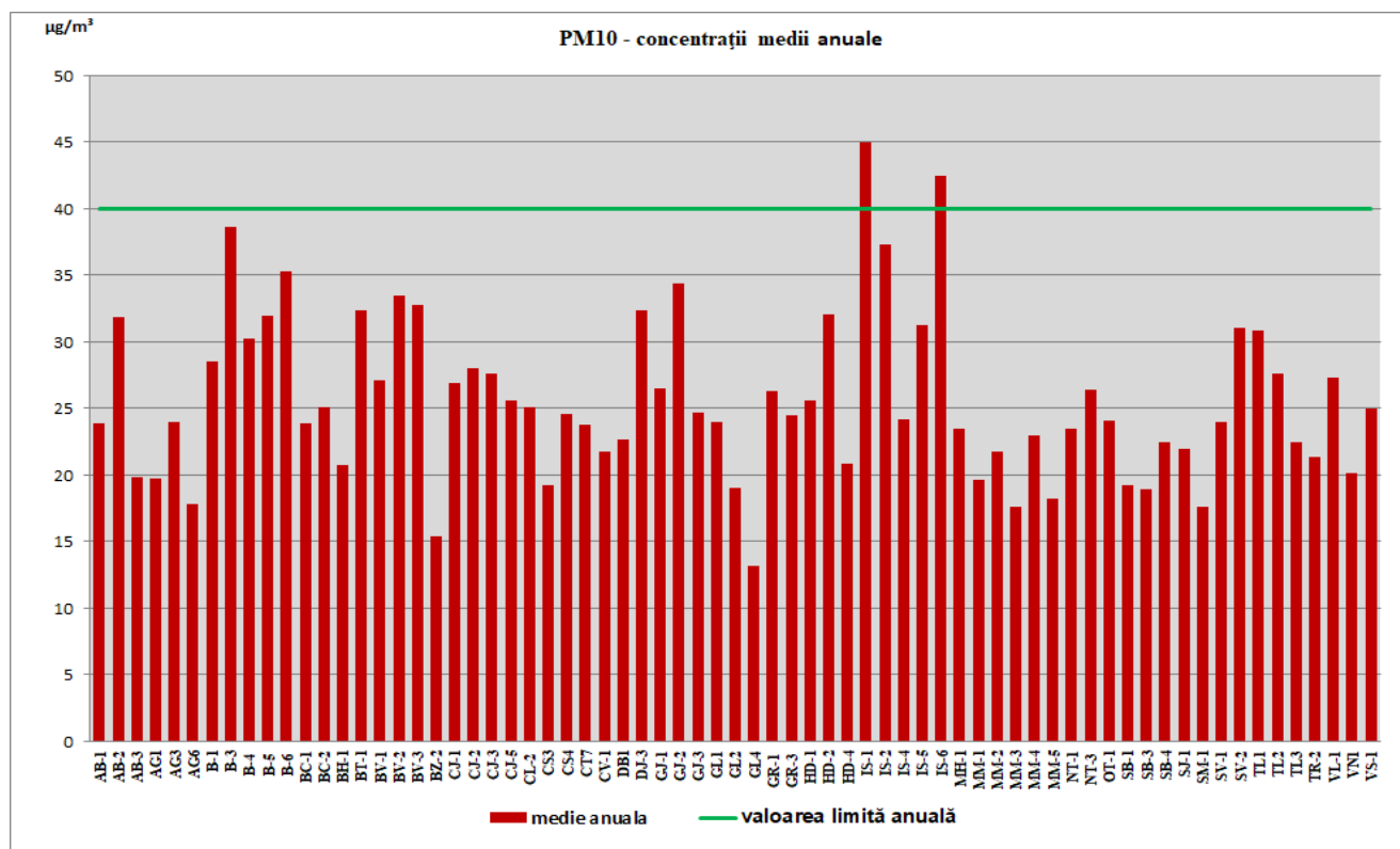
Fig. 6 Particule în suspensie (PM 10 ) - concentrații medii anuale 2018
