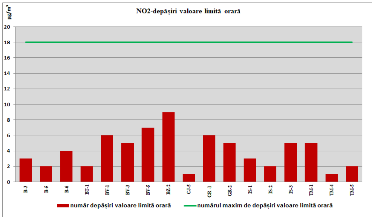
Fig.2 Dioxidul de azot ( NO_2 ) - depășiri ale valorii limită orare 2018
