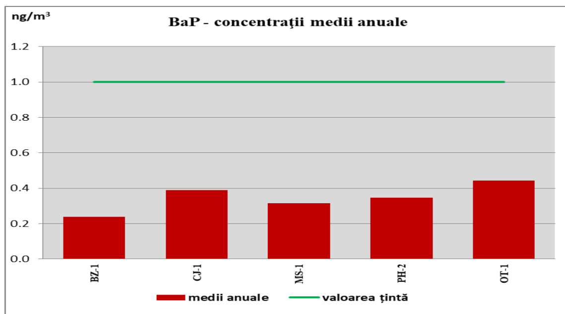
Fig.14 Benzo(a)pirenul (BaP) - concentrații medii anuale 2018
