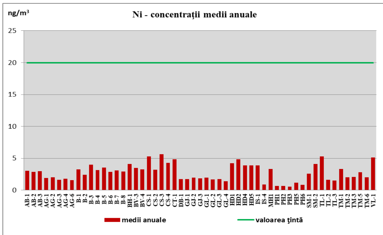
Fig.13 Nichel (Ni) - concentrații medii anuale 2018
