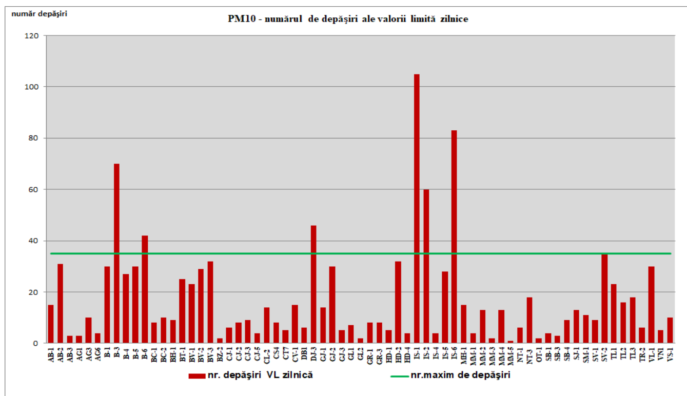
Fig.7 Particule în suspensie ( PM_{10} ) - numărul de depășiri ale valorii limită zilnice 2018
