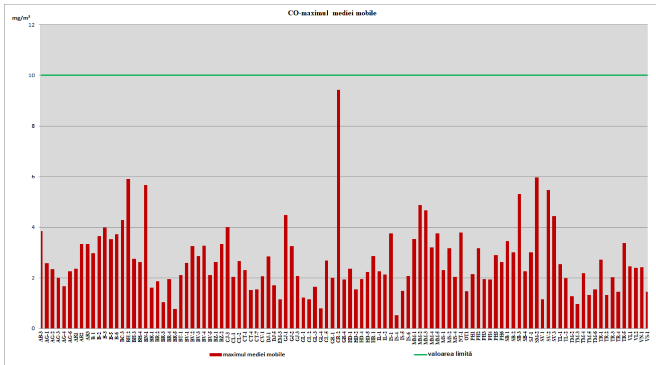
Fig.4 Monoxidul de carbon (CO) - maximul mediei mobile 2018
