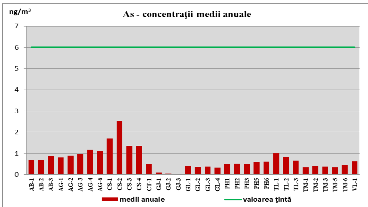
Fig.11 Arsen (As) - concentrații medii anuale 2018
