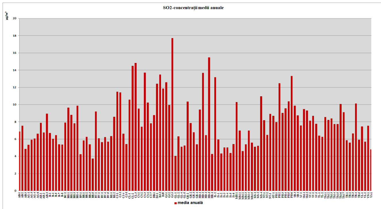
Fig.3 Dioxidul de sulf ( \text{SO}_2 ) - valori medii anuale 2018
