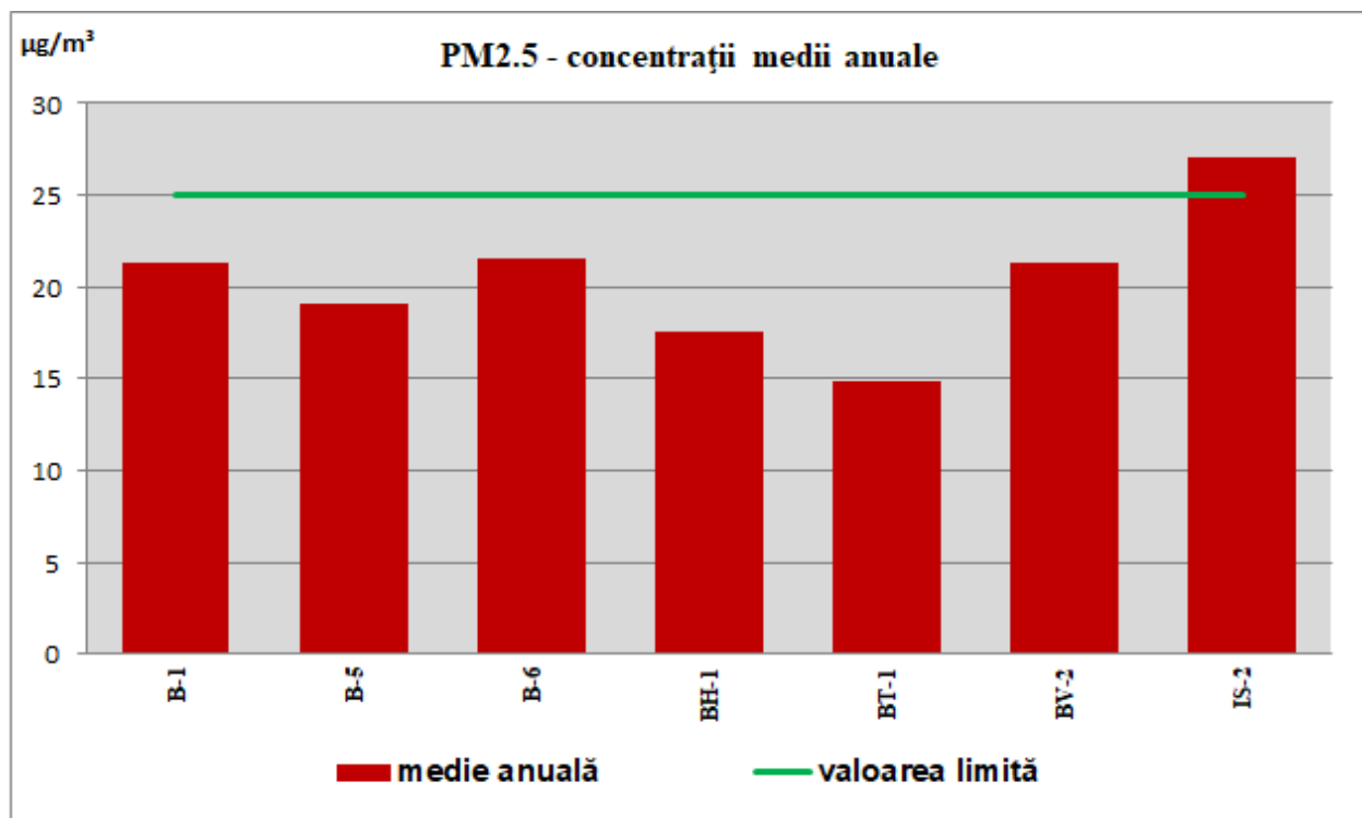
Fig.8 Particule în suspensie ( PM_{2.5} ) - concentrații medii anuale 2018
