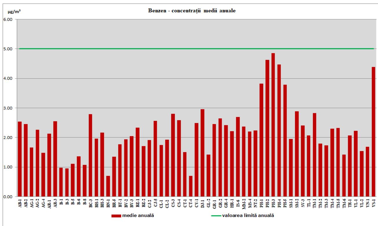
Fig.9 Benzen ( C_6H_6 ) - concentrații medii anuale 2018
