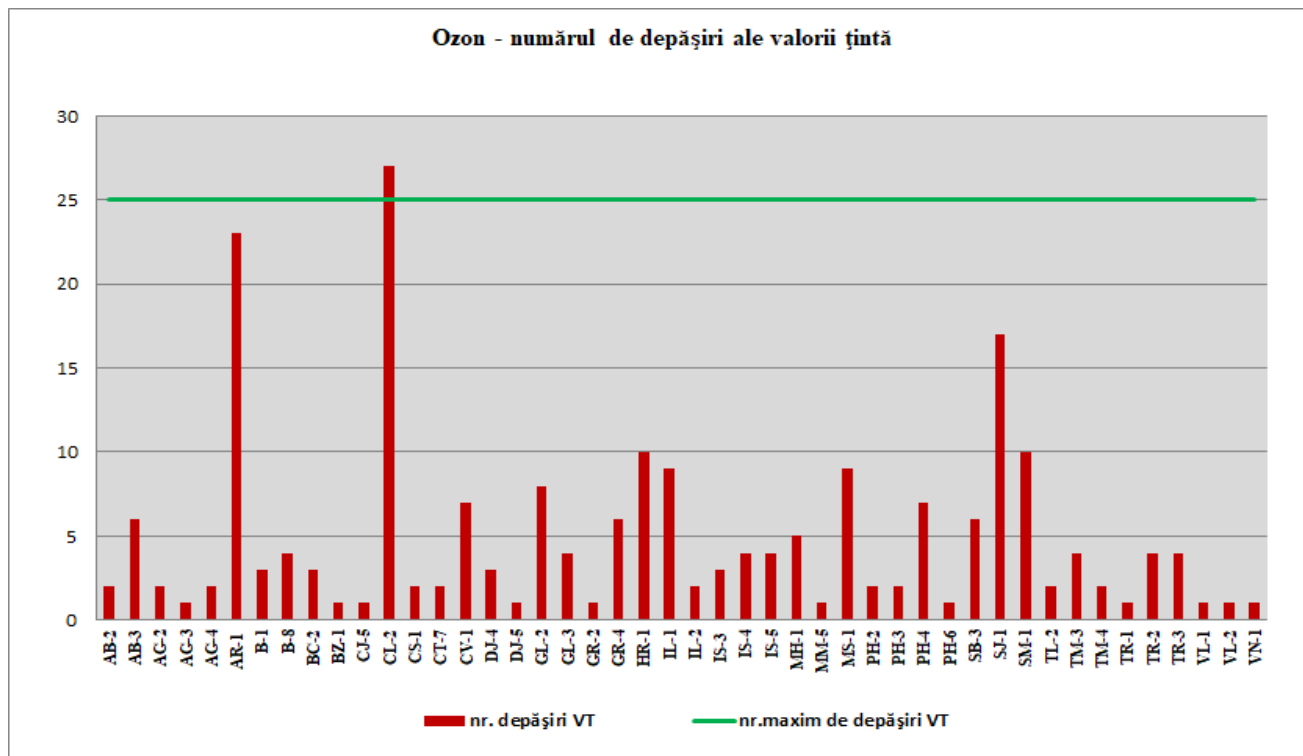
Fig. 5 Ozon ( O_3 ) - numărul de depășiri ale valorii țintă 2018
