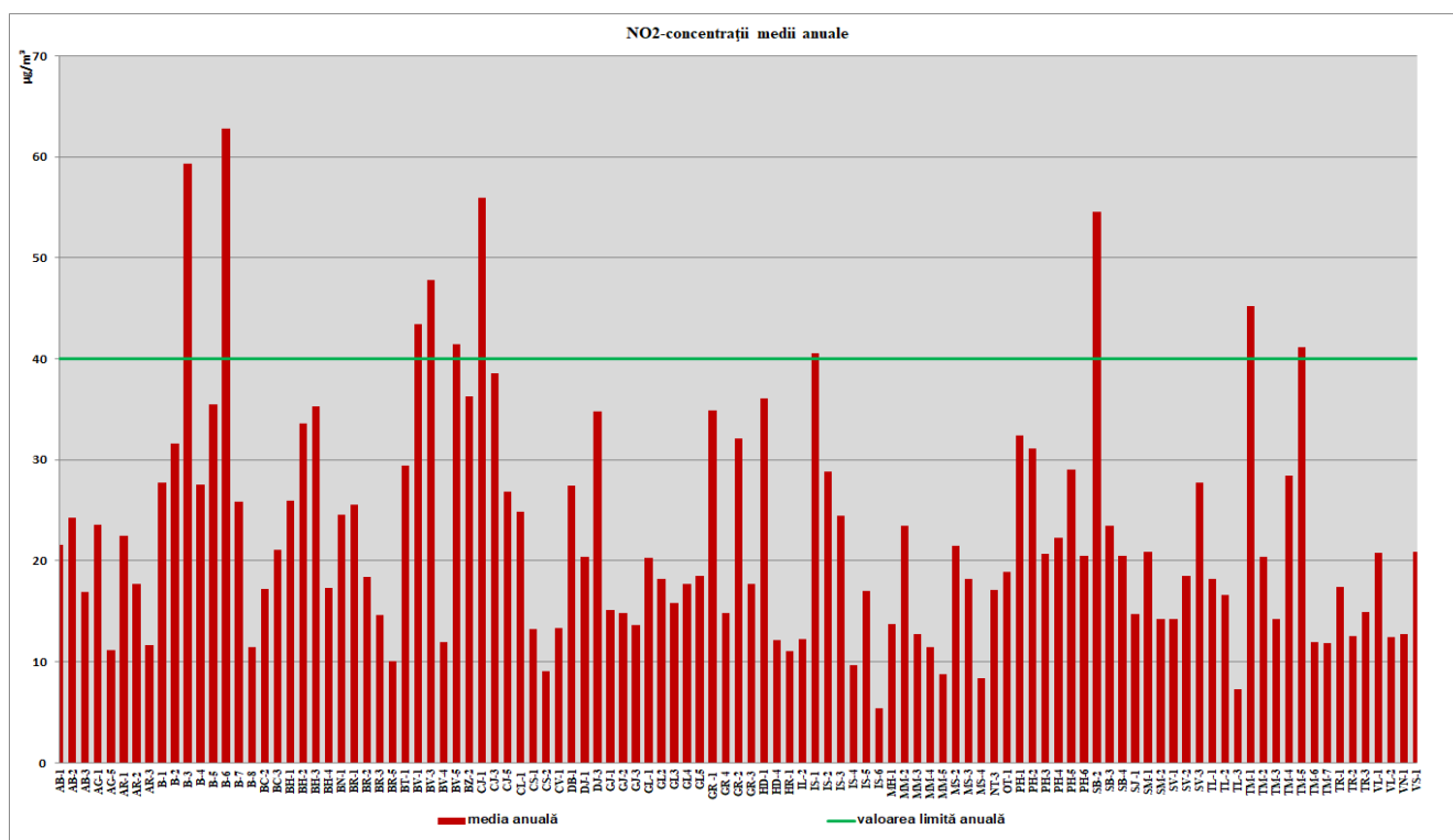
Fig.1 Dioxidul de azot ( \text{NO}_2 ) - valori medii anuale 2018
