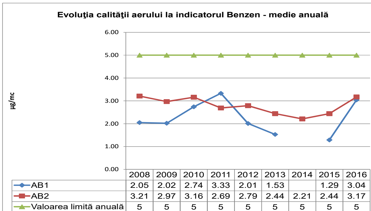
Figura nr. I.1.1.2.5.
