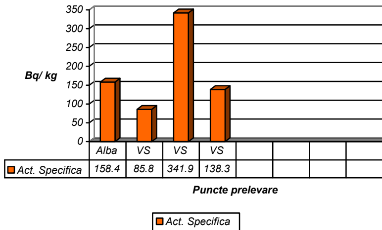
Figura. IX.2.1.3. Activitate beta globală – Vegetație spontană (măsurători 5 zile)
