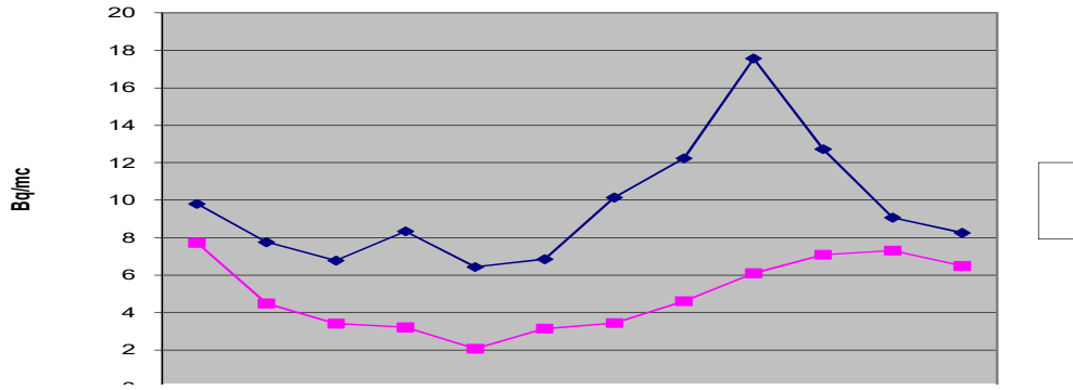
Figuraura IX.1.1.1.5 Variația activității specifice medii lunare a toronului din atmosferă în funcție de variația diurnă( Bq\ m^{-3} ), în anul 2016.
