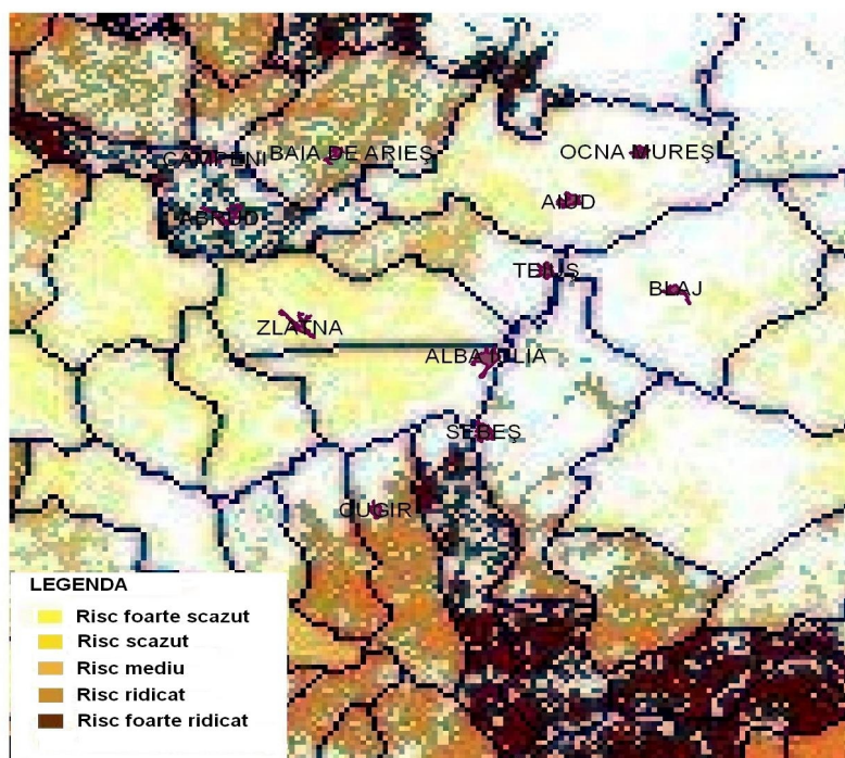
Figura V.1.3.6. Riscul la doboraturi de vant
