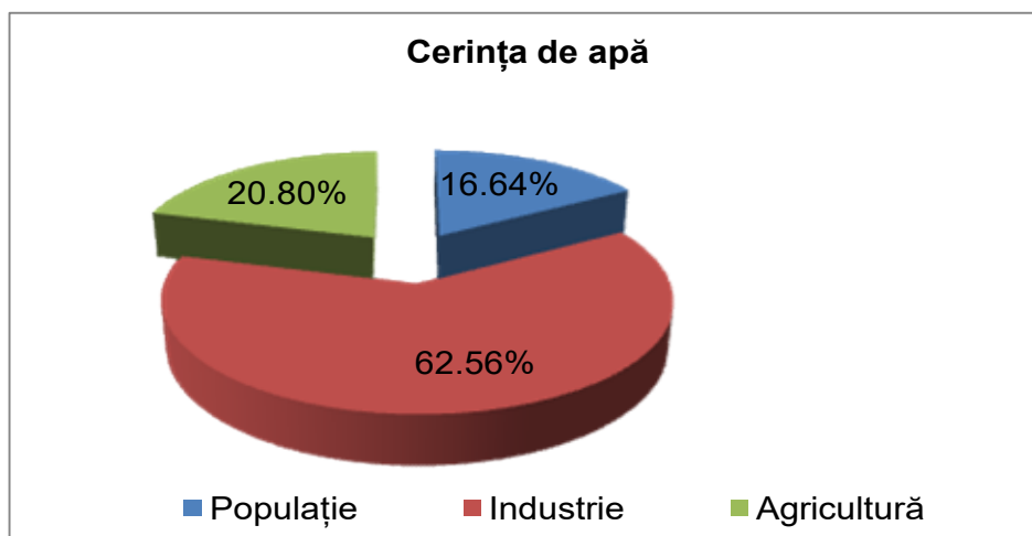
Figura nr. II.1.1.2.1 – Cerința de apă la nivel național
