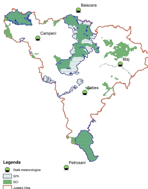
Figura V.1.3.1. Stații meteorologice
