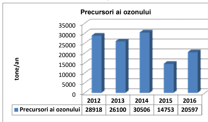
Figura nr. 2.1.2.20. – Emisiile totale de precursori ai ozonului 2012-2016
