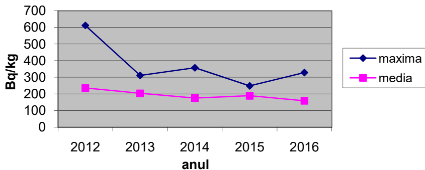
Figura. IX.1.4.1 Variația mediilor și maximelor anuale ale activității beta globale la vegetația spontană în ultimii 5 ani( Bqkg^{-1} )
