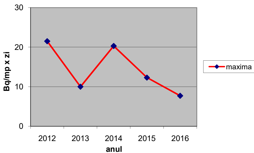
Figura IX.1.1.3.3 Variația valorilor maxime anuale ale activității specifice beta globale imediate ( Bq/m^2 \cdot zi ) la depunerile atmosferice în ultimii 5 ani.
