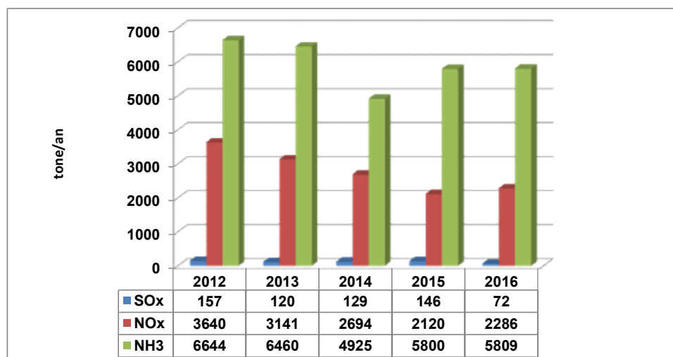
Figura nr. 2.1.2.10. – Emisiile de substanțe acidifiante 2012-2016
