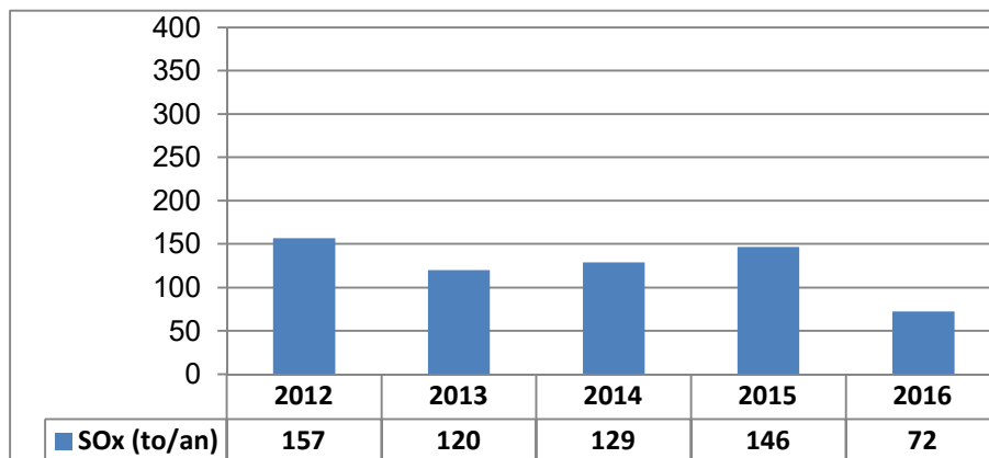
Figura nr . I.2.1.2.1. Evoluția emisiilor de dioxid de sulf în perioada 2012 – 2016
