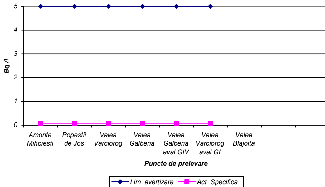
Figura. IX.2.1.1. – Activitate beta globală – Apă de suprafață (măsurători 5 zile)
