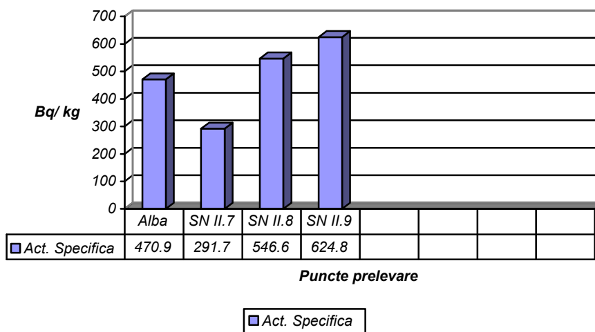
Figura.IX.2.1.2. Activitate beta globală – Sol necultivat (măsurători 5 zile)
