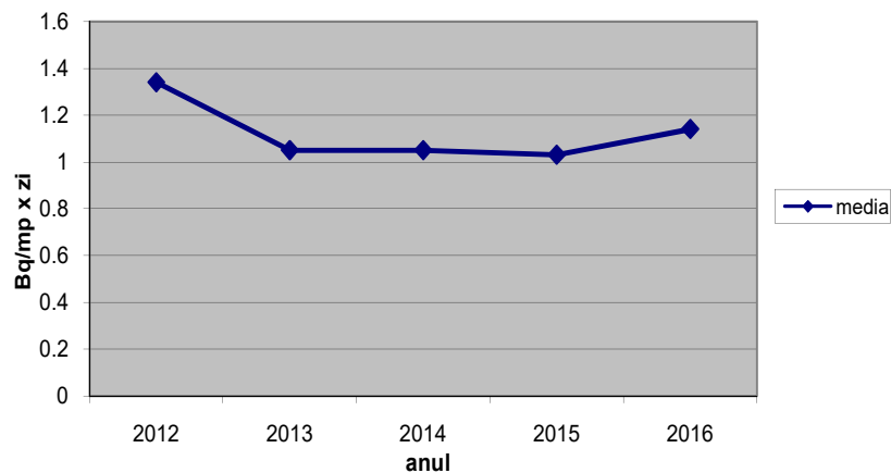
Figura IX.1.1.3.2 Variația medie anuală a activităților specifice beta globale imediate ( Bq/m^2 \cdot zi ) la depunerile atmosferice în ultimii 5 ani.
