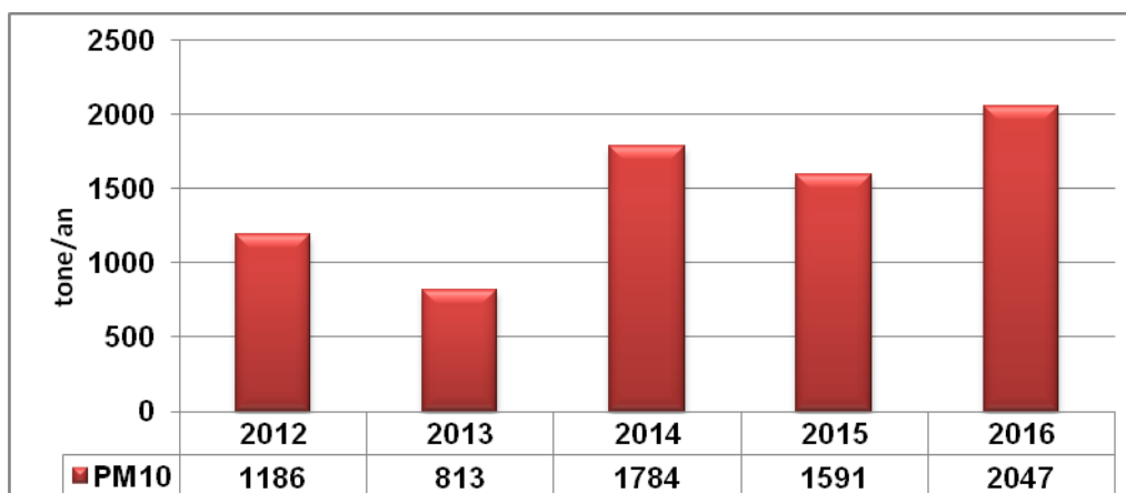
Figura nr. 2.1.1.22. – Evoluția emisiilor de pulberi în suspensie PM 10
