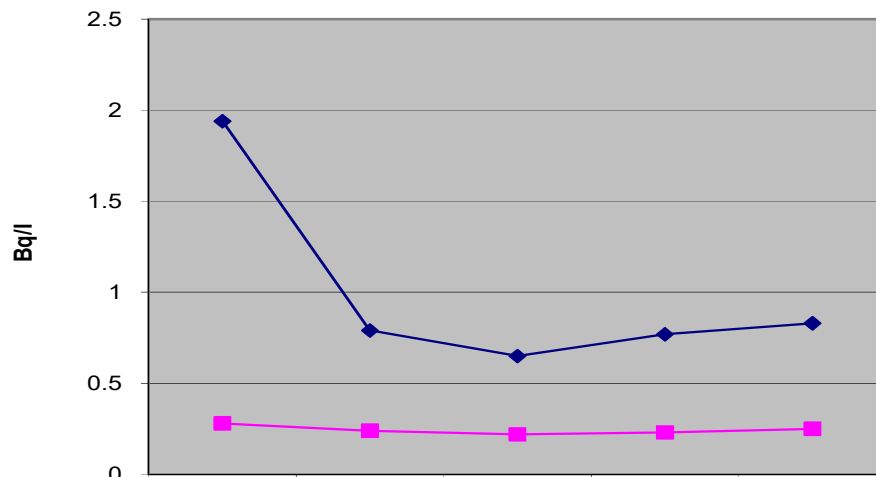
Figura. IX.1.2.2. Variația mediilor și maximelor anuale (măsurători imediate) ale activității beta globale a râului Mureș în ultimii 5 ani (Bq/l)
