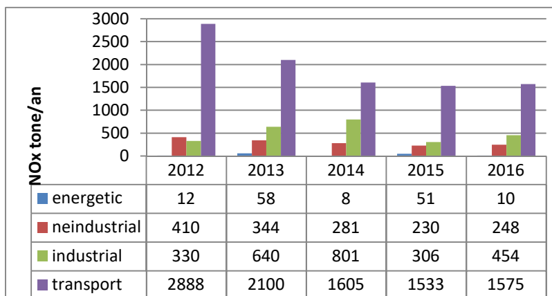
Figura nr. I.2.1.2.5. Evoluția emisiilor de NO x în perioada 2012 – 2016 pe sectoare de activitate
