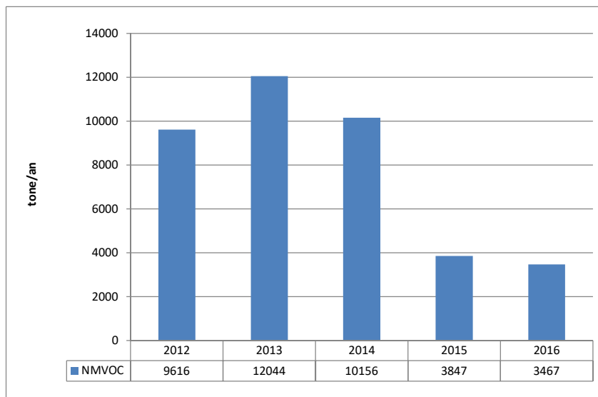
Figura nr. 2.1.2.13. - Evoluția emisiilor de NMVOC în perioada 2012 - 2016
