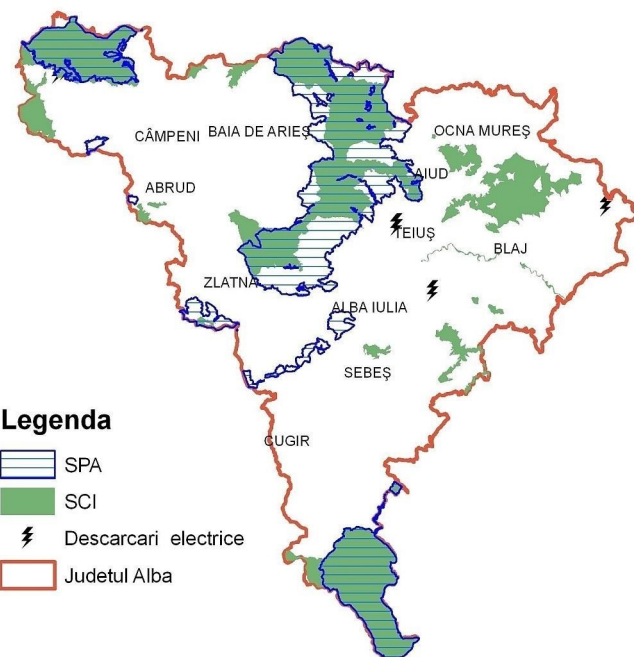
Figura V.1.3.5. Localizarea fenomenelor de descarcari electrice in perioada 2010 - 2016
