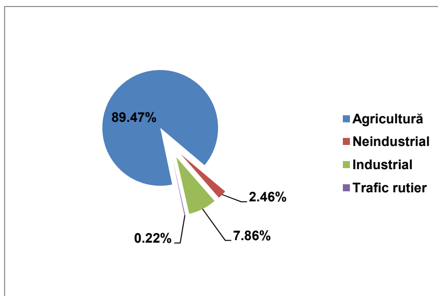
Figura nr. 2.1.2.9. – Surse de emisie de amoniac
