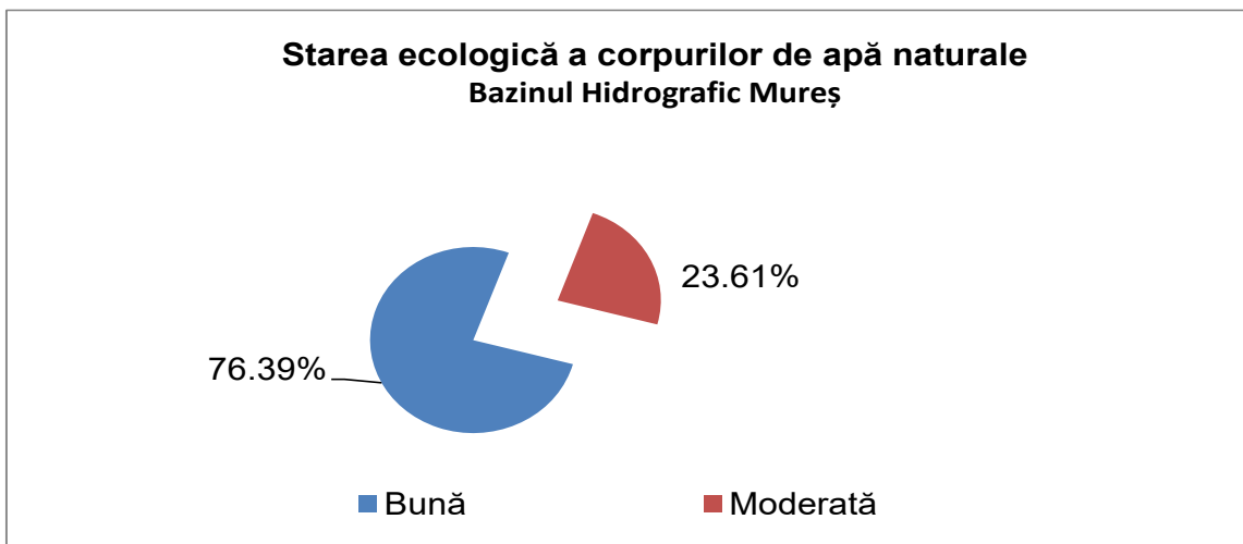
Figura nr. 2.1.1.1 Starea ecologică a corpurilor naturale de apă de suprafață
