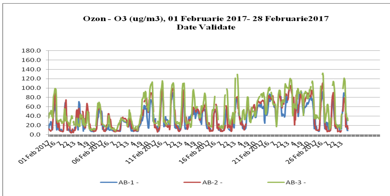
Figura. 1.1.4.1 Ozon – valori orare
