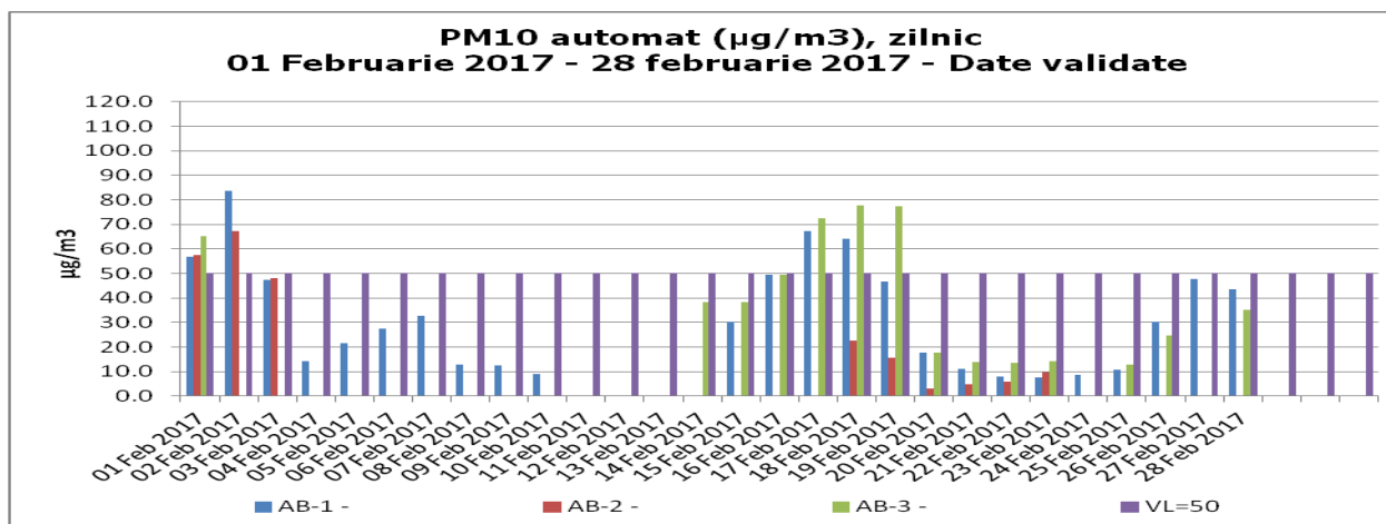
Figura. 1.1.6.1 Pulberi în suspensie PM 10 – metoda automată
