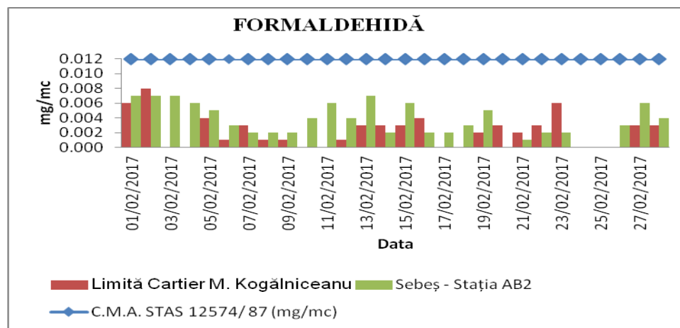
Figura. 1.2.1.1 – Aldehydă formică – Municipiul Sebeș
