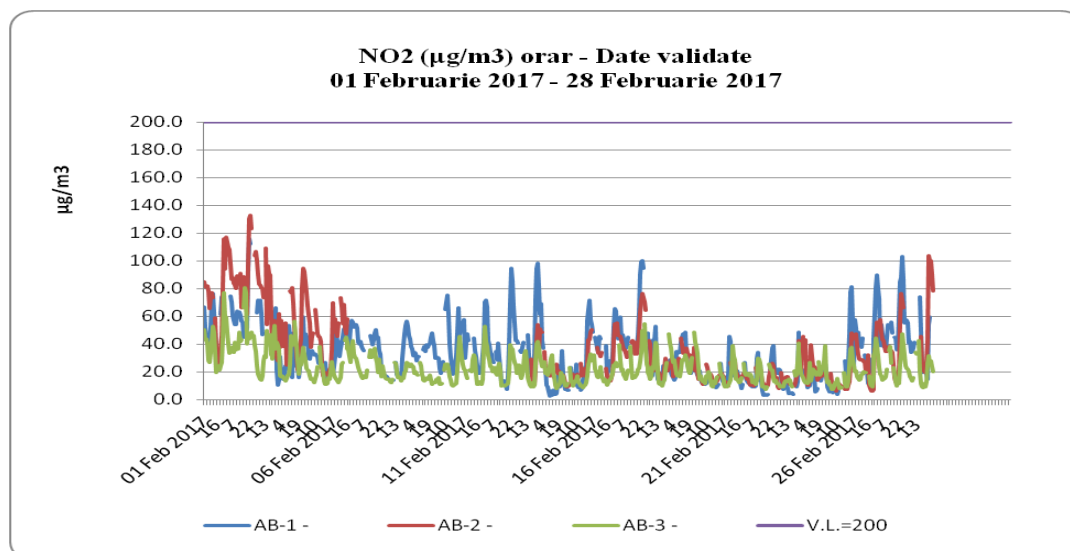
Figura 1.1.1 – Dioxid de azot
