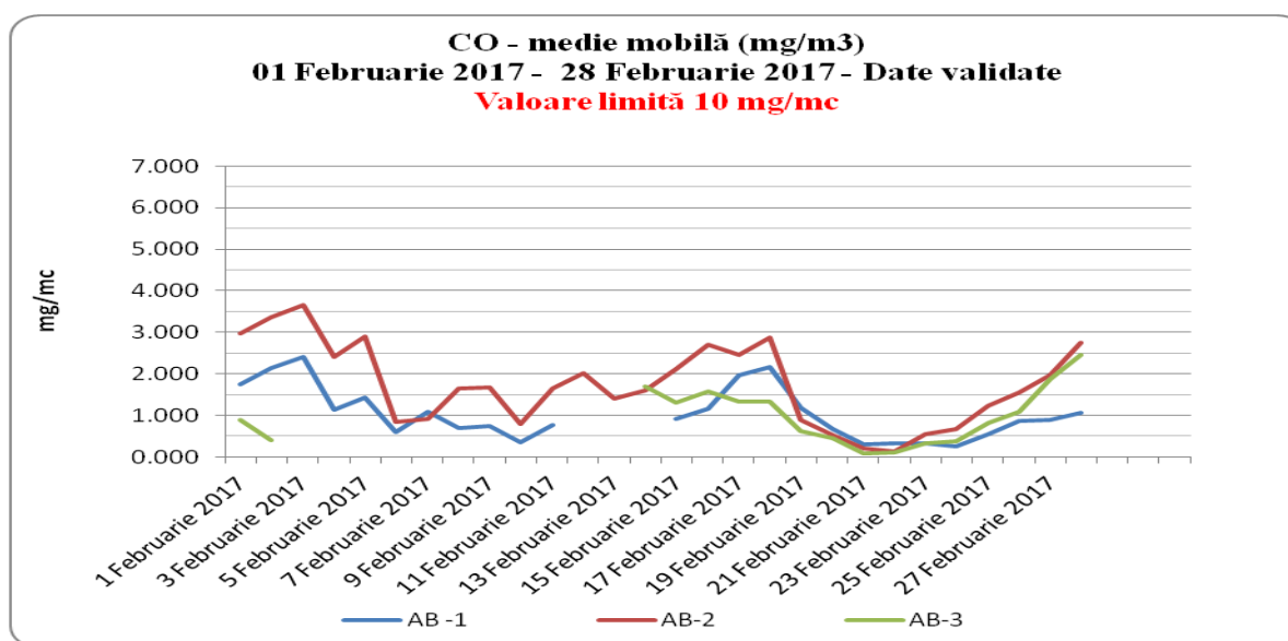
Figura. 1.1.3 – Monoxid de carbon – medie mobilă
