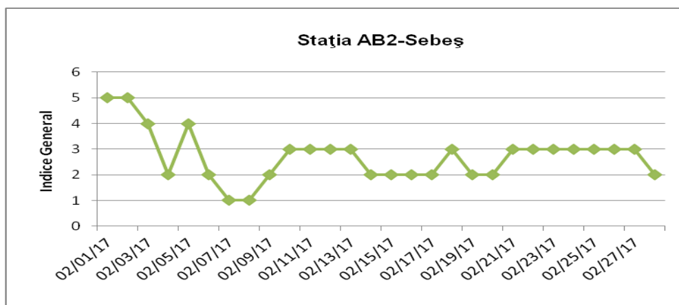
Figura. 1.1.7.3 – Indicele general de calitate a aerului – AB2
