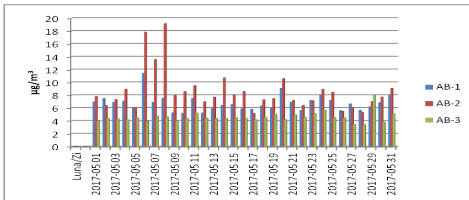
Figura. 1.1.2.2 Dioxid de sulf – media la 24 ore
