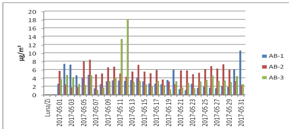
Figura. 1.1.6.1 Pulberi în suspensie PM 10 – metoda automată
