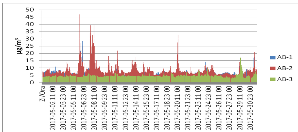
Figura. 1.1.2.1 – Dioxid de sulf – valori orare
