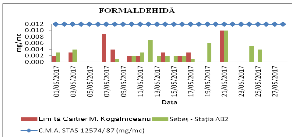
Figura. 1.2.1.1 – Aldehidă formică – Municipiul Sebeș
