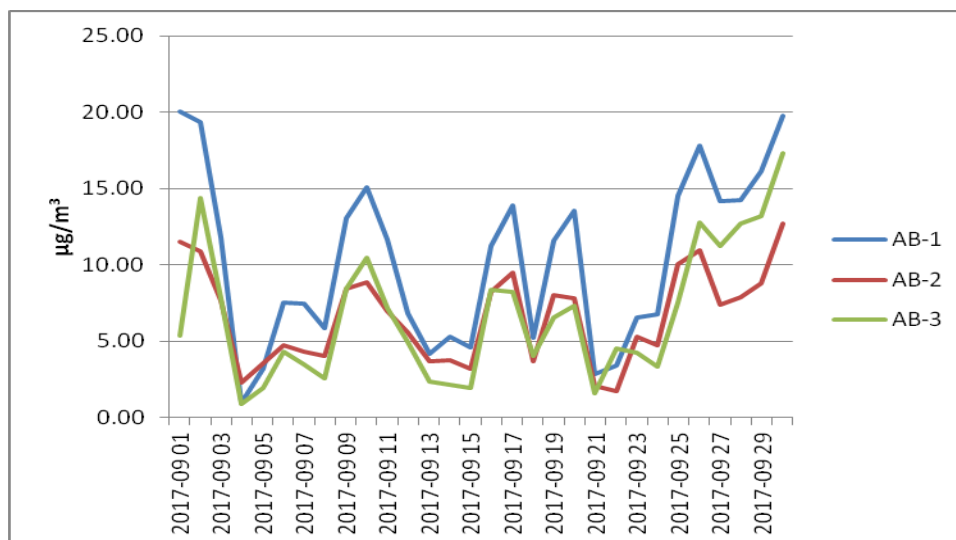
Figura. 1.1.6.1 Pulberi în suspensie PM 10 – metoda automată
