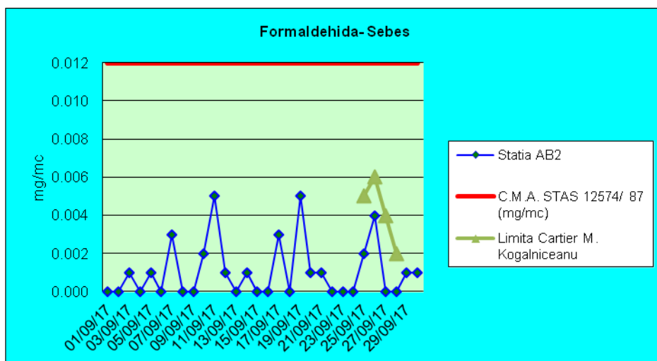
Figura. 1.2.1.1 – Aldehydă formică – Municipiul Sebeș
