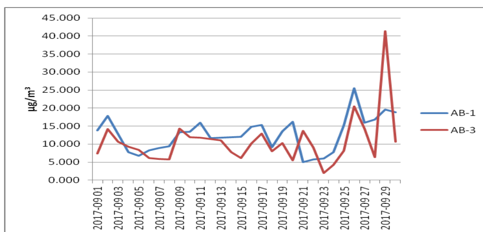
Figura. 1.1.6.2 Pulberi în suspensie PM 10 – metoda gravimetrică
