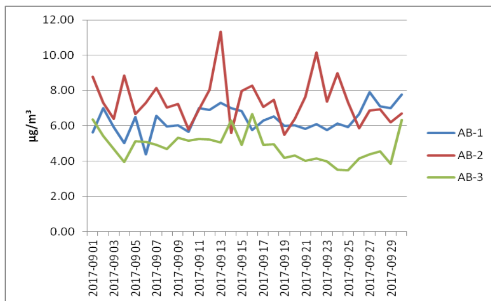
Figura. 1.1.2.2 Dioxid de sulf – media la 24 ore
