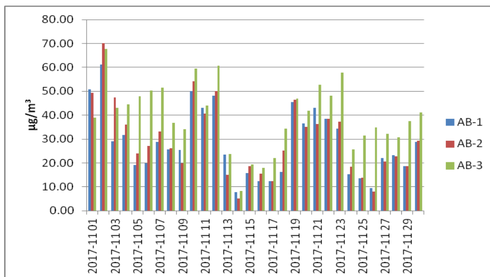
Figura. 1.1.4.2 Ozon – medie mobilă
