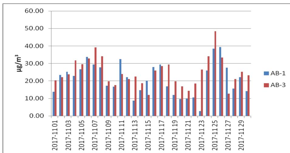
Figura. 1.1.6.2 Pulberi în suspensie PM 10 – metoda gravimetrică
