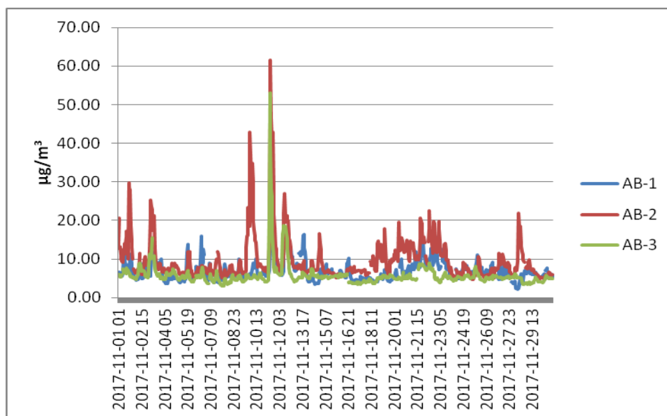
Figura. 1.1.2.1 – Dioxid de sulf – valori orare
