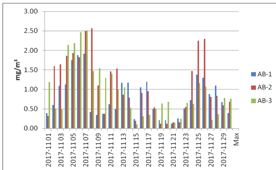
Figura. 1.1.3 – Monoxid de carbon – medie mobilă
