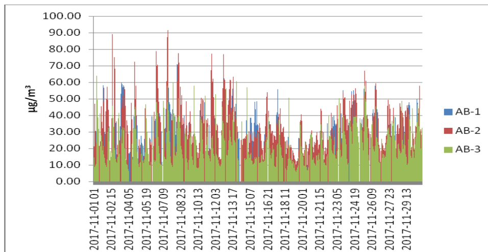
Figura 1.1.1 – Dioxid de azot - valori orare
