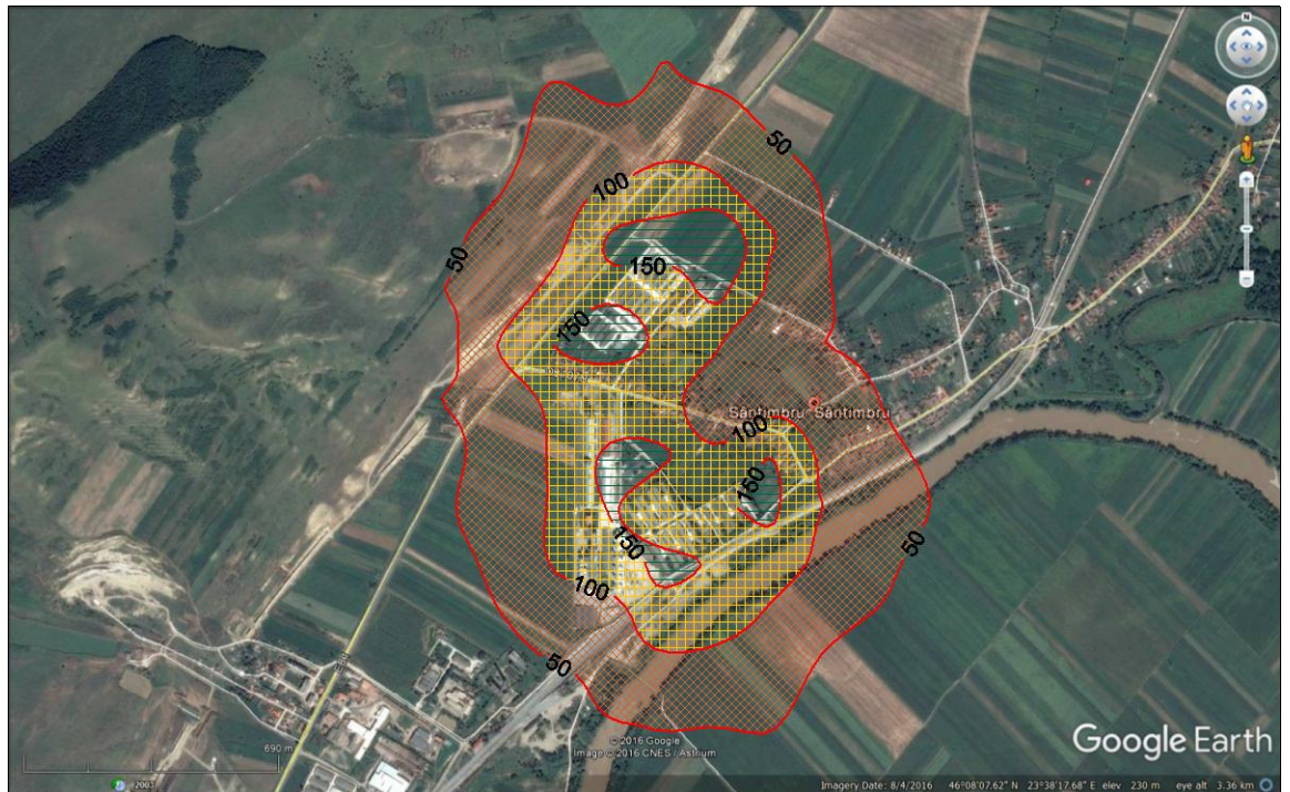
Figura 5: Concentratii maxime de amoniac in aer – timp de mediere 30 min (fermele 3 si 4 Santimbru)
