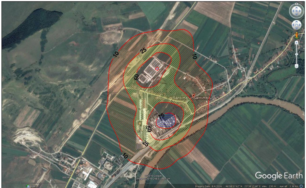
Figura 6: Concentratii maxime de amoniac in aer – timp de mediere 24 ore (fermele 3 si 4 Santimbru)
