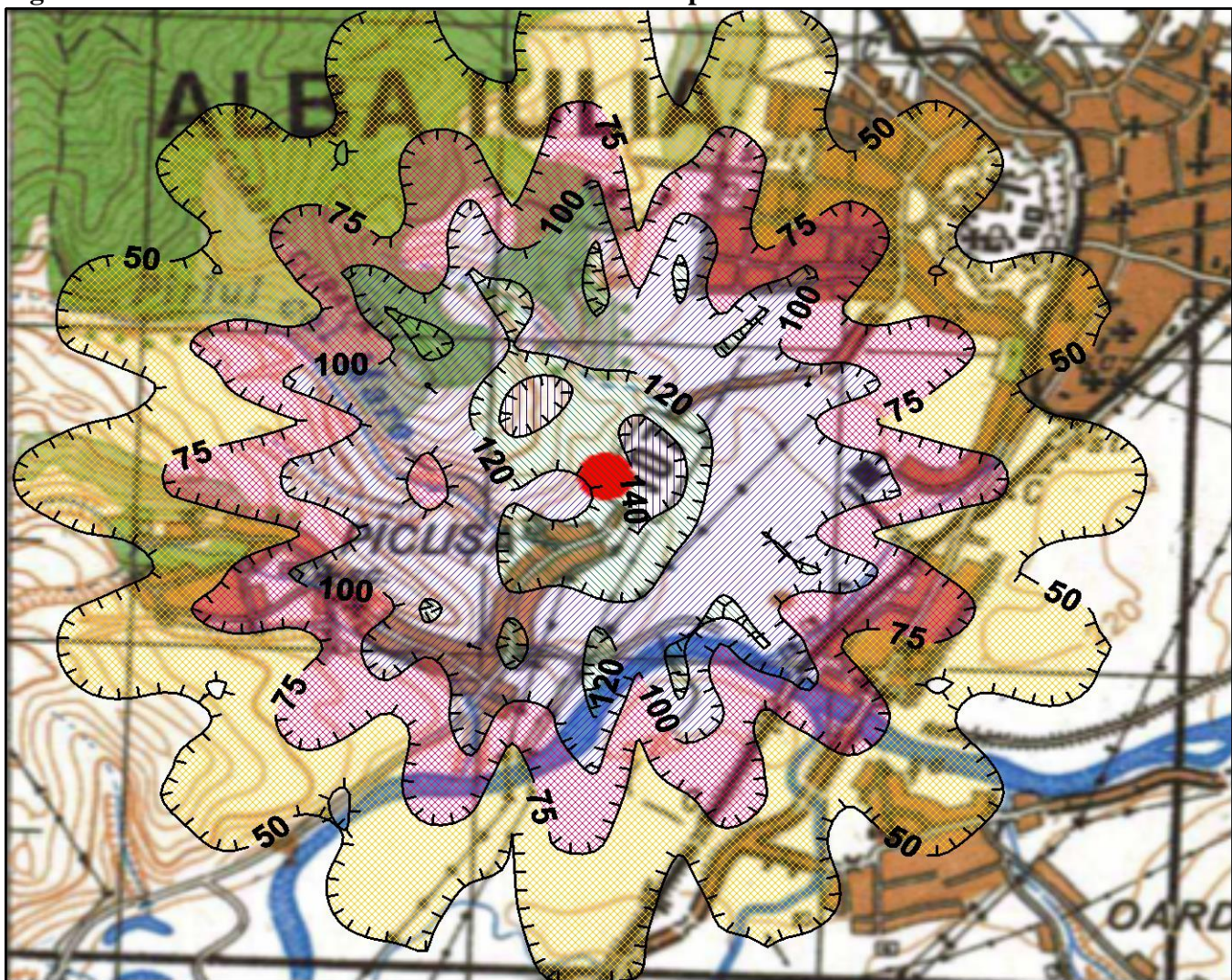
Fig. nr.1. Concentratii maxime de amoniac in aer – timp de mediere 30 minute
