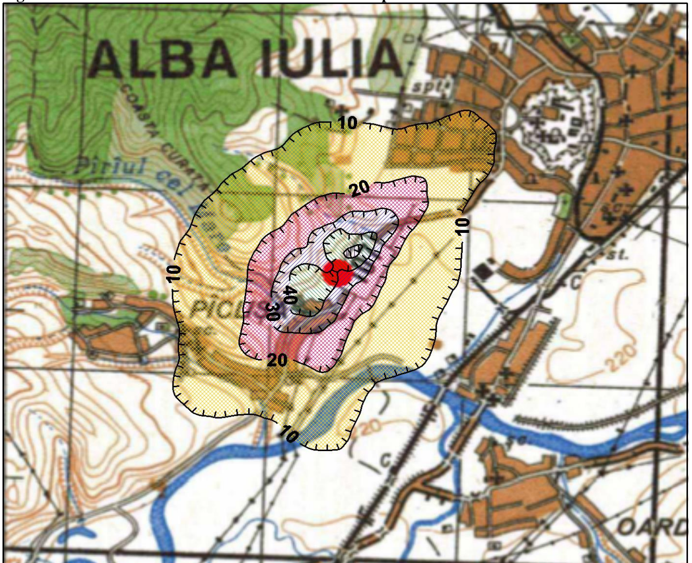
Fig. nr.2. Concentratii maxime de amoniac in aer – timp de mediere 24 ore
