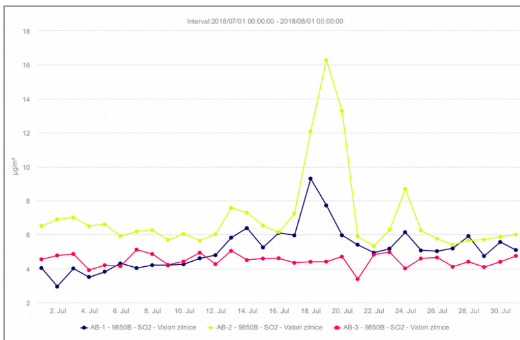
Figura. 1.1.2.2 Dioxid de sulf – media la 24 ore
