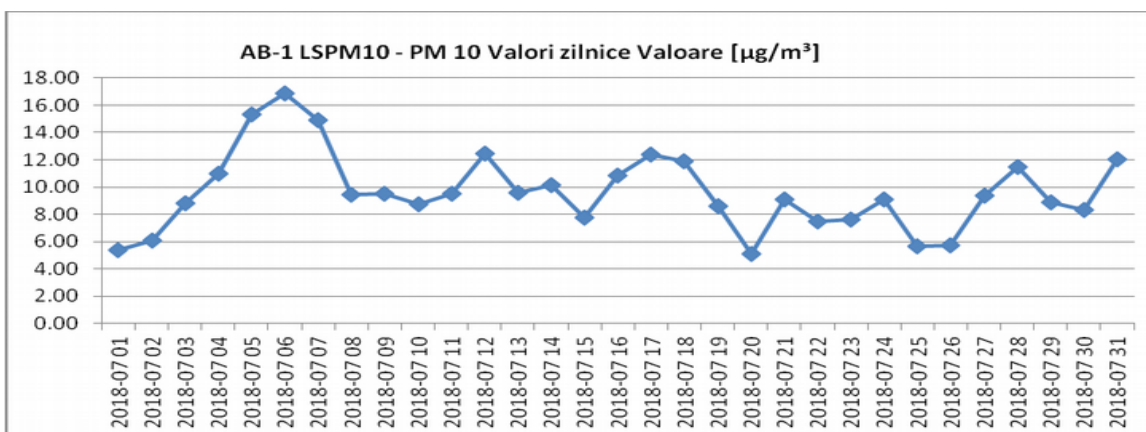
Figura. 1.1.6.1 Pulberi în suspensie \text{PM}_{10} – metoda automată
