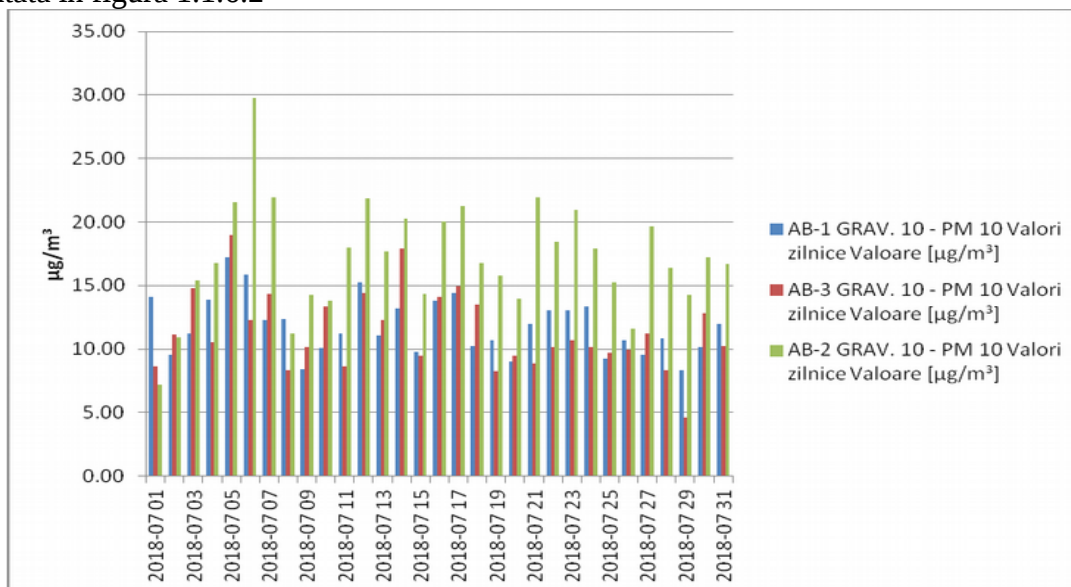
Figura. 1.1.6.2 Pulberi în suspensie \text{PM}_{10} – metoda gravimetrică
