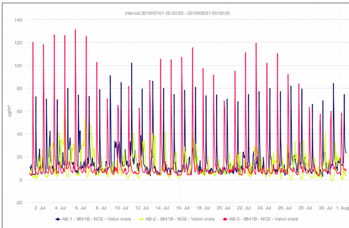
Figura 1.1.1 – Dioxid de azot - valori orare
