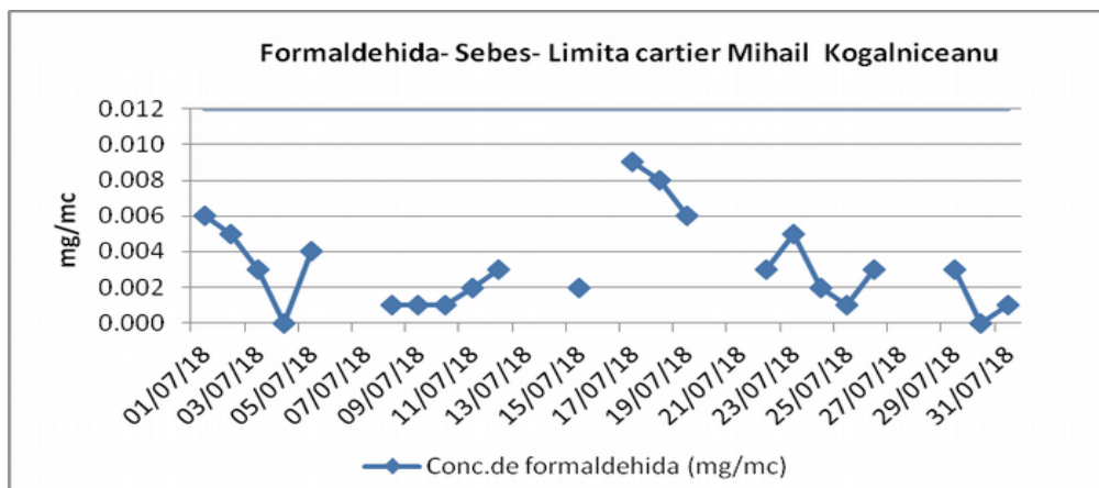
Figura. 1.2.1.2 – Aldehidă formică – Sebeș, Limită Cartier M. Kogălniceanu
