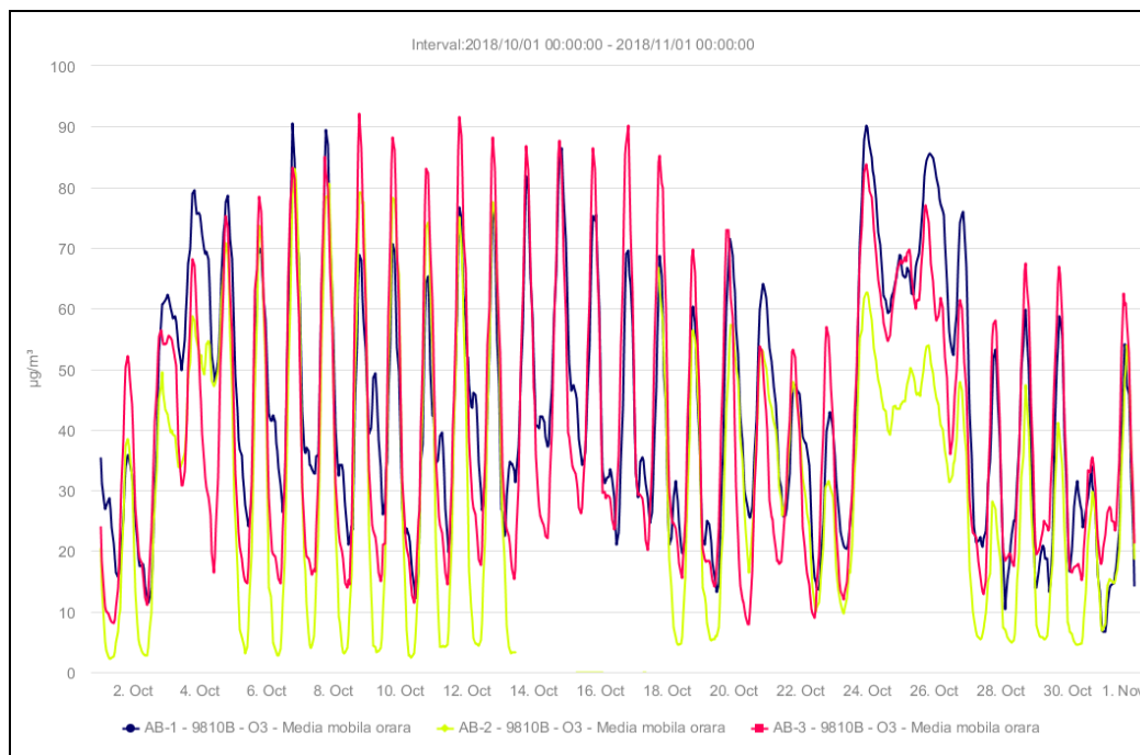
Figura. 1.1.4.2 Ozon – medie mobilă
