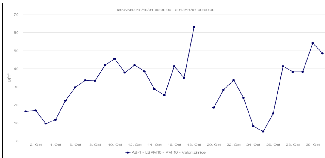
Figura. 1.1.6.1 Pulberi în suspensie PM 10 – metoda automată
