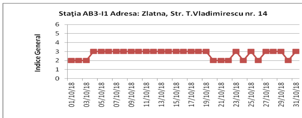
Figura. 1.1.7.4 – Indicele general de calitate a aerului – AB3
