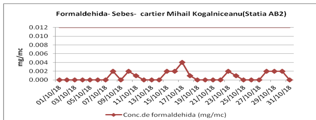
Figura. 1.2.1.1 – Aldehidă formică – Sebeș, stația AB2
