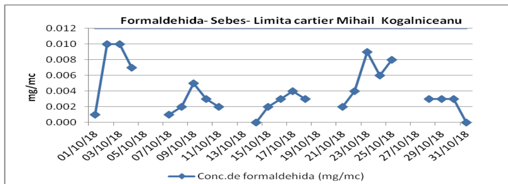
Figura. 1.2.1.2 – Aldehidă formică – Sebeș, Limită Cartier M. Kogălniceanu
