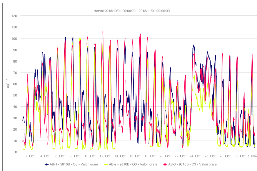
Figura. 1.1.4.1 Ozon – valori orare
