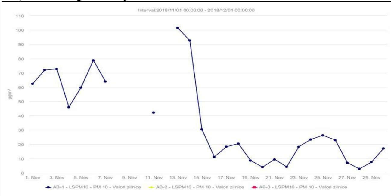
Figura. 1.1.6.1 Pulberi în suspensie PM 10 – metoda automată
