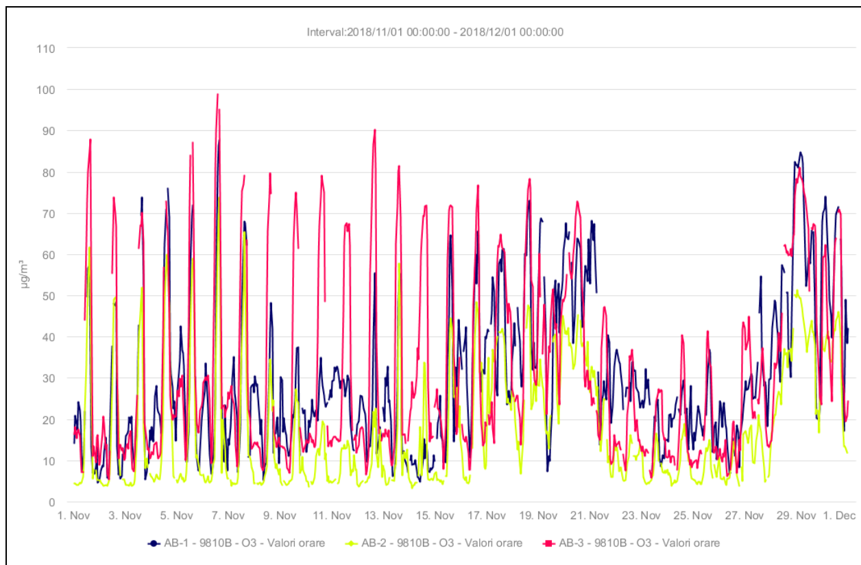
Figura. 1.1.4.1 Ozon – valori orare
