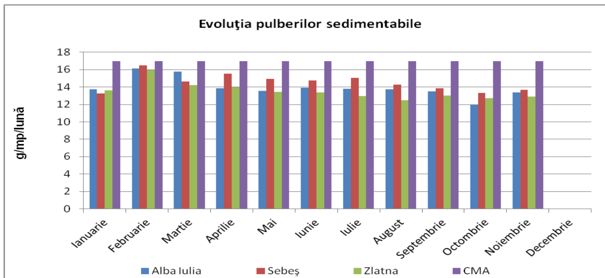
Figura. 1.2.2.2 – Evoluția pulberilor sedimentabile
