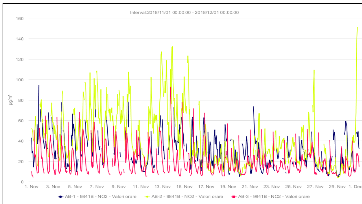
Figura 1.1.1 – Dioxid de azot - valori orare
