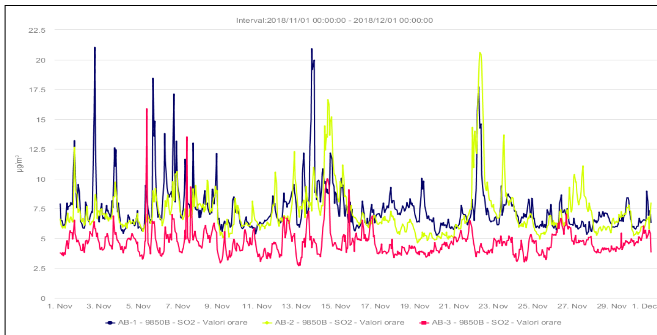
Figura. 1.1.2.1 – Dioxid de sulf – valori orare
