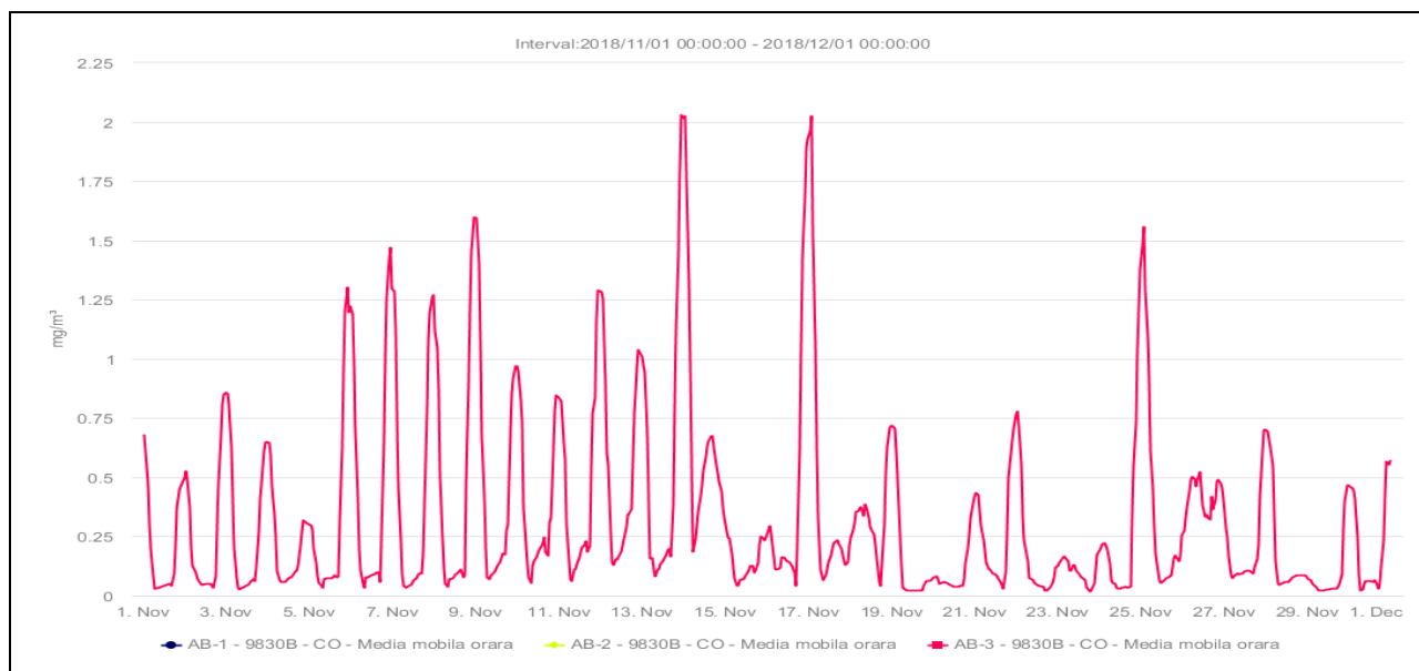
Figura. 1.1.3 – Monoxid de carbon – medie mobilă
