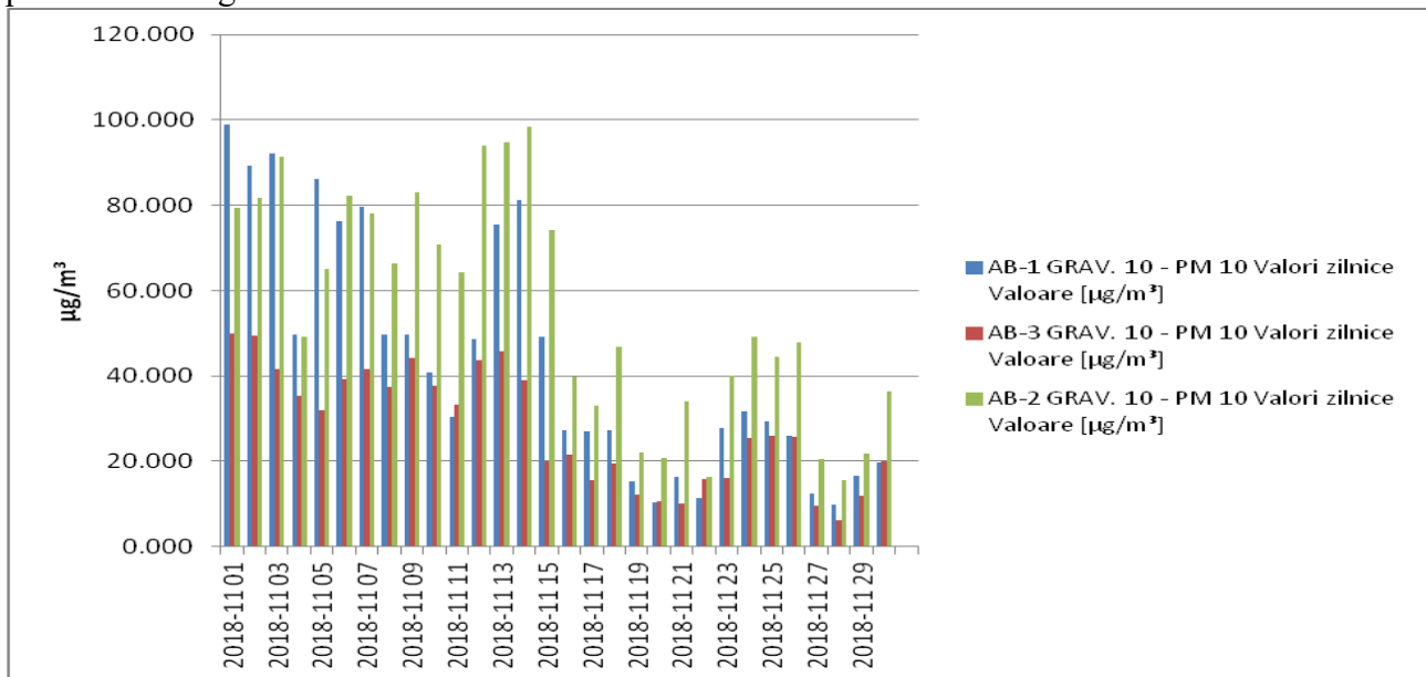
Figura. 1.1.6.2 Pulberi în suspensie PM 10 – metoda gravimetrică
