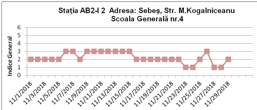
Figura. 1.1.7.2 – Indicele general de calitate a aerului – AB1
