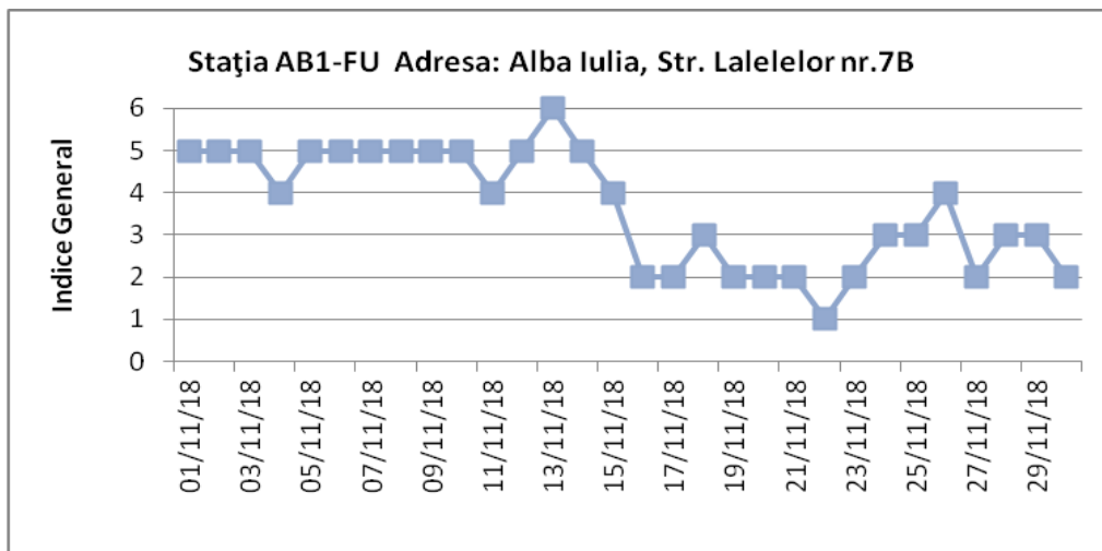
Figura. 1.1.7.3 – Indicele general de calitate a aerului – AB2
