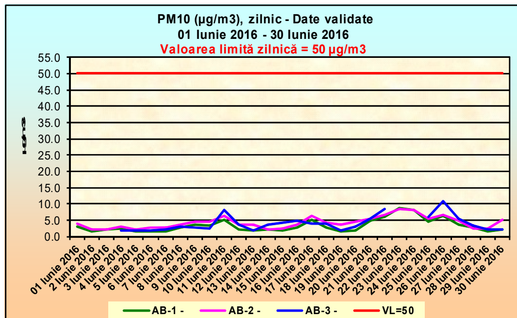
Figura. 1.1.6.1 Pulberi în suspensie PM_{10} – metoda automată
