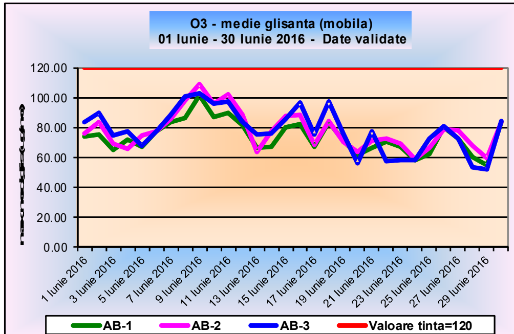
Figura. 1.1.4 Ozon – medie mobila
