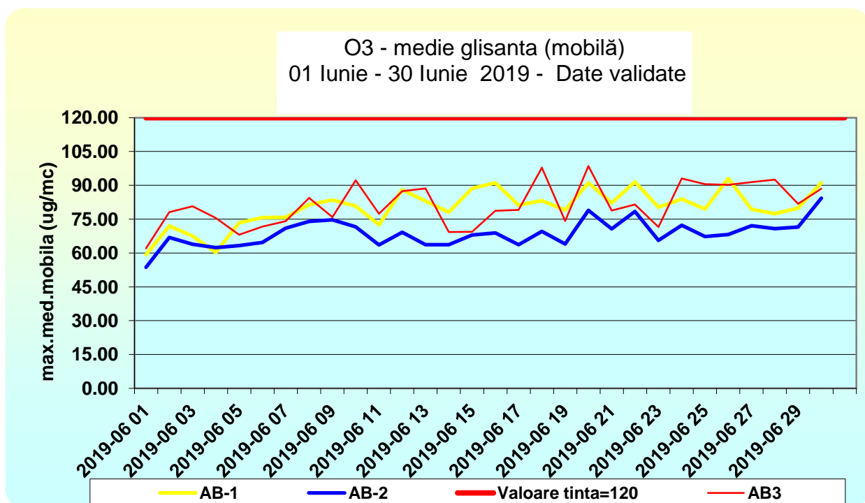
Figura. 1.1.4.2 Ozon – medie mobilă
