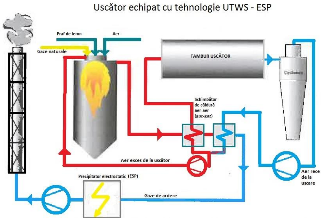
Figura 4 Uscator cu UTWS- ESP
