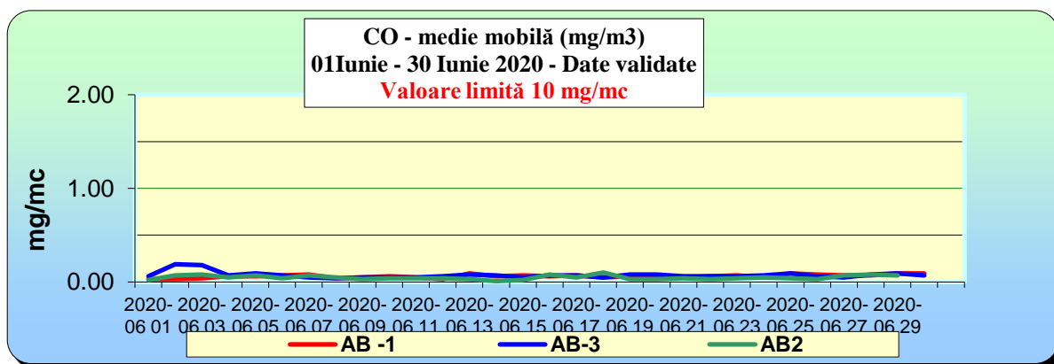
Figura. 1.1.3 – Monoxid de carbon – medie mobilă
