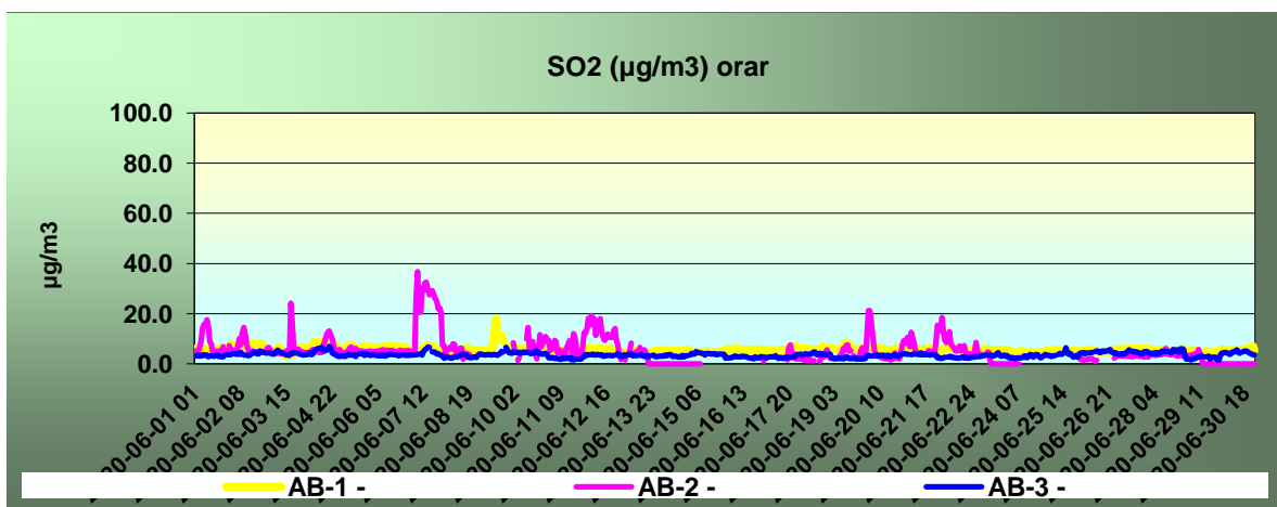
Figura. 1.1.2.1 – Dioxid de sulf – valori orare
