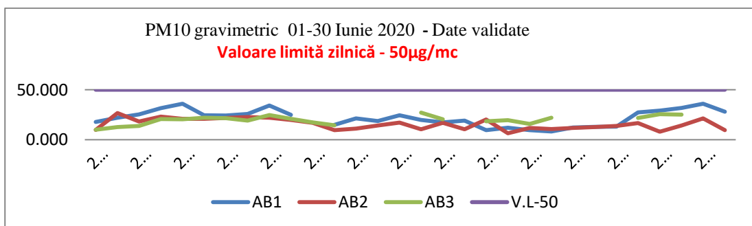
Figura. 1.1.6.2 Pulberi în suspensie PM 10 – metoda gravimetrică
