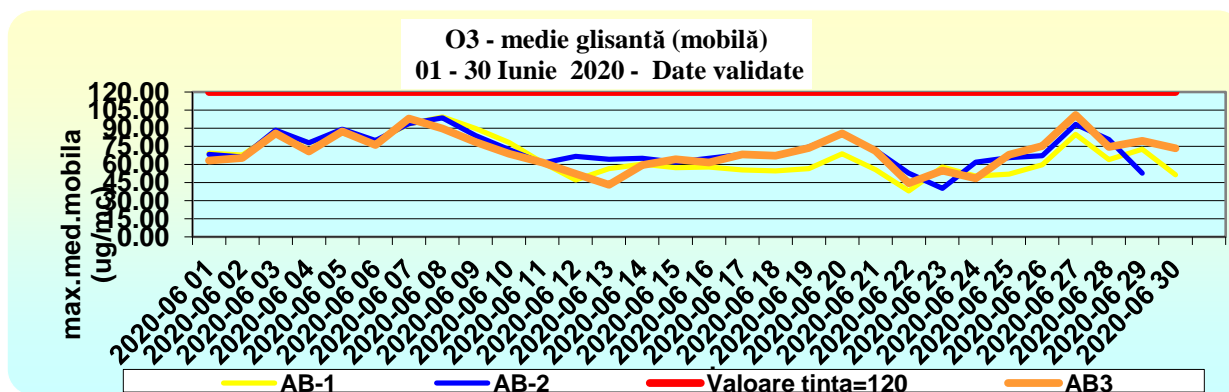
Figura. 1.1.5. Ozon – concentrații maxime zilnice ale mediilor glisante de 8 ore
