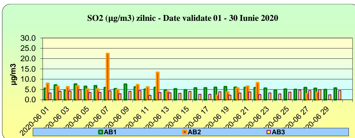
Figura. 1.1.2.2 Dioxid de sulf – media la 24 ore
