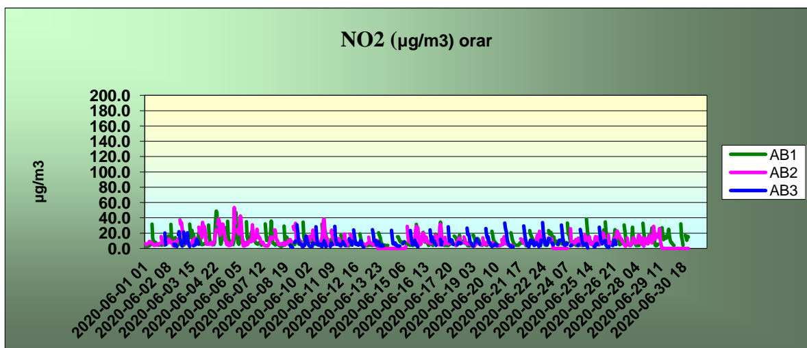
Figura. 1.1.1.1 – Dioxid de azot – valori orare Valoarea limită orară pentru protecția sănătății umane de 200 µg/m 3 nu a fost depășită.
