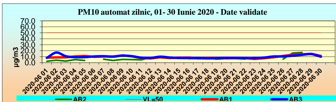
Figura. 1.1.6.1 Pulberi în suspensie PM 10 – metoda automată
