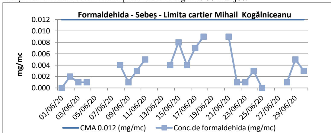
Figura. 1.2.1.1 – Aldehidă formică – Sebeș, Limită Cartier M. Kogălniceanu
