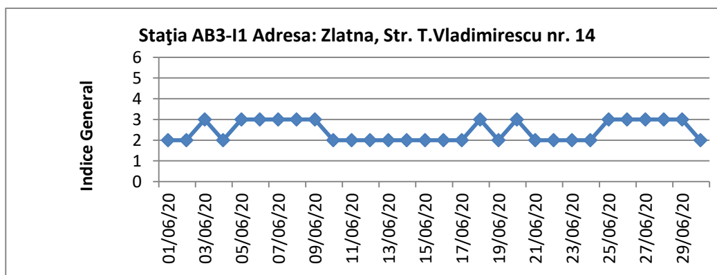
Figura. 1.1.7.4 – Indicele general de calitate a aerului – AB3
