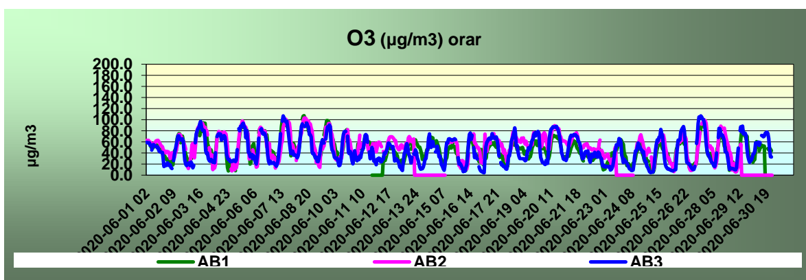
Figura. 1.1.4. Ozon – valori orare
