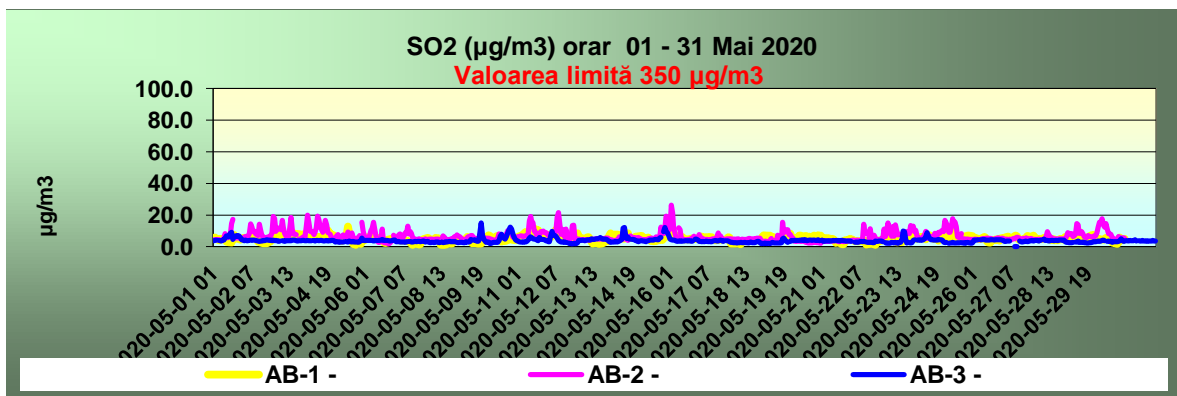
Figura. 1.1.2.1 – Dioxid de sulf – valori orare
