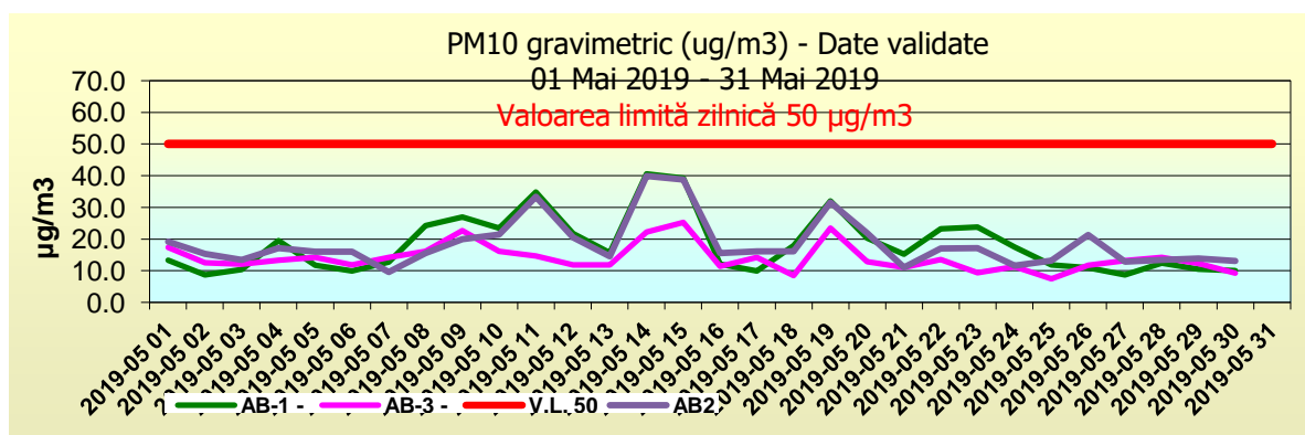
Figura. 1.1.6.2 Pulberi în suspensie \text{PM}_{10} – metoda gravimetrică
