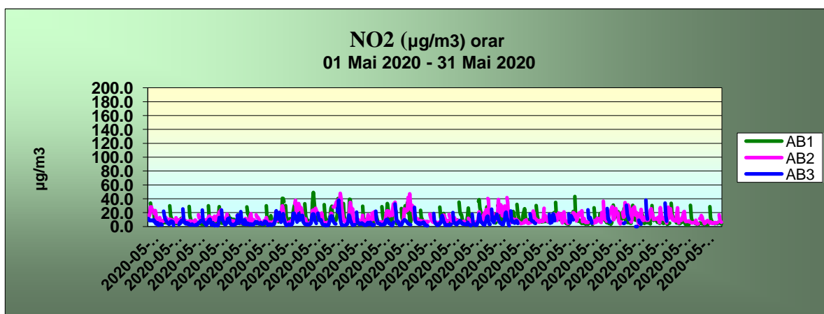
Figura. 1.1.1.1 – Dioxid de azot – valori orare Valoarea limită orară pentru protecția sănătății umane de 200 \mu\text{g}/\text{m}^3 nu a fost depășită.
