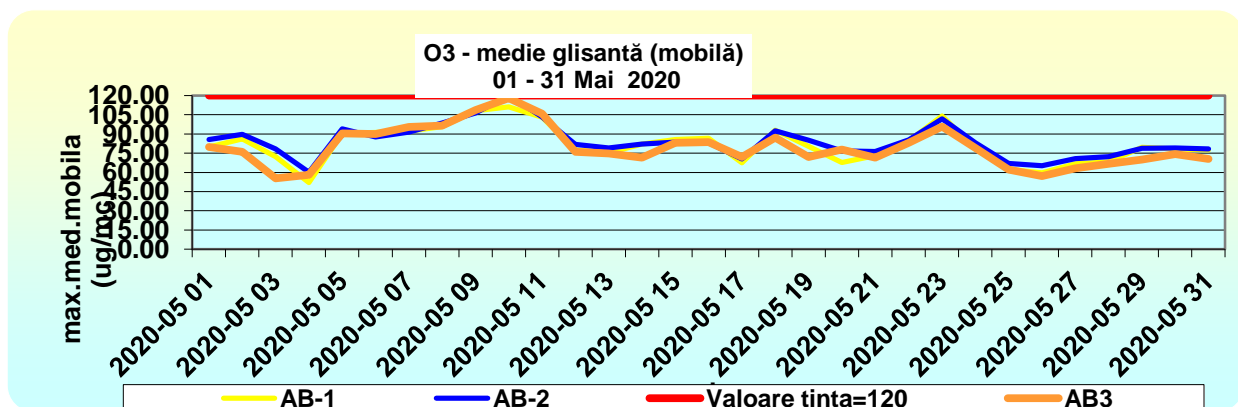
Figura. 1.1.5. Ozon – concentrații maxime zilnice ale mediilor glisante de 8 ore
