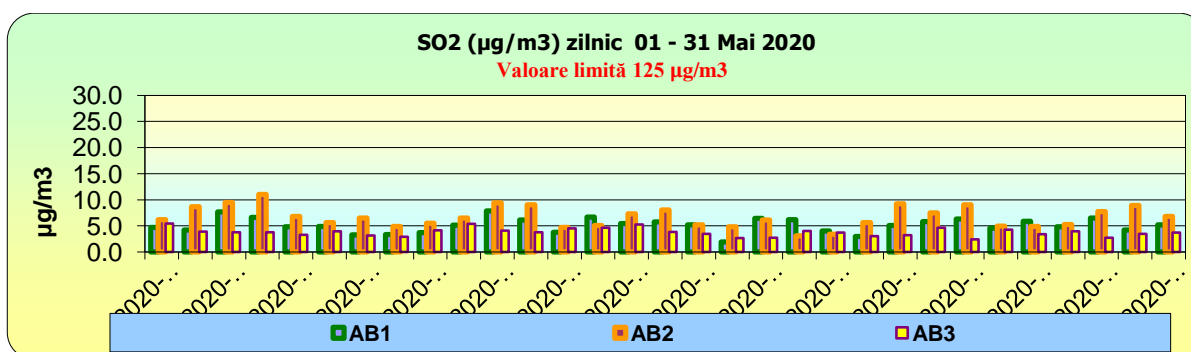
Figura. 1.1.2.2 Dioxid de sulf – media la 24 ore
