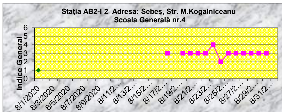
Figura. 1.1.7.3 – Indicele general de calitate a aerului – AB2
