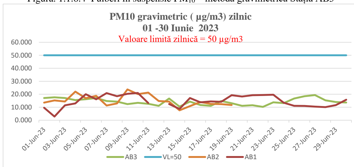
Figura. 1.1.6.2 Pulberi în suspensie \text{PM}_{10} – metoda gravimetrică- comparativ AB1, AB2, AB3
