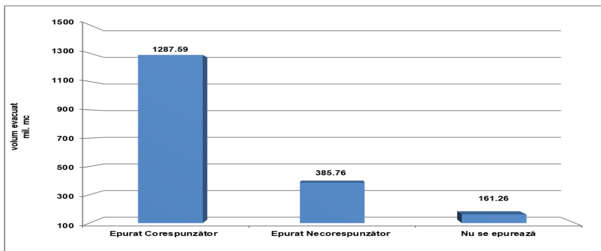
Figura II.2.2.2.1 Volume de ape uzate care necesită epurare, evacuate la nivel național în receptorii naturali în anul 2021 (mii mc.)
