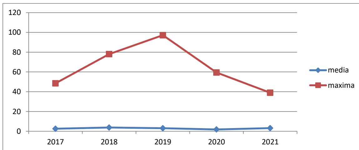
Figura IX.1.1.10 Variația mediilor și maximelor anuale ale activității specifice a depunerilor atmosferice în ultimii 5 ani (Bq·m -2 ·zi -1 ).
