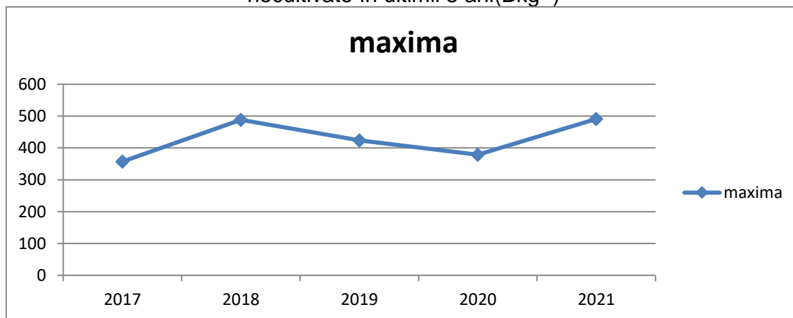
Figura IX.1.4 Variația maximelor anuale ale activității beta globale a vegetației necultivate în ultimii 5 ani ( \text{Bkg}^{-1} )
