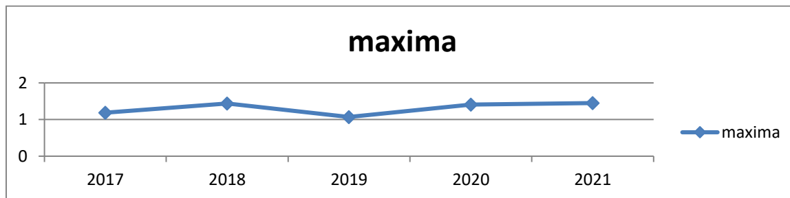
Figura IX.1.2.2 Variația maximelor anuale ale activității beta globale a râului Mureș în ultimii 5 ani (Bql -1 ).
