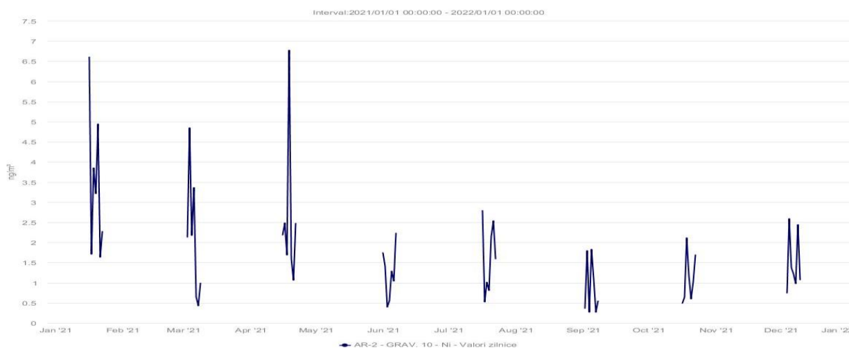
Figura nr. I.1.1.1.3.4. Evoluția valorilor țintă de Ni (ng/mc) din PM 10 gravimetric în anul 2021, la Stația automată de monitorizare AR2
