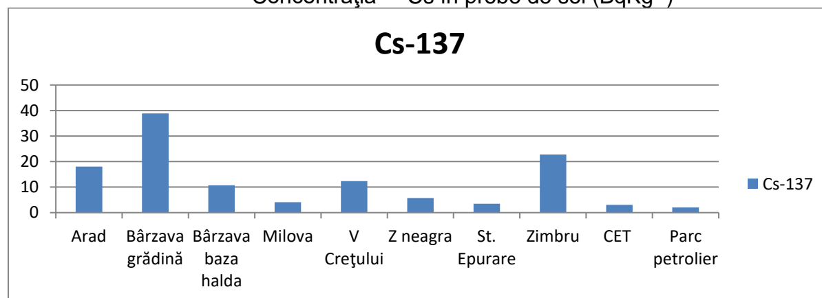
Figura IX.2.1 Concentrația 137 Cs în probe de sol (BqKg -1 )
