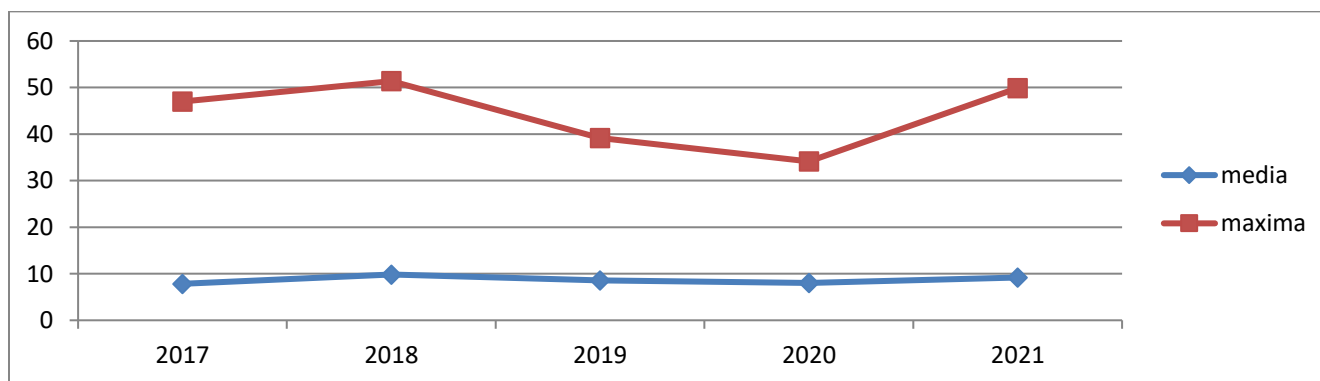
Figura IX.1.1.6 Variația mediilor și maximelor anuale ale activității specifice a radonului din atmosferă în ultimii 5 ani(Bqm -3 ).
