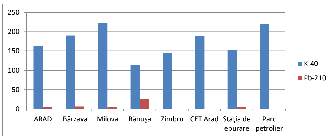
Figura IX.2.2 Concentrația ^{210}\text{Pb} și ^{40}\text{K} în probele de vegetație recoltate în județul Arad ( \text{Bq.Kg}^{-1} ).
