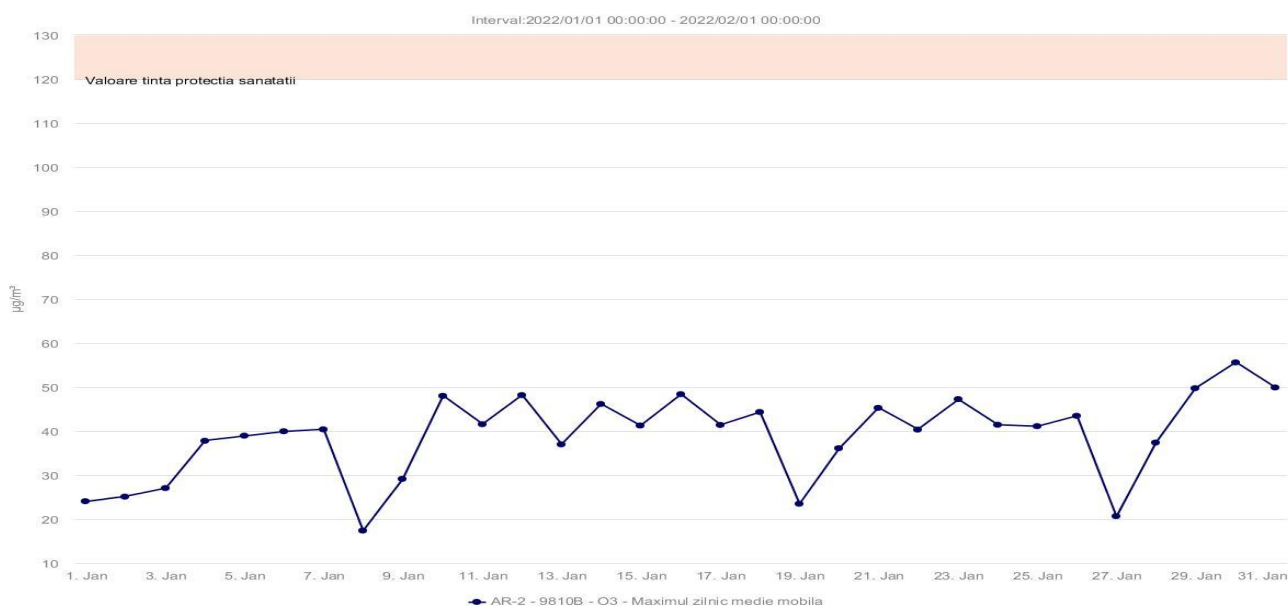
Fig. 1.2.4.2. Concentrațiile mediilor zilnice ale poluantului \text{O}_3
