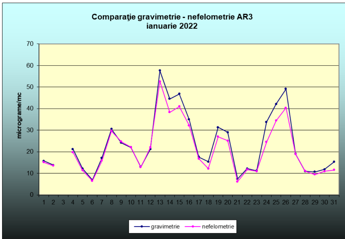
În fig.1.2.5.3. se prezintă grafic, evoluția măsurătorilor gravimetrice față de măsurătorile nefelometrice ale PM10, la Stația de monitorizare AR3.
