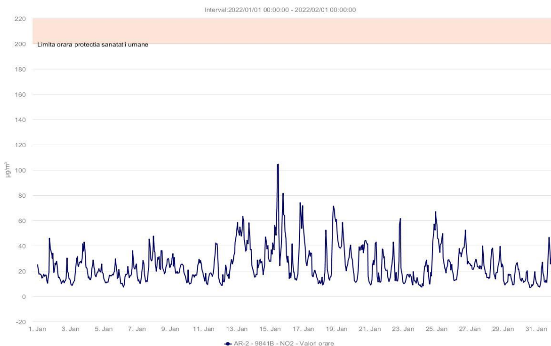
Fig.1.2.2.2. Concentrațiile medii orare ale poluantului \text{NO}_2
