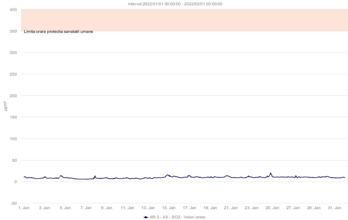
Fig. 1.2.1.6. Concentrațiile medii zilnice ale poluantului SO 2
