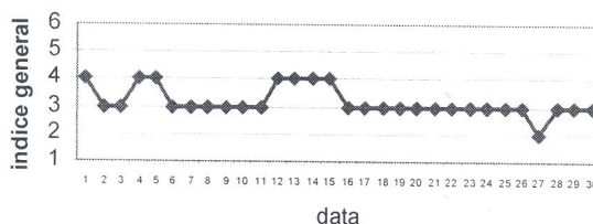
Evoluția indicelui general de calitate a aerului stația BC 3 - aprilie 2018
