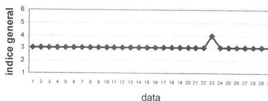
Evoluția indicelui general de calitate a aerului stația BC 2 - aprilie 2018
