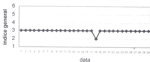
Evoluția indicelui general de calitate a aerului stația BC 1 - aprilie 2018
