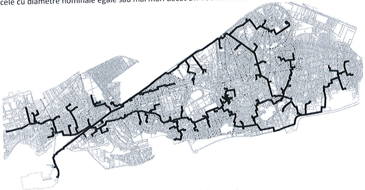
Configurație rețea termică primară
