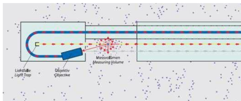
Principiu de masura analizor de pulberi D-R800
