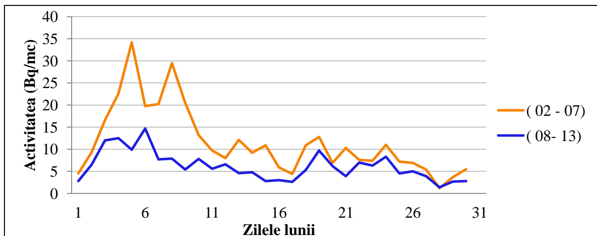
Fig.4.1.1.1. Activitatea specifică beta globală aerosolilor atmosferici
