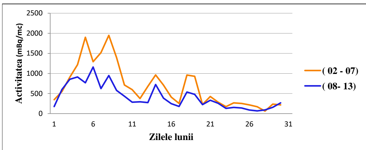
Fig.4.1.2.2. Activitatea specifică beta globală a Toronului
