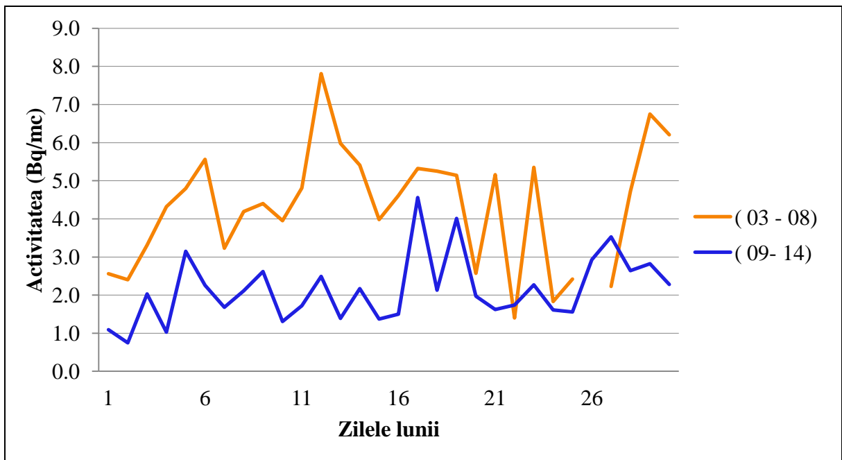
Fig.4.1.1.1. Activitatea specifică beta globală aerosolilor atmosferici
