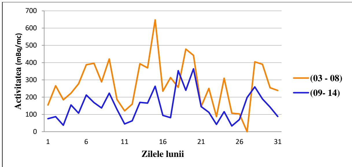
Fig.4.1.2.2. Activitatea specifică beta globală a Toronului
