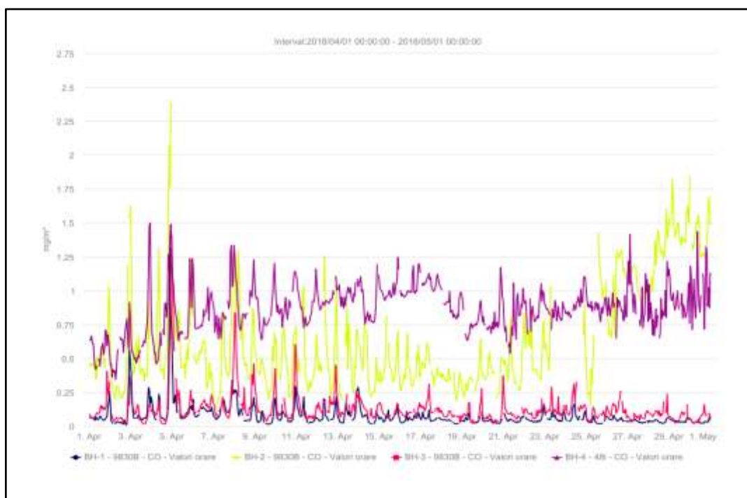
Fig.6. Concentrații CO
