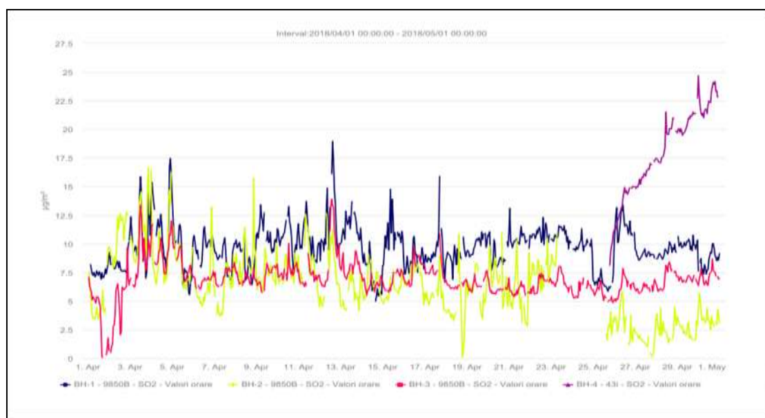
Fig.4. Concentrații SO 2
