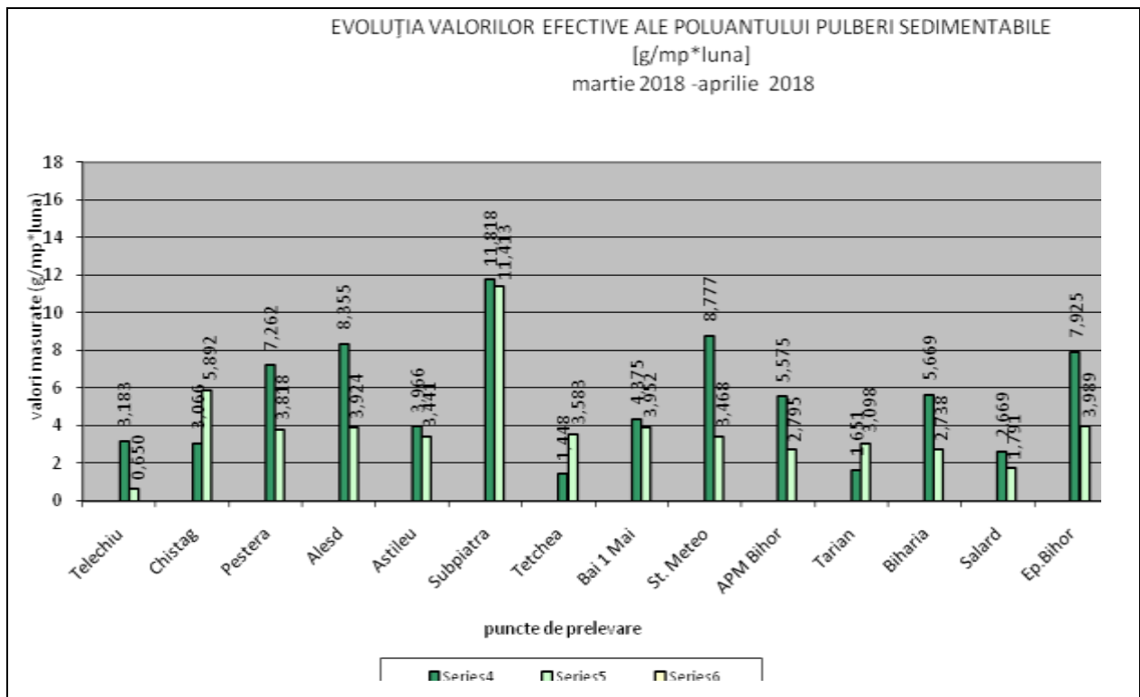
Fig.1. Pulberi sedimentabile
