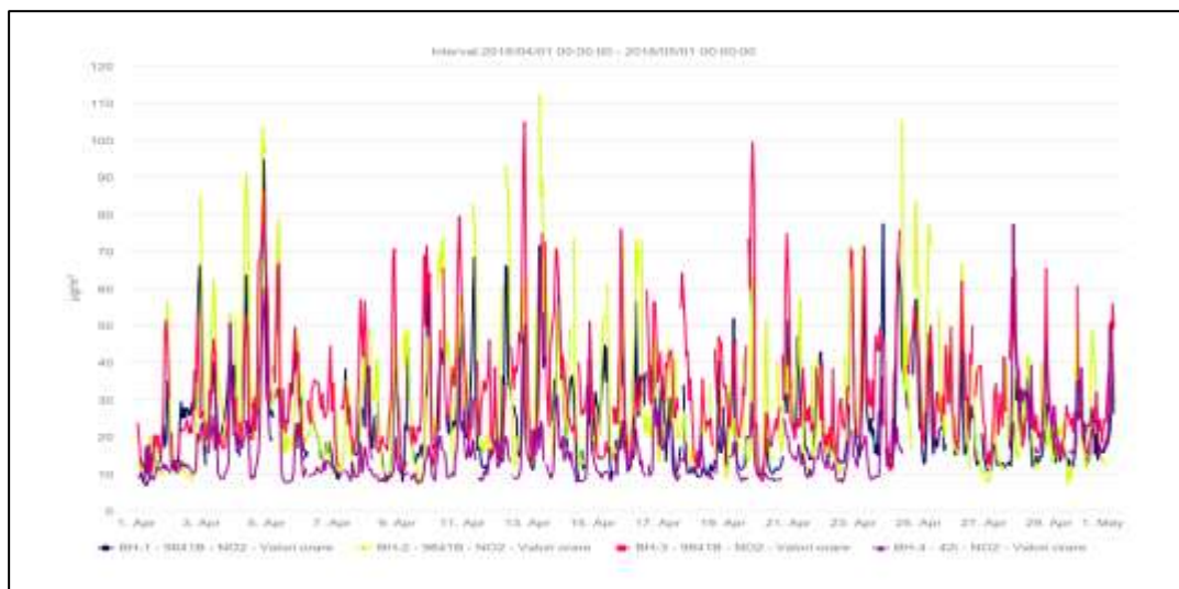
Fig.5. Concentrații NO 2
