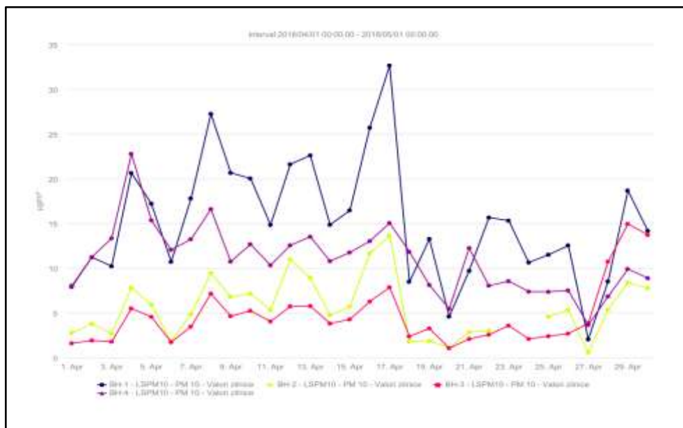
Fig.7. Concentrații PM_{10}
