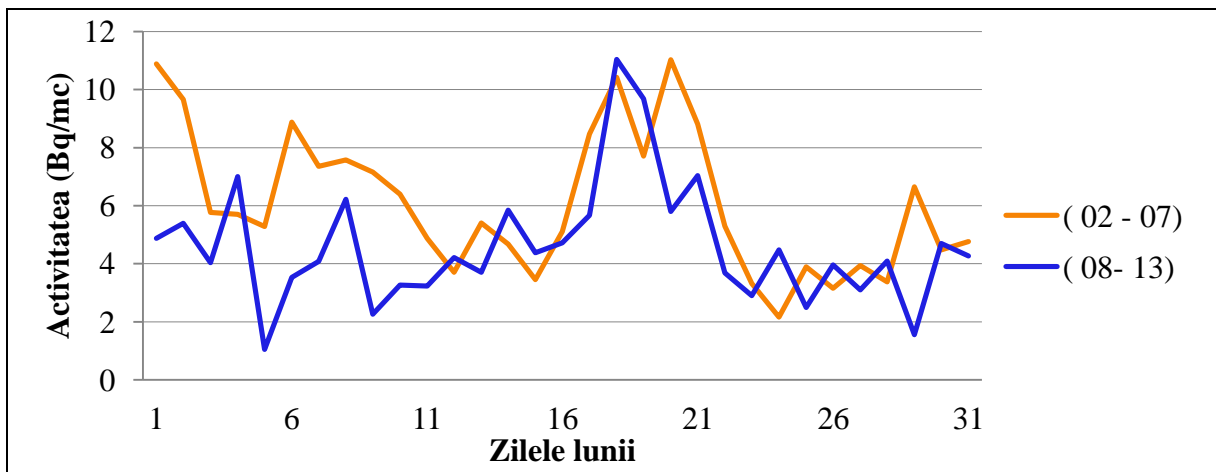
Fig.4.1.1.1. Activitatea specifică beta globală aerosolilor atmosferici
