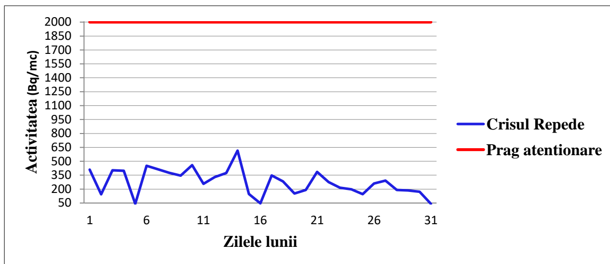
Fig.4.1.4.1. Activitatea specifică beta globală a apei – Crișul Repede
