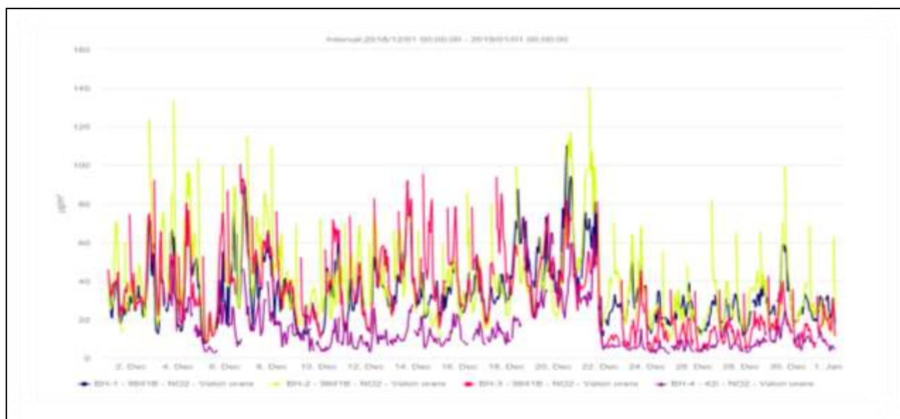
Fig.2.2.4. Concentrații NO_2
