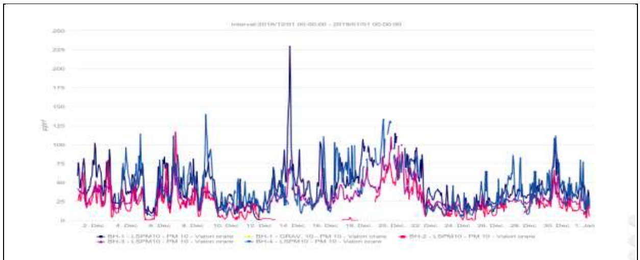
Fig.2.2.6. Concentrații PM 10
