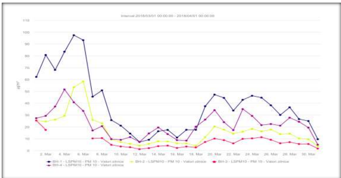
Fig.7. Concentrații PM 10
