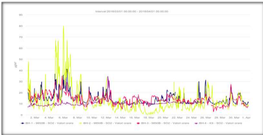
Fig.4. Concentrații SO_2
