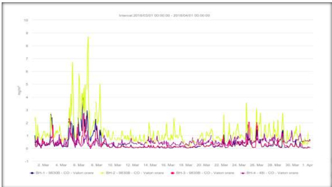
Fig.6. Concentrații CO
