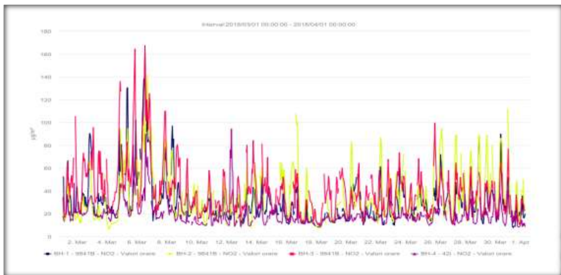
Fig.5. Concentrații NO_2
