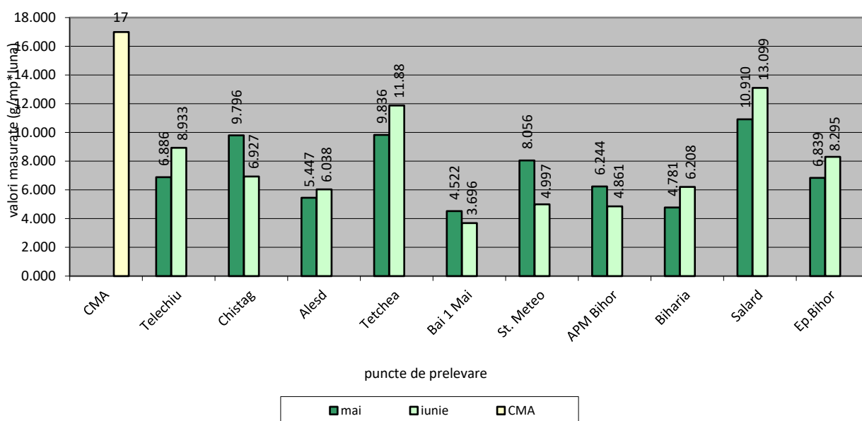
EVOLUȚIA VALORILOR EFECTIVE ALE POLUANTULUI PULBERI SEDIMENTABILE [g/mp*lună] pentru luna iunie 2023
