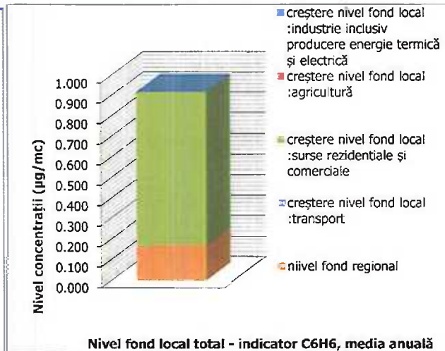
Figura nr. III-96 Fond local total – indicator C6H6
