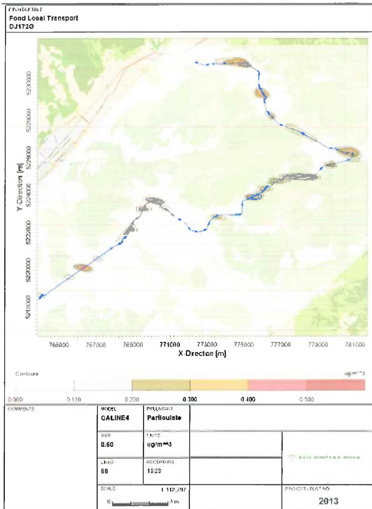
Figura nr. III-84 Creșterea nivel Fond local Transport DJ172G – PM10
