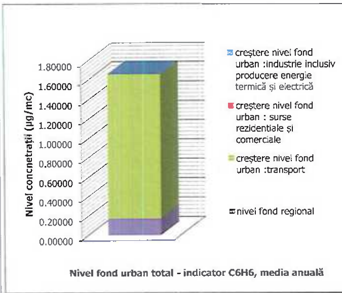
Figura nr. III-37 Nivel Fond urban total – indicator C6H6
