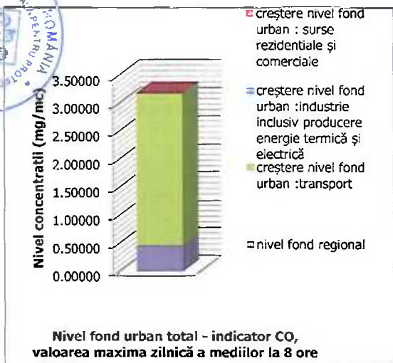
Figura nr. III-30 Nivel fond urban total – indicator CO
