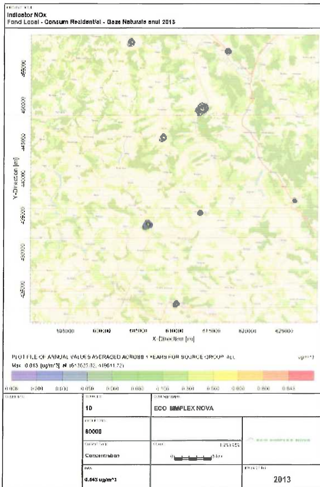
Figura nr. III-51 Creșterea nivel Fond local-Consum Rezidential GN NO2
