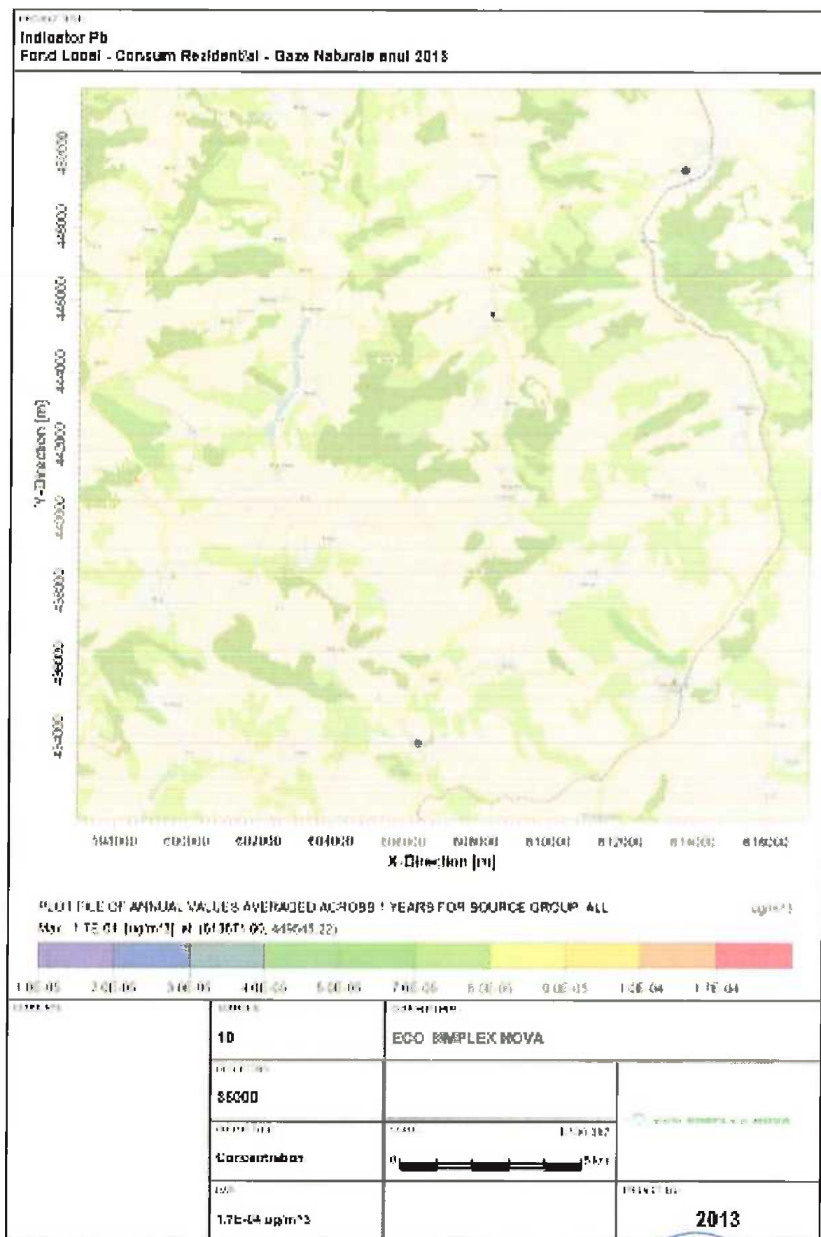
Figura nr. III-55 Creştere nivel Fond local – Consum Rezidential GN – Pb
