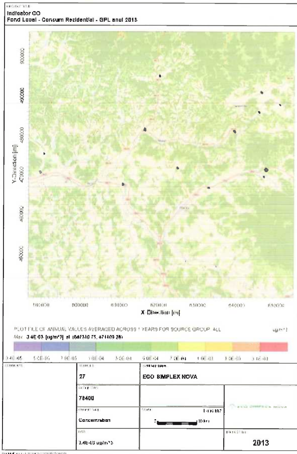
Figura nr. III-60 Creștere nivel Fond local – Consum Rezidențial GPL – CO
