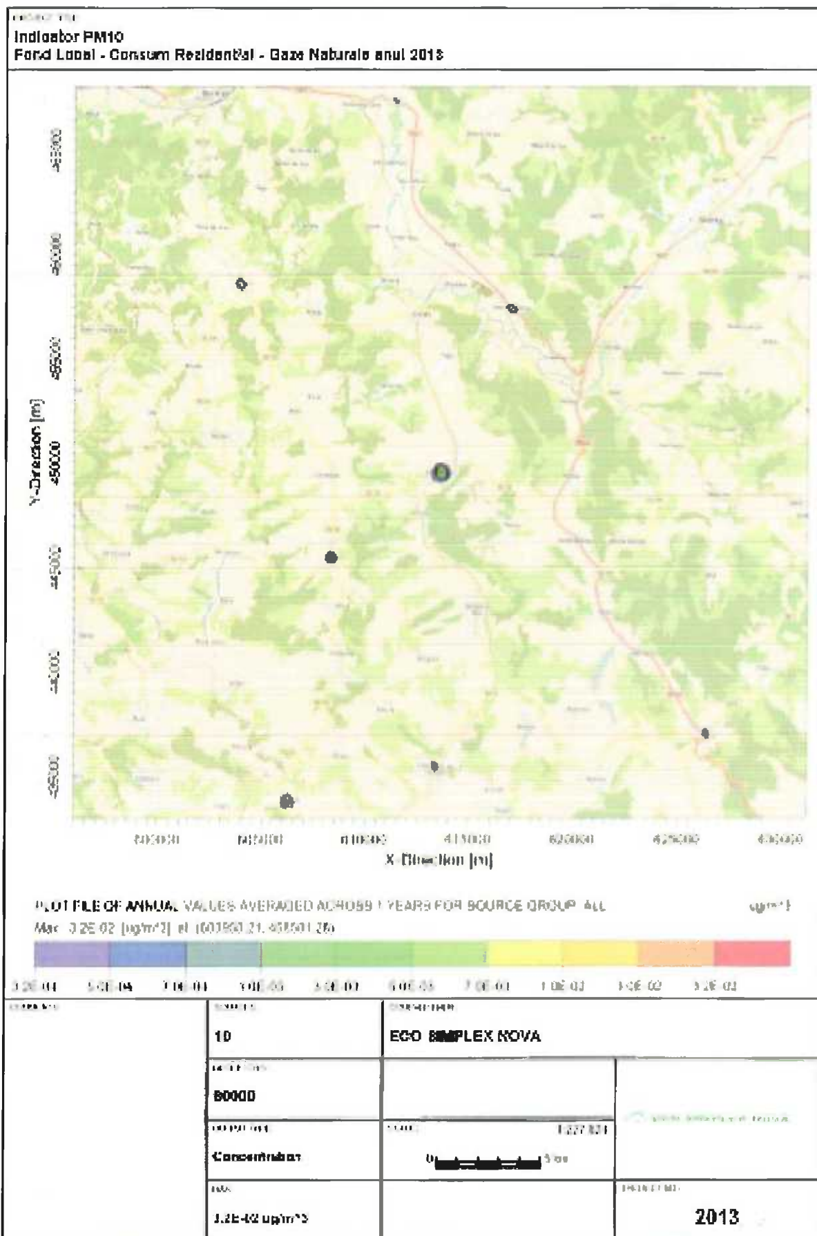
Figura nr. III-53 Creștere nivel Fond local – Consum Rezidențial GN 3 PM10
