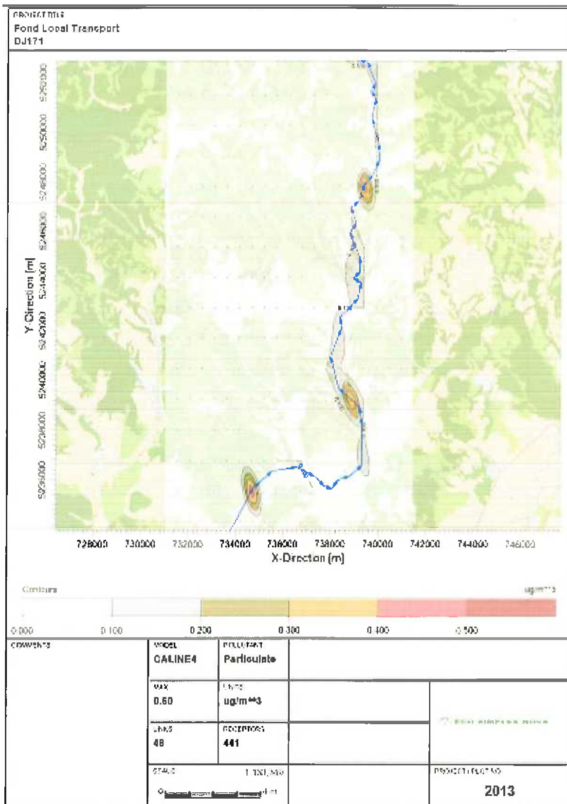
Figura nr. III-82 Creșterea nivel Fond local Transport DJ171 – PM10
