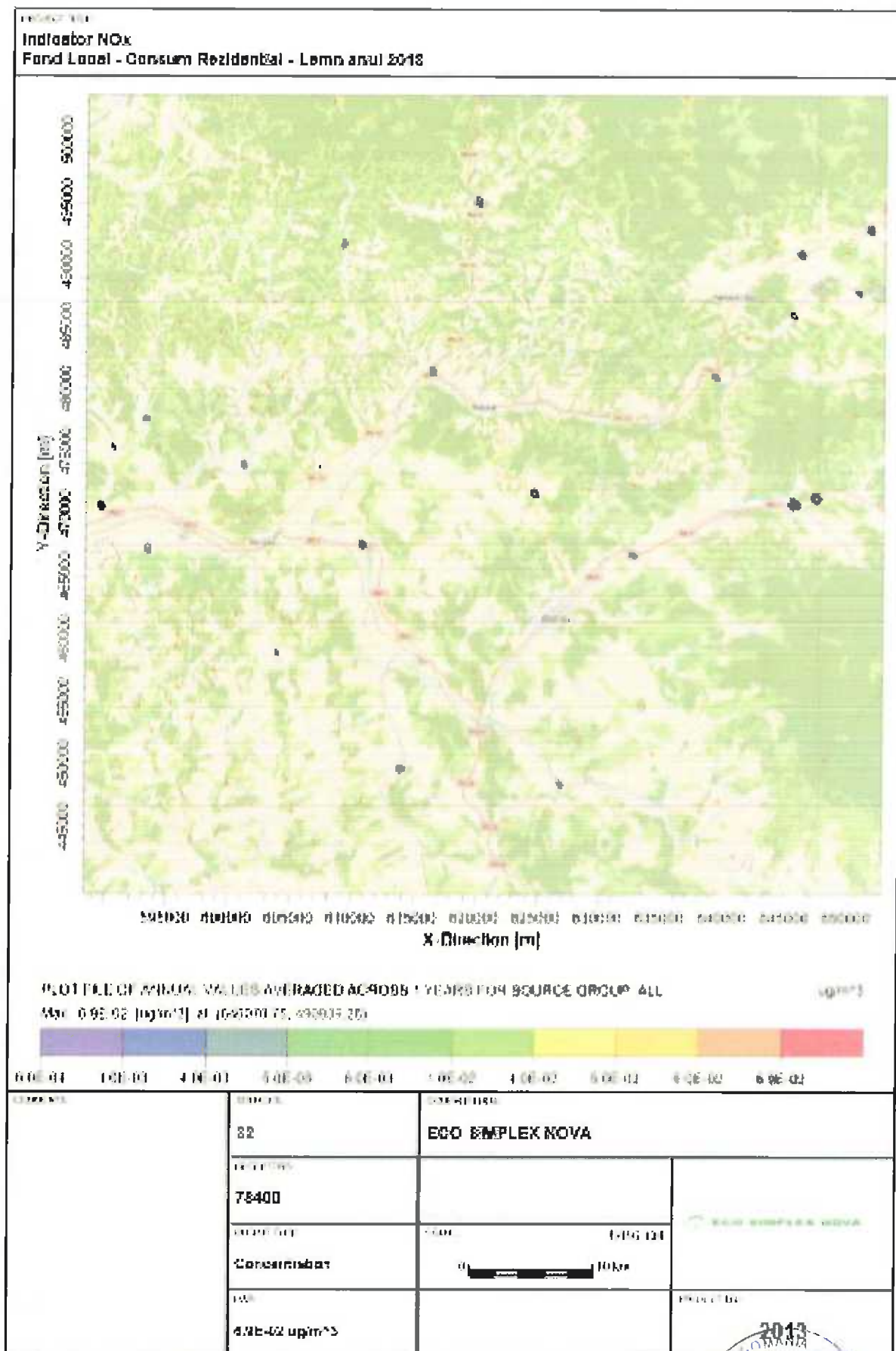
Figura nr. III-63 Creștere nivel Fond local – Consum Rezidențial Lemn – NO 2
