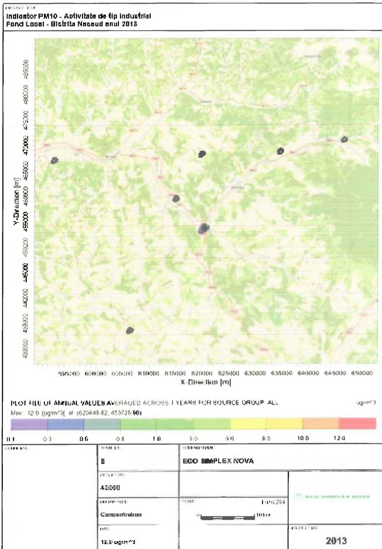
Figura nr. III-41 Creșterea nivelului Fond local – Industrie – Indicator PM10
