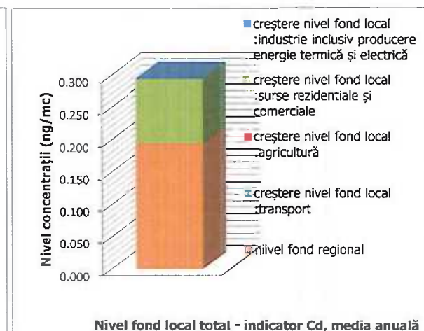
Figura nr. III-93Fond local total – indicator Cd
