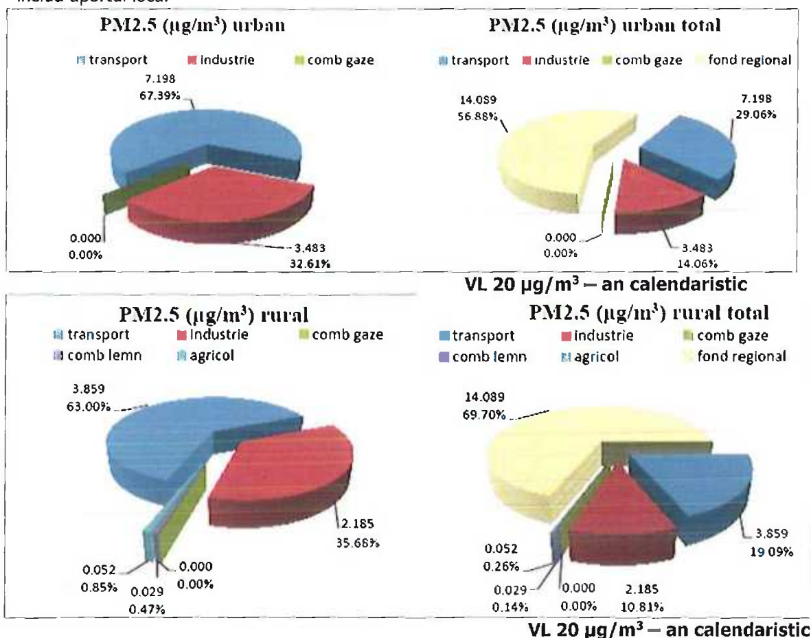
Figura nr. IV-4 Nivelul PM 2,5 în anul de proiecție, fără aplicarea măsurilor PMCA -valori maxime* ale concentrațiilor medii nuale
