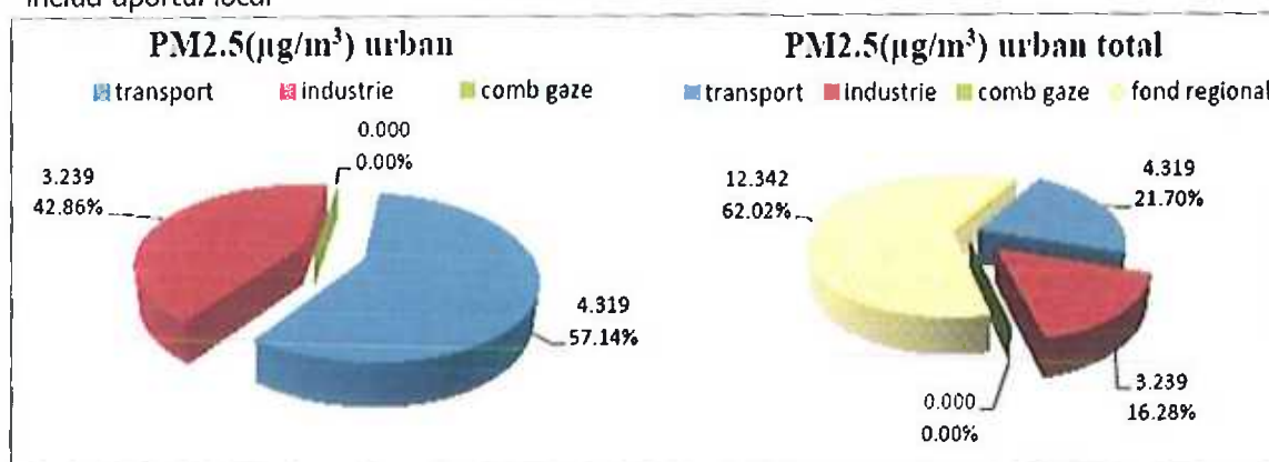
Figura nr. IV-5 Nivelul PM2,5 în anul de proiecție, cu aplicarea măsurilor PMCA - valori maxime* ale concentrațiilor medii anuale
