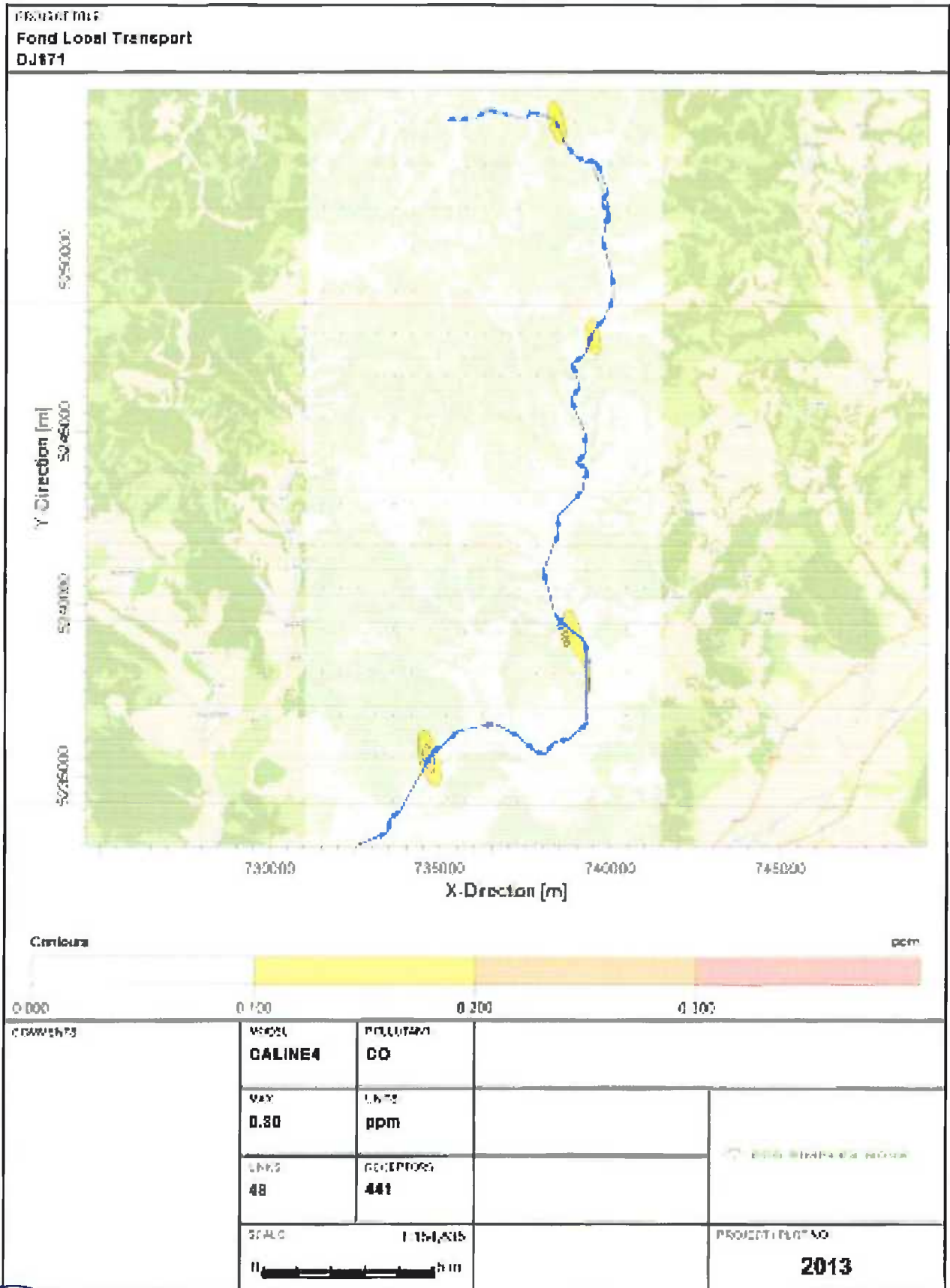
Figura nr. III-76 Creștere nivel Fond local Transport DJ171 - CO
