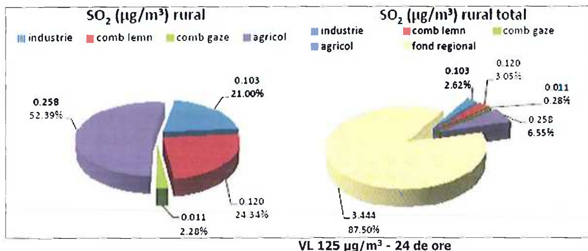
Figura nr,IV-11 Nivelul SO 2 în anul de proiecție, cu aplicarea măsurilor PMCA –valori maxime* concentrații la 24 de ore *inclus aportul local
