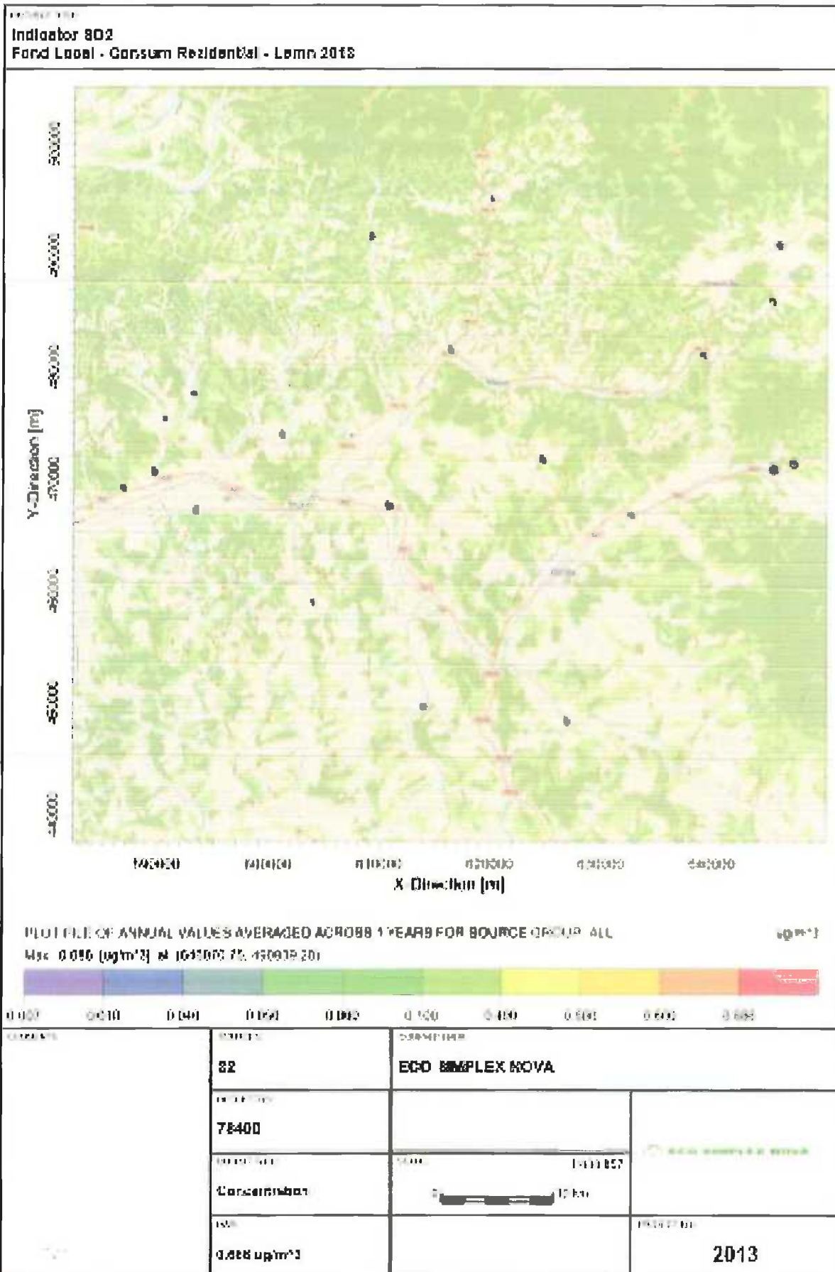
Figura nr. III-62 Creșterea nivelului Fond local – Consum rezidențial Lemn – SO2
