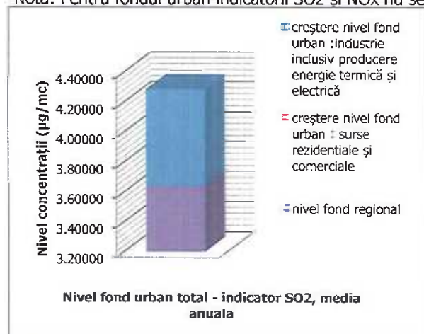
Figura nr. III-27 Nivel Fond urban total – indicator SO 2
