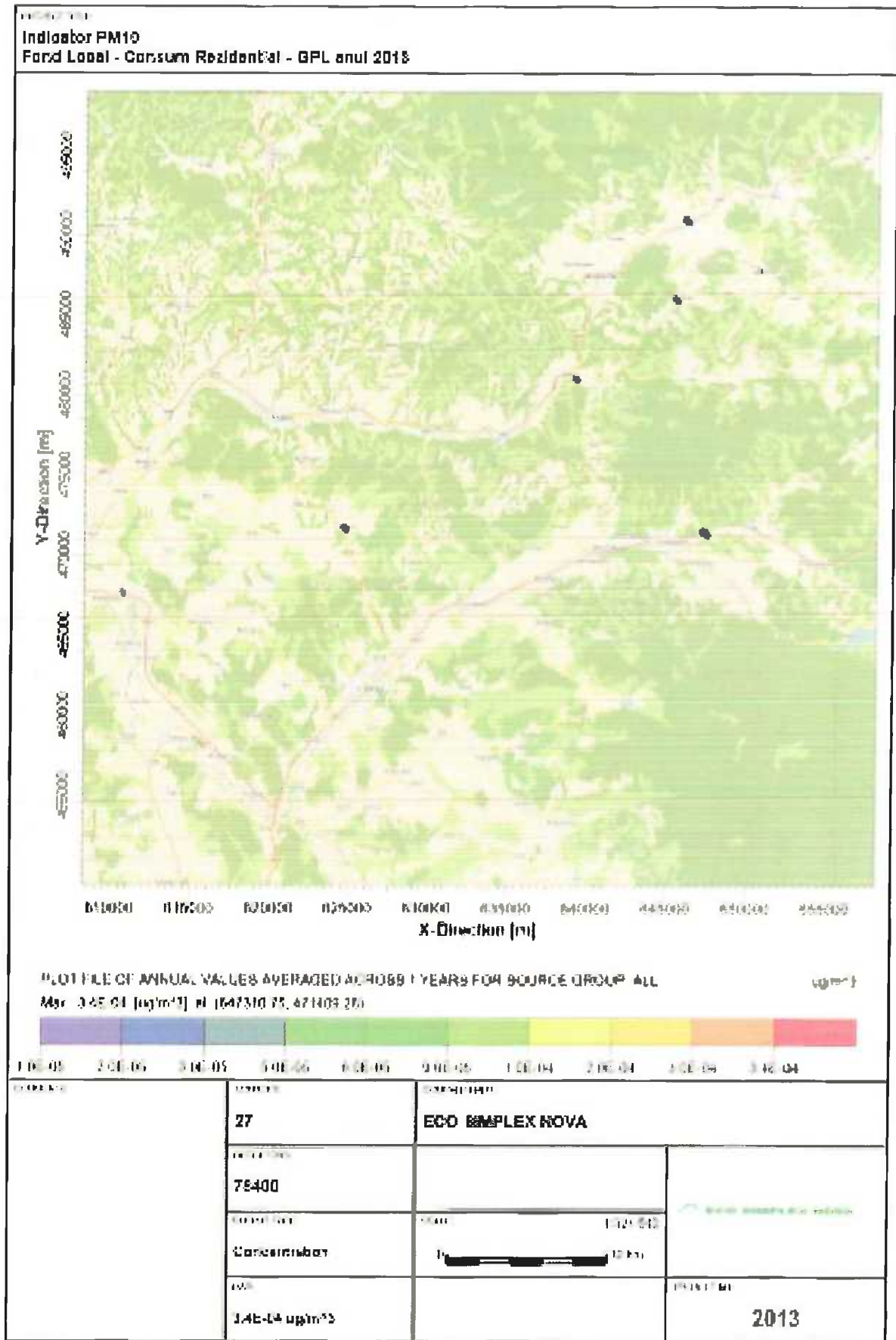
Figura nr. III-61 Creșterea nivelului fondului local – Consum rezidențial GPL
