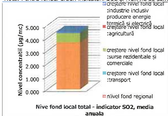
Figura nr. III-86Fond local total – indicator SO2
