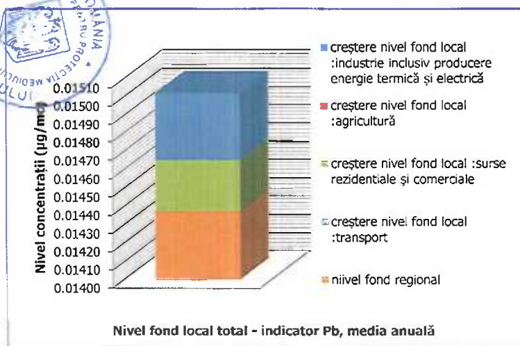
Figura nr. III-95Fond local total – indicator Pb
