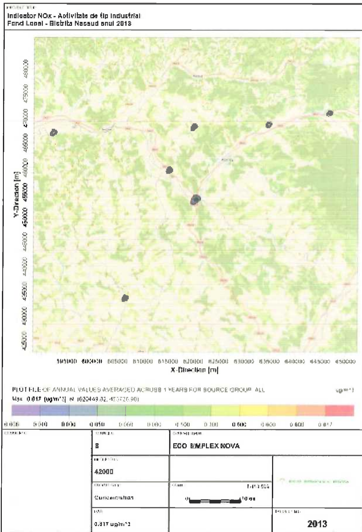
Figura nr. III-39 Creştere nivel Fond local – Industrie – Indicator NOx
