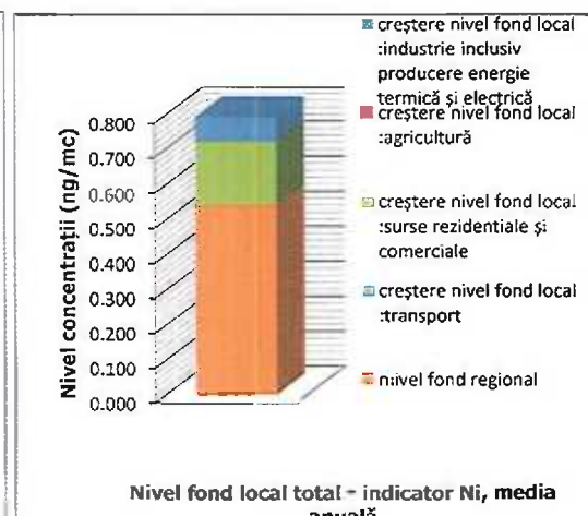
Figura nr. III-94Fond local total – indicator Ni
