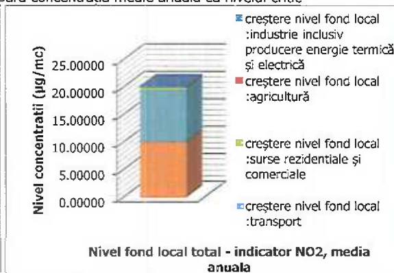
Figura nr. III-87Fond local total – indicator NO2
