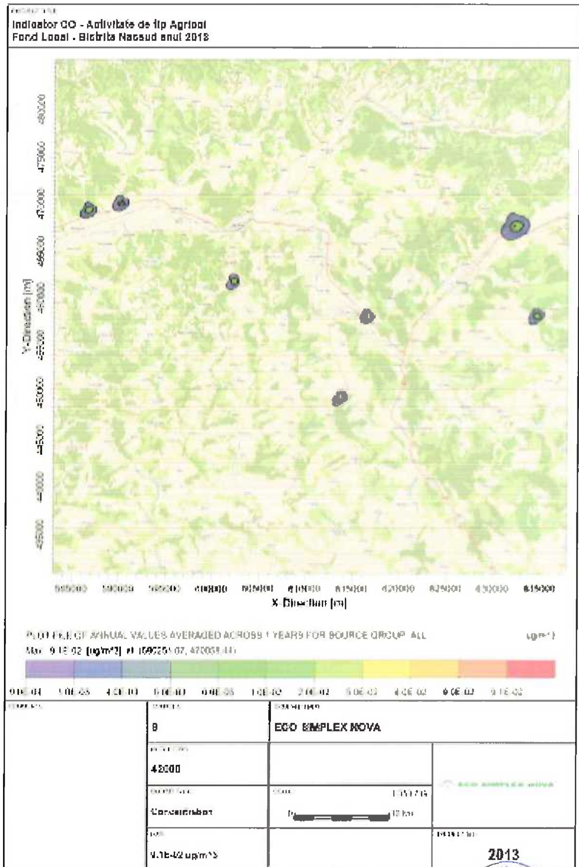
Figura nr. III-47 Creșterea nivelului Fond local – Agricultură – Indicator CO
