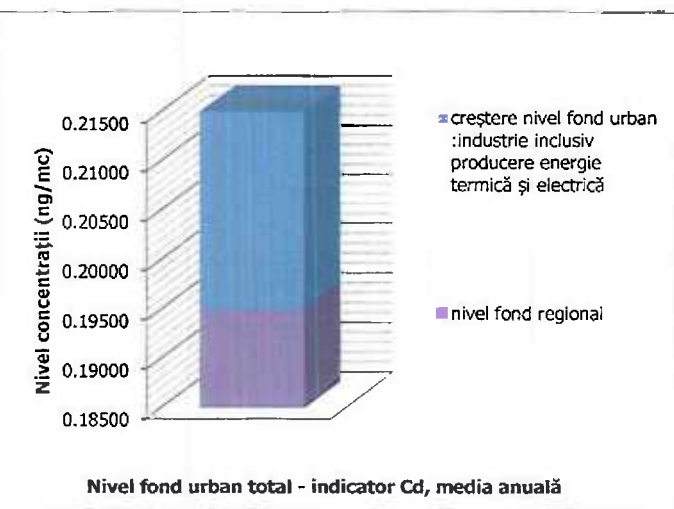
Figura nr. III-34 Nivel Fond urban total – indicator Cd
