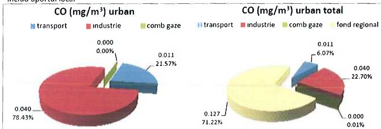
Figura nr. IV-9 Nivelul CO în anul de proiecție, cu aplicarea măsurilor PMCA – valori maxime* zilnice ale mediei mobile
