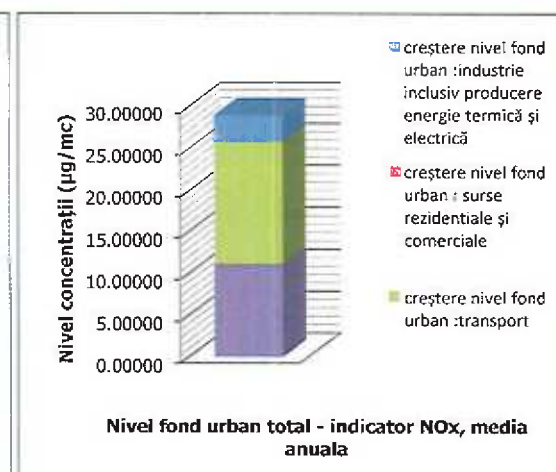
Figura nr. III-29 Nivel Fond urban total – indicator NOx
