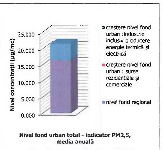
Figura nr. III-32Nivel Fond urban total – indicator PM2,5
