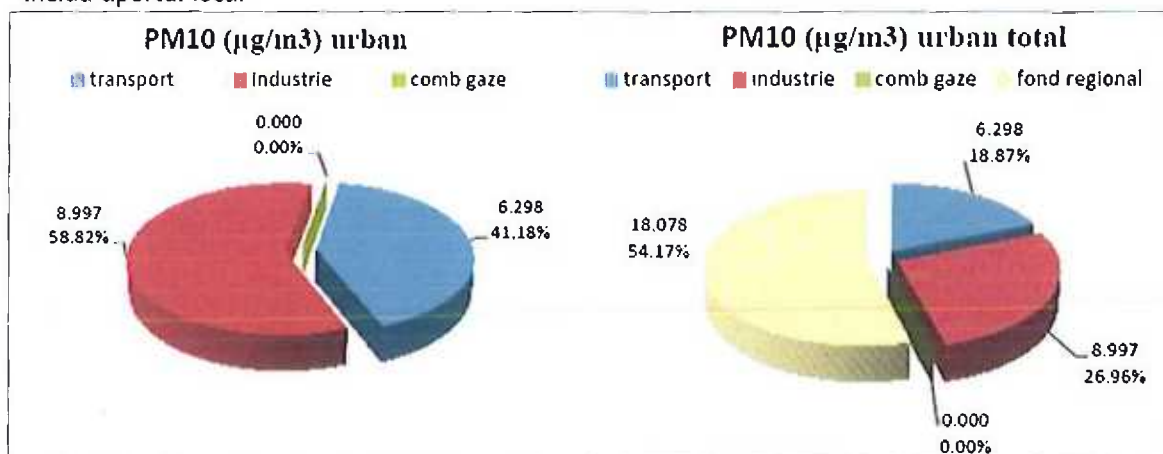
Figura nr. IV-3 Nivelul PM10 în anul de proiecție, cu aplicarea măsurilor PMCA-valori maxime* ale concentrațiilor medii anuale
