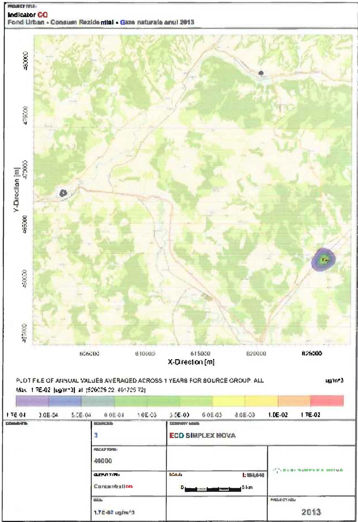
Figura nr. III-15 Creștere nivel Fond urban – Consum Rezidențial GN GO
