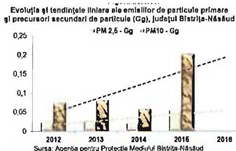
Figura nr. III-3 Evoluția emisiilor totale în perioada 2012-2015
