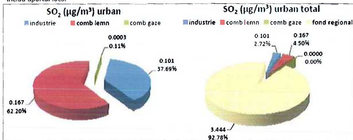
Figura nr,IV-11 Nivelul SO 2 în anul de proiecție, cu aplicarea măsurilor PMCA –valori maxime* concentrații la 24 de ore *inclus aportul local
