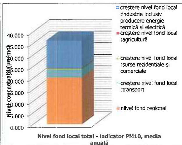
Figura nr. III-90Fond local total – indicator PM10
