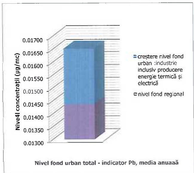
Figura nr. III-36 Nivel Fond urban total – indicator Pb
