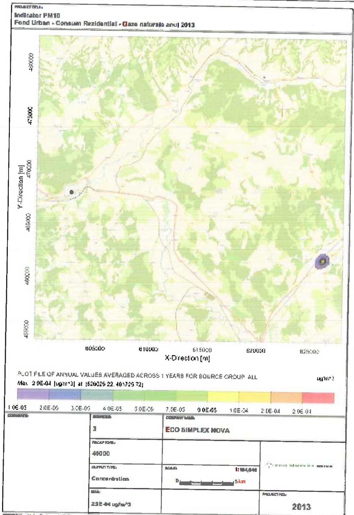
Figura nr. III-16 Creștere nivel Fond urban – Consum Rezidențial GN – PM10
