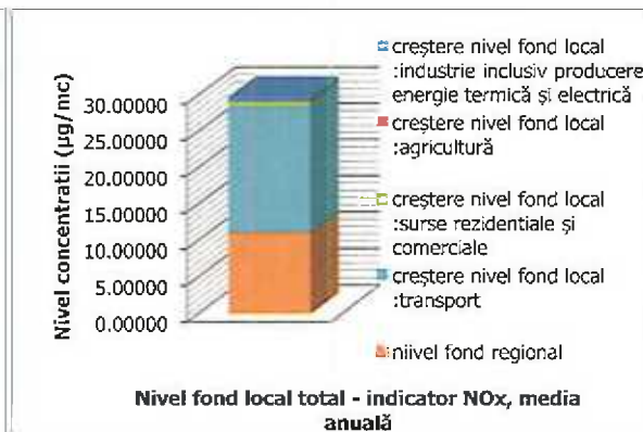
Figura nr. III-88 Fond local total – indicator NOx
