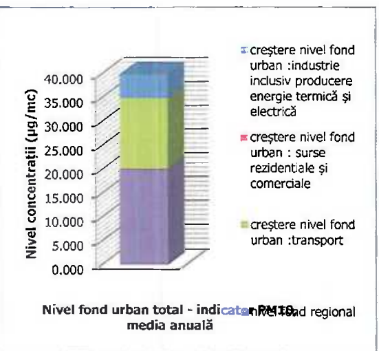
Figura nr. III-31 NivelFond urban total – indicator PM10
