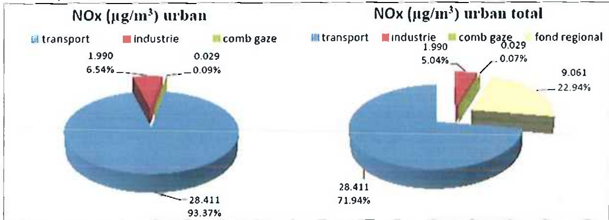
Figura nr. IV-6 Nivelul NO 2 și NO x în anul de proiecție, fără aplicarea măsurilor PMCA - valori maxime* concentrații medii anuale *includ aportul local
