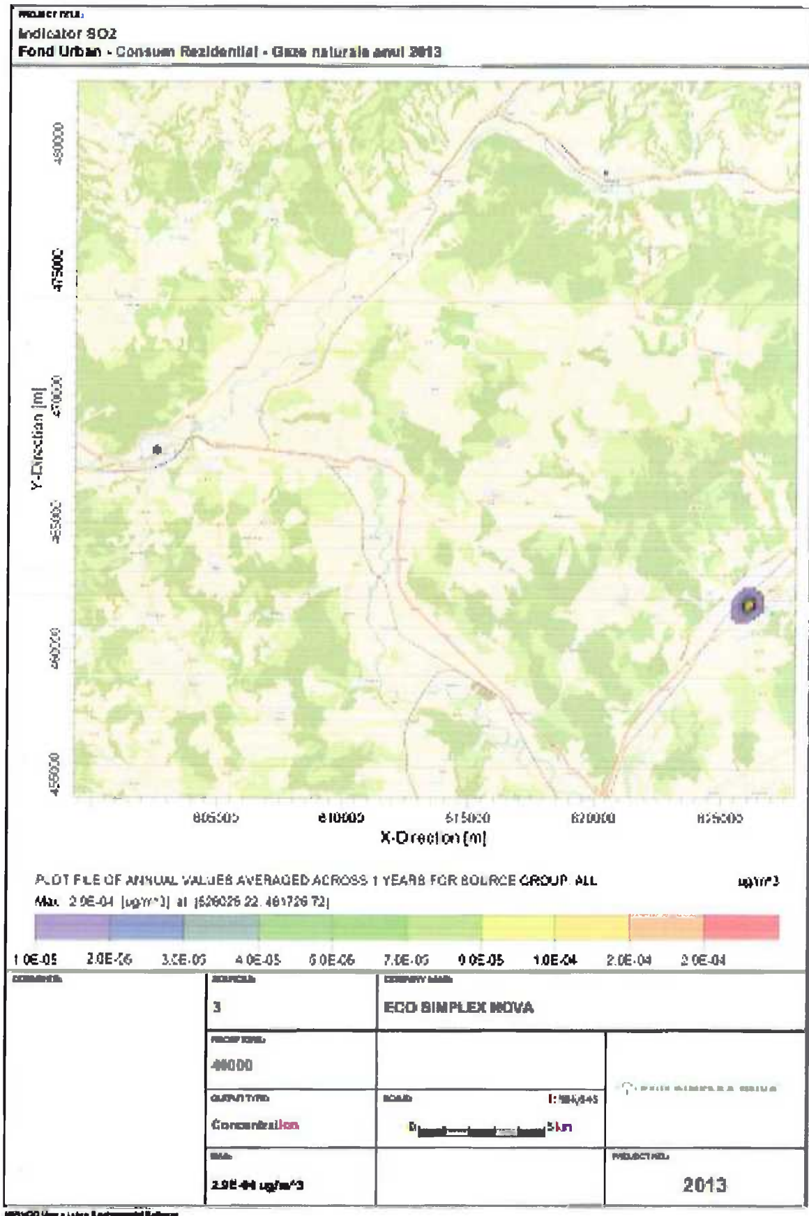
Figura nr. III-13 Creșterea nivelului Fond urban – Consum Rezidential GN- SO 2
