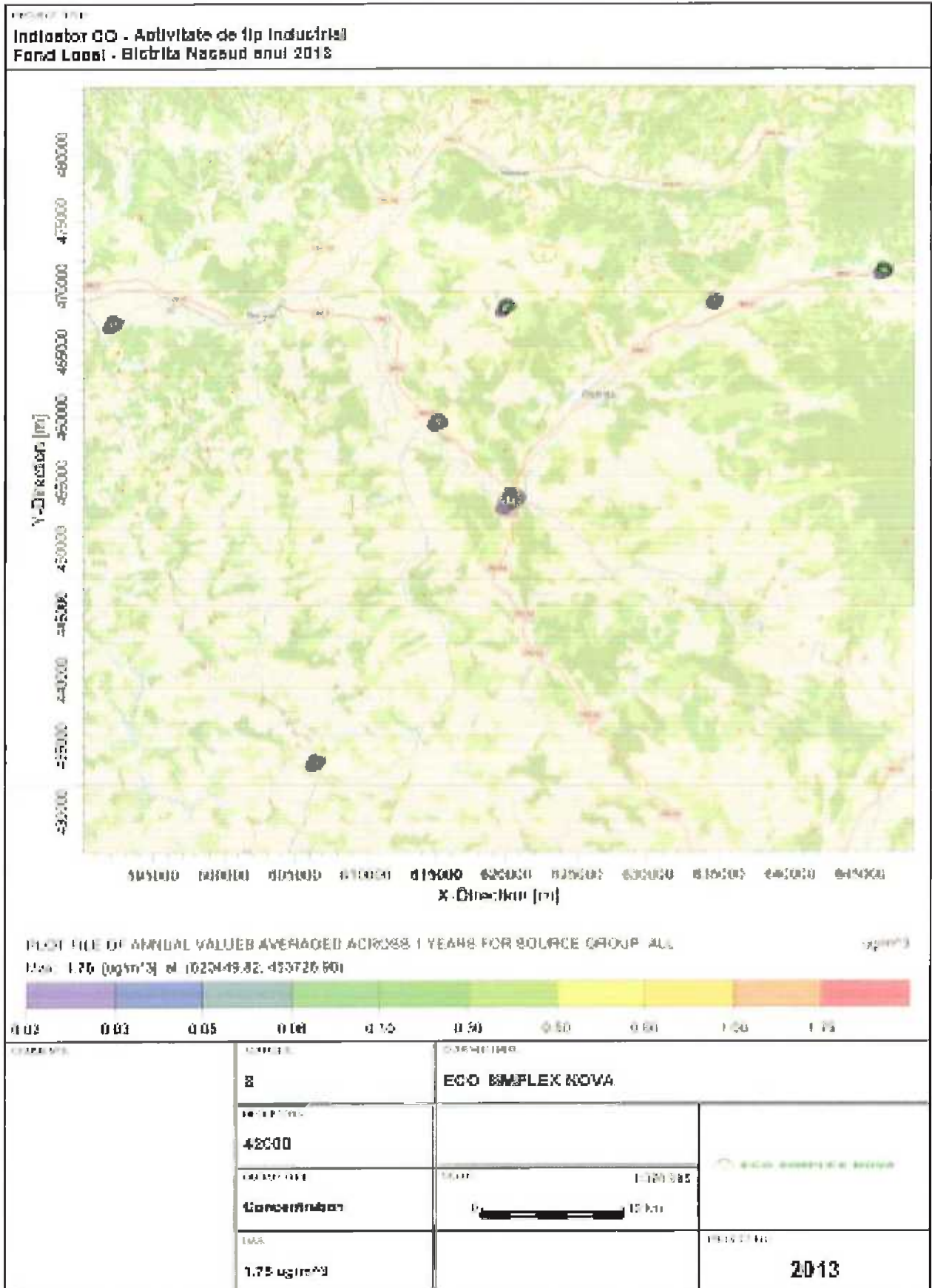
Figura nr. III-40 Creștere nivel Fond Local – Industrie – Indicator CO
