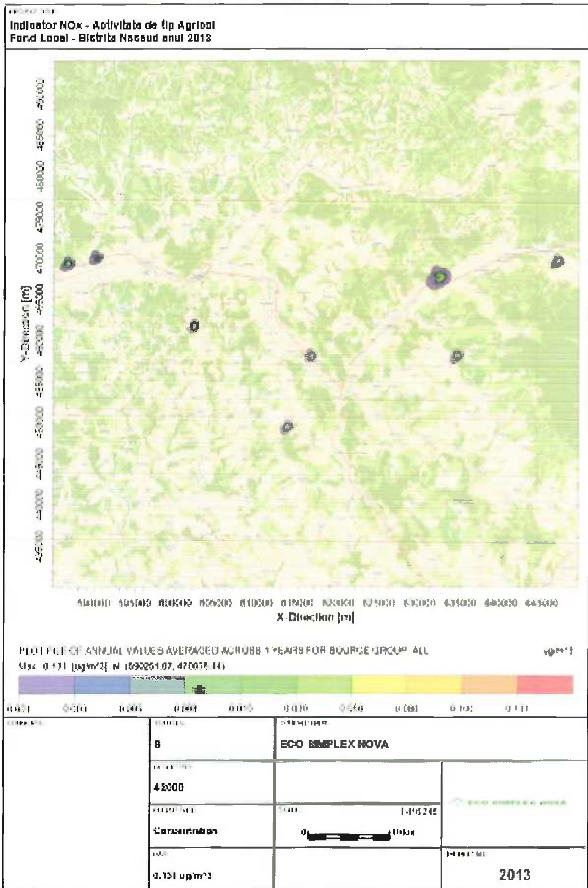
Figura nr. III-46 Creștere nivel Fond local – Agricultură – Indicator NOx
