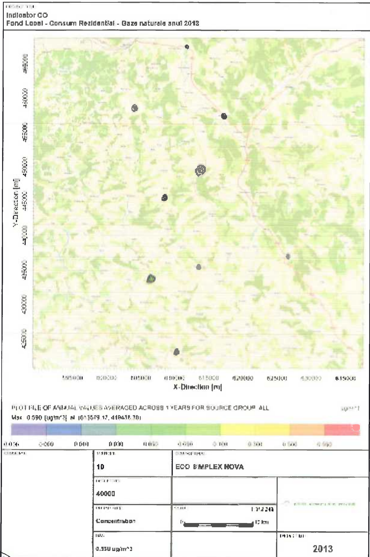
Figura nr. III-52 Creștere nivel Fond local- Consum Rezidențial GN- CO
