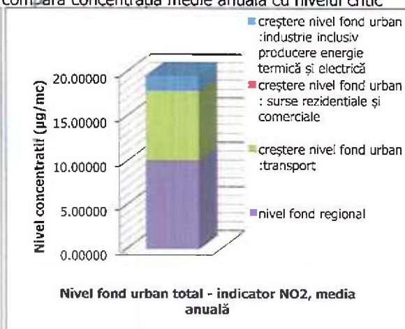
Figura nr. III-28 Nivel Fond urban total – indicator NO 2
