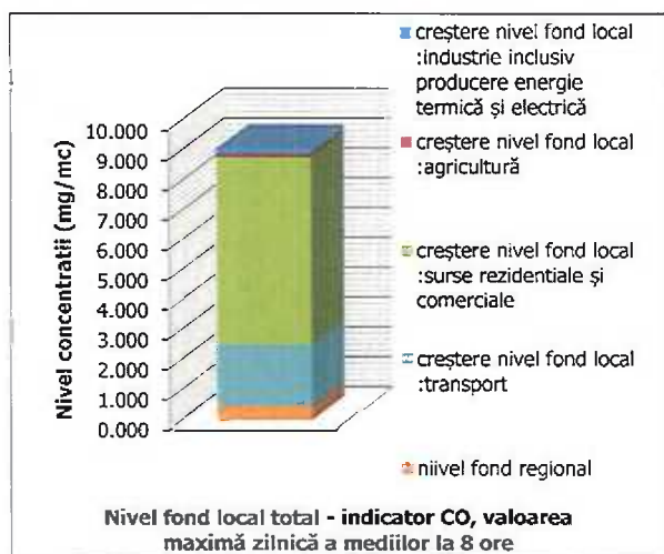
Figura nr. III-89Fond local total – indicator CO
