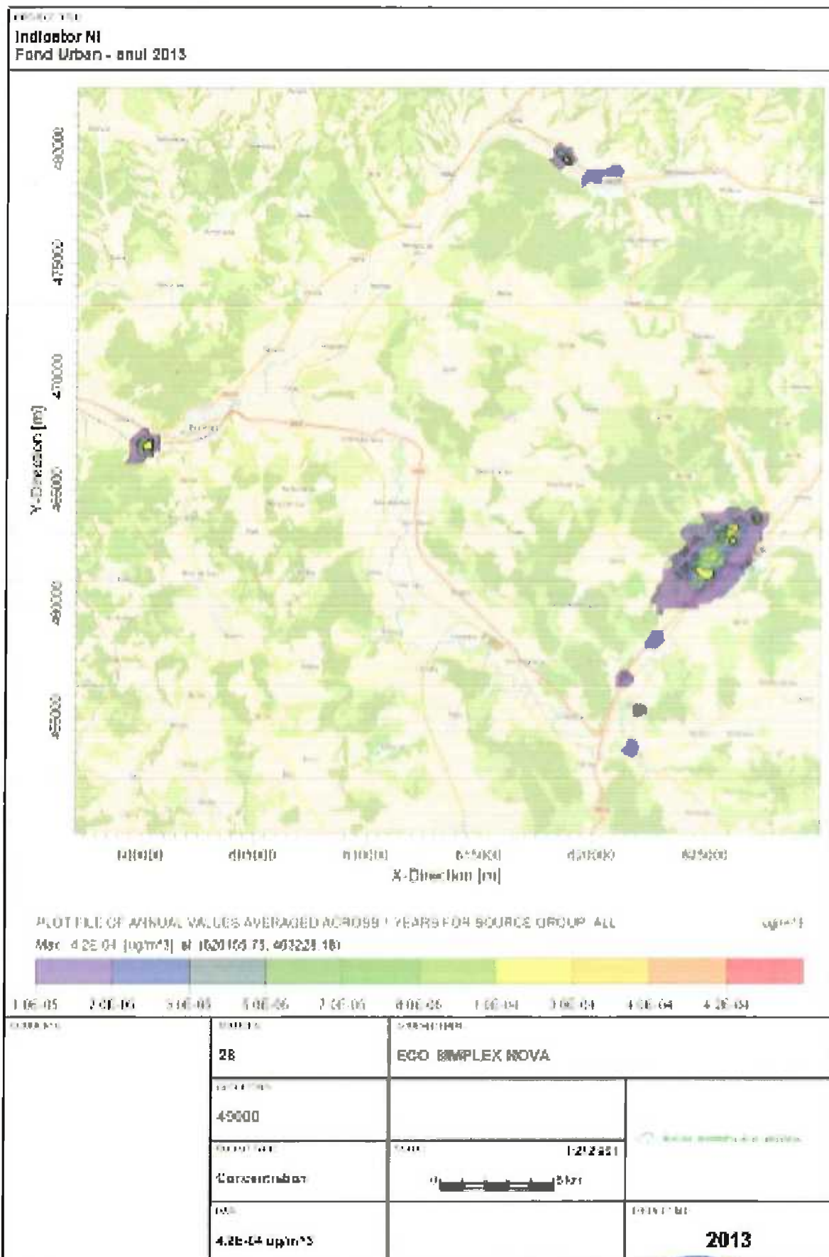
Figura nr. III-11 Creșterea nivelului Fondului urban – Industrie - Indicator Ni
