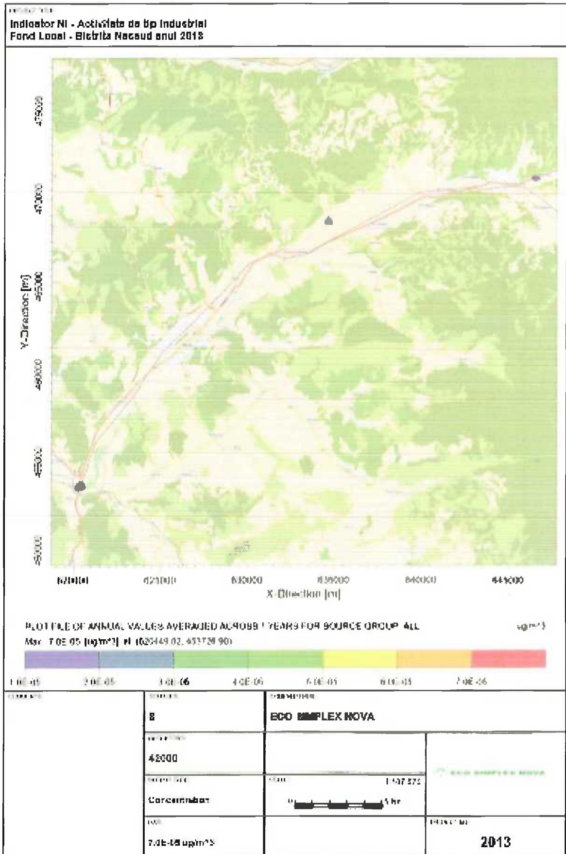
Figura nr. III-44 Creștere nivel Fond local – Industrie – Indicator Ni
