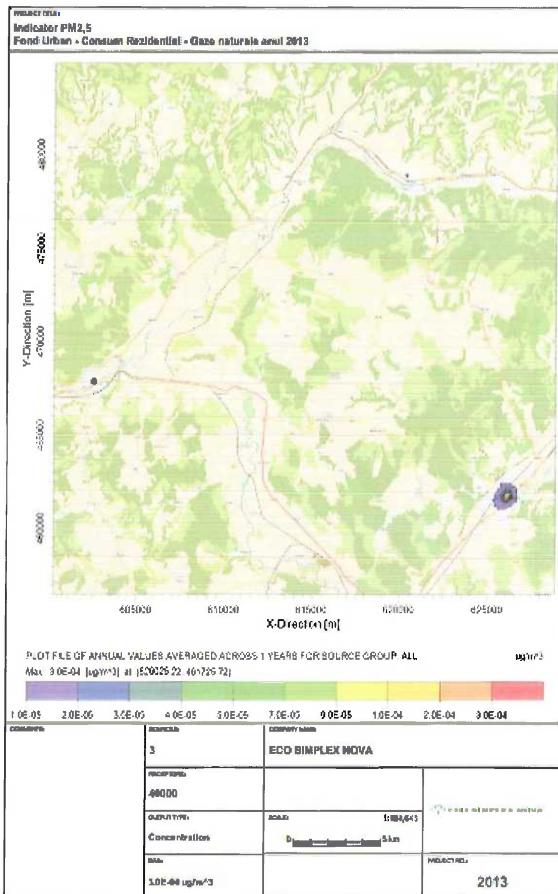
Figura nr. III-17 Creștere nivel Fond urban – Consum Rezidențial GN-PM2,5
