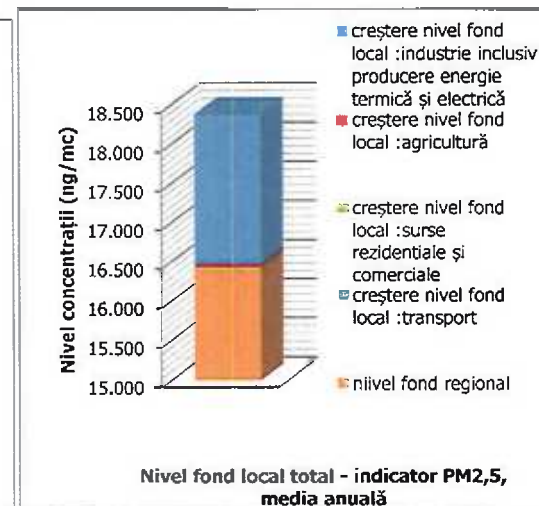
Figura nr. III-91Fond local total – indicator PM2,5
