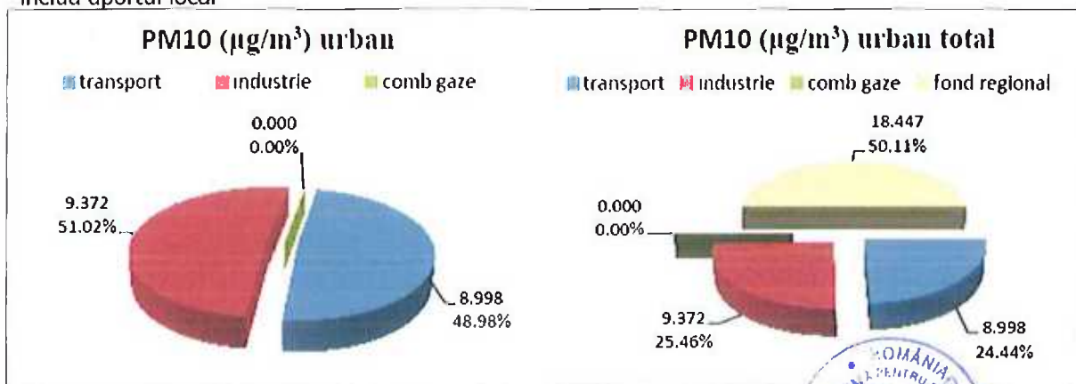
Figura nr. IV-2 Nivelul PM10 în anul de proiectie, fără aplicarea măsurilor PMCA-valori maxime* ale concentrațiilor medii anuale
