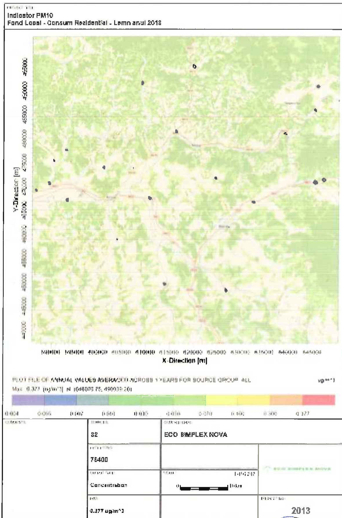
Figura nr. III-65 Creșterea nivelului Fond local – Consum rezidențial Lemn – PM10
