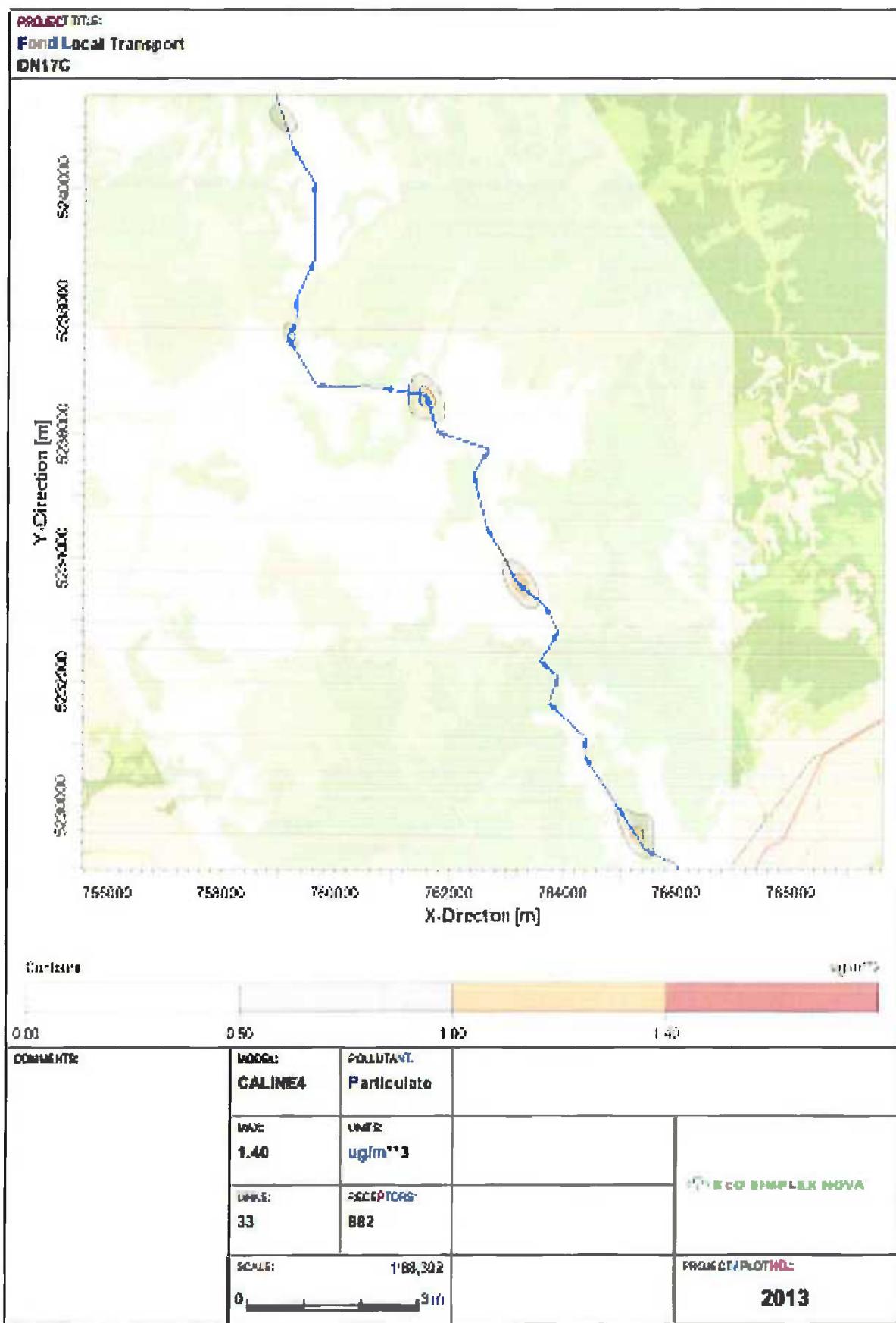
Figura nr. III-25 Creștere nivel fond local (rural) - Transport DN17C – PM10
