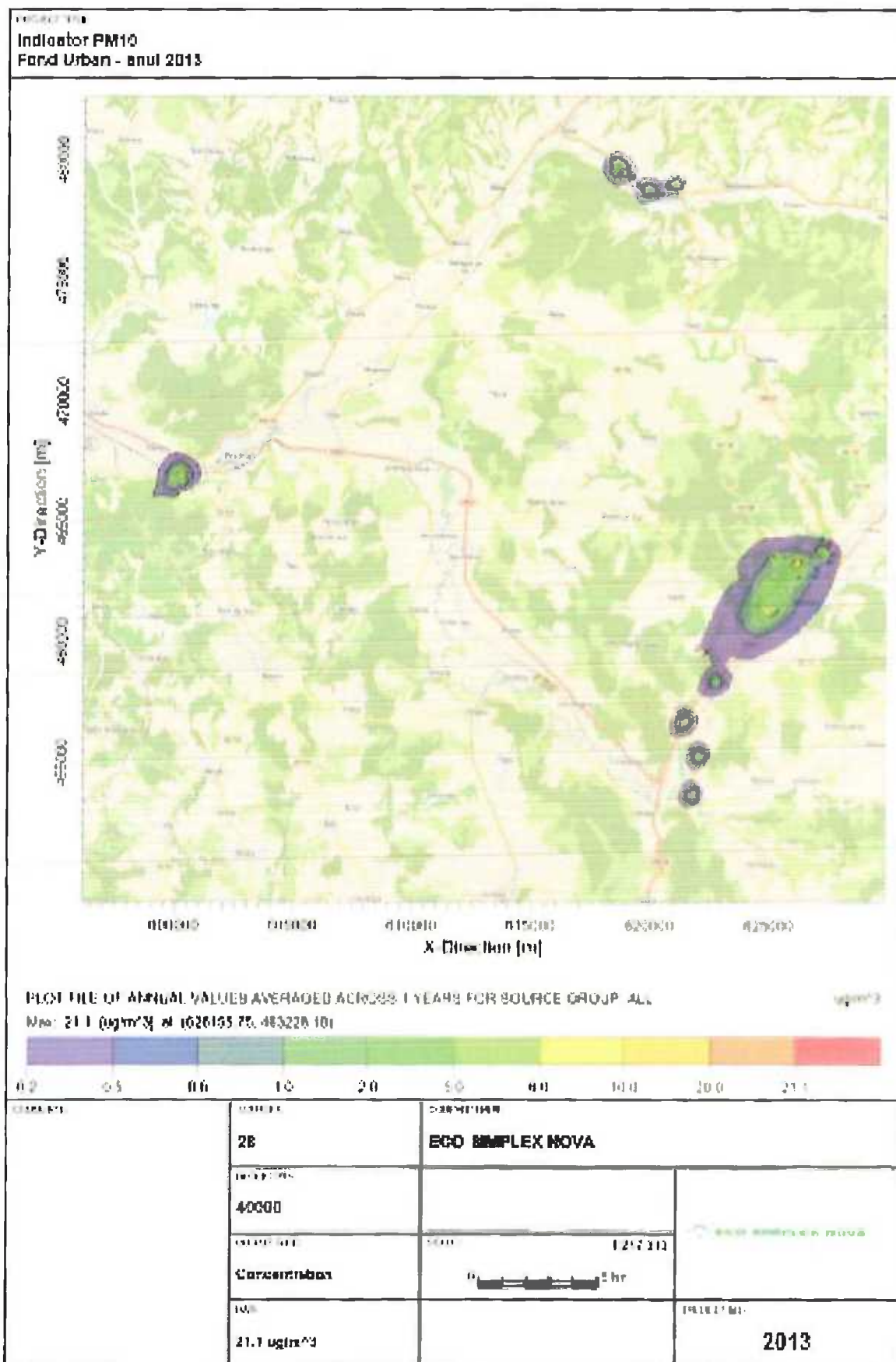
Figura nr. III-8 Creștere nivel Fond urban –Industrie - Indicator PM10
