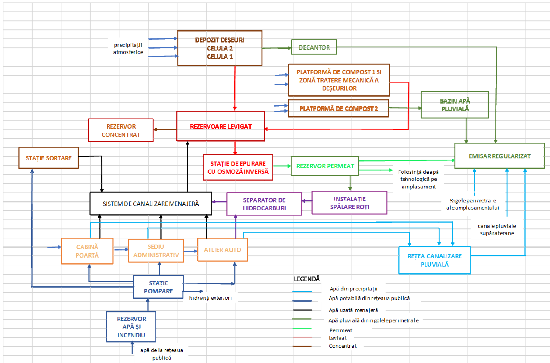
Figura 1. Diagrama circuitului apei – amplasament CMID Tâmpiu
