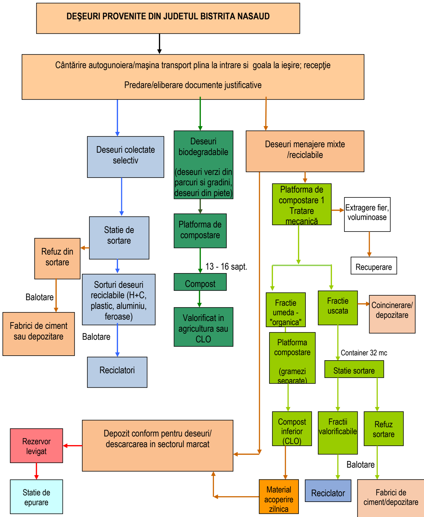
Figura 1 SCHEMA GENERALĂ DE FUNCȚIONARE A CMID TÂMPIU
