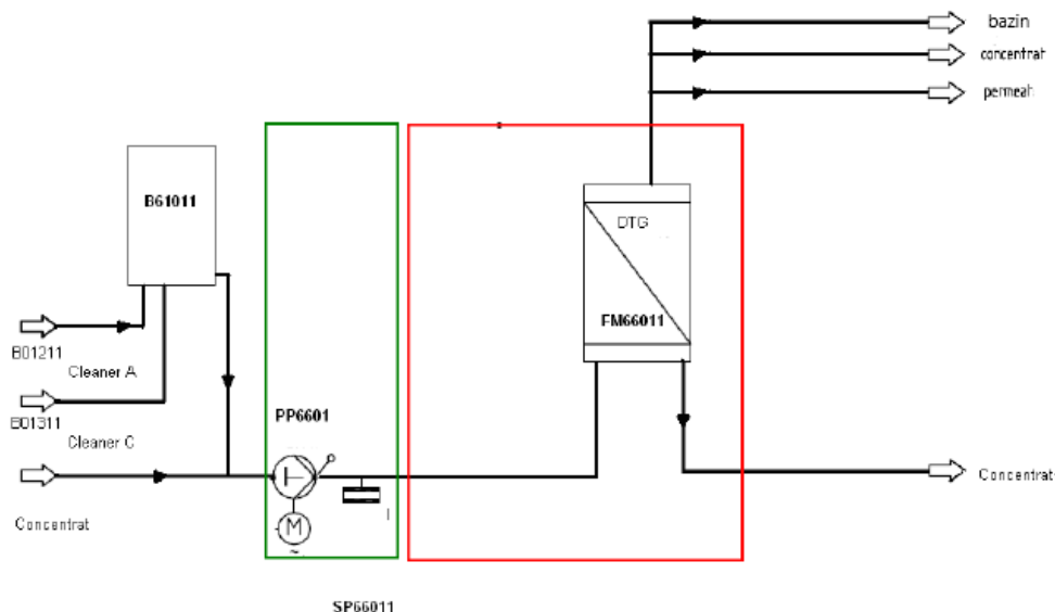
Figura 12 Diagrama specifică treptei de tratare concentrat
