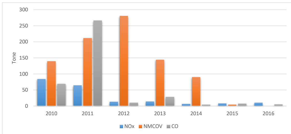
Figura nr. 4-9: Tendința emisiilor de poluanți precursori ai ozonului din sectorul de activitate industrie, la nivelul județului Brăila, în perioada 2010 - 2016
