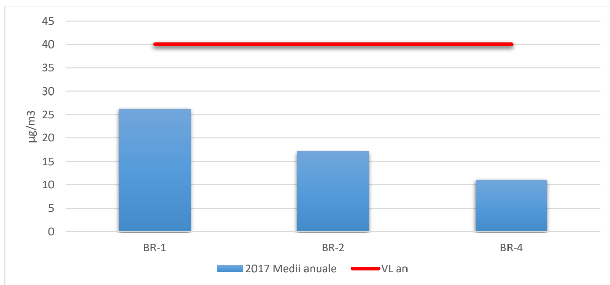
Figura nr. 5-15: Concentrația medie anuală a dioxidului de azot (NO 2 ), înregistrată la cele trei stații automate de monitorizare a calității aerului din aglomerarea Brăila, în anul 2017
