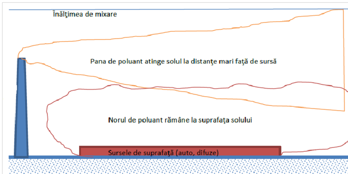
Figura nr. 5-11: Prezentarea schematică a dispersiei poluanților
