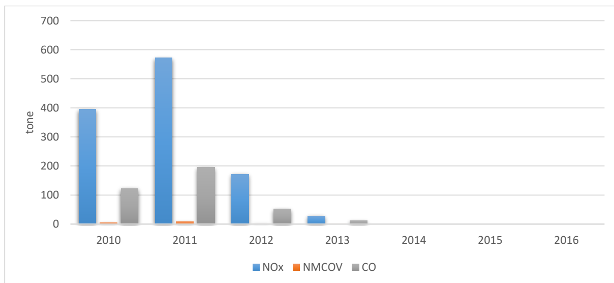
Figura nr. 4-8: Tendința emisiilor de poluanți precursori ai ozonului din sectorul de activitate energie, la nivelul județului Brăila, în perioada 2010 - 2016
