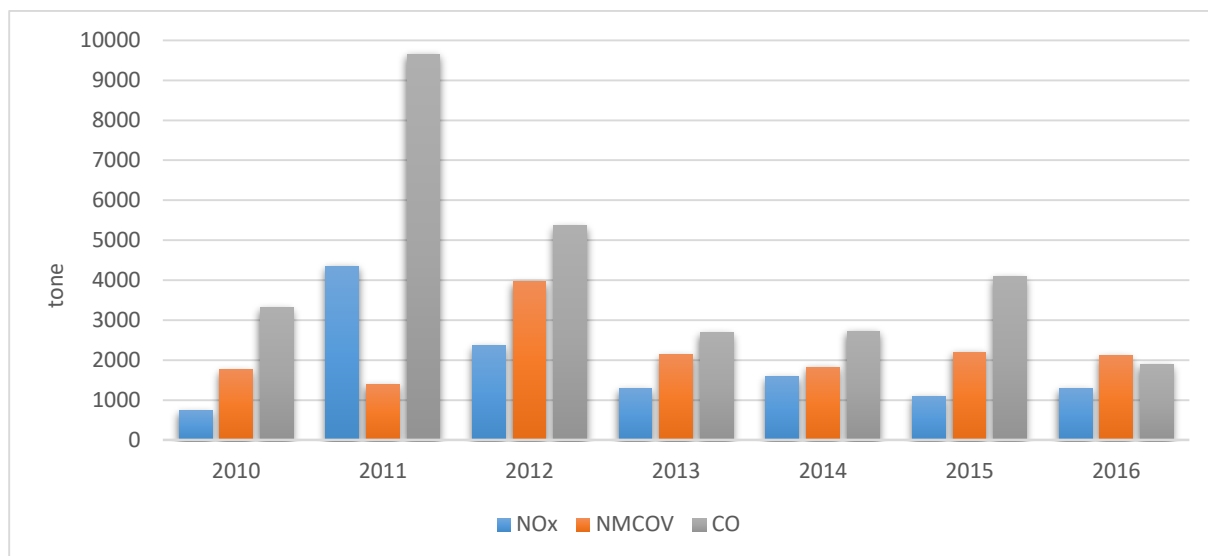
Figura nr. 4-7: Tendința emisiilor de poluanți precursori ai ozonului, la nivelul județului Brăila, în perioada 2010 - 2016
