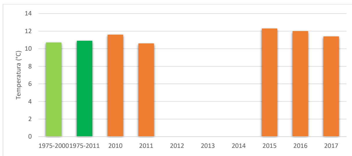
Figura nr. 2-3: Temperatura medie anuală a aerului (°C) din perioada 2010 – 2017 comparativ cu temperatura medie multianuală (°C) din perioada 1975-2000 și 1975 – 2011 la Stația meteorologică Brăila
