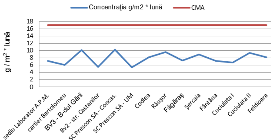
Figura 1.1.1.2. Cantitatea de pulberi sedimentabile în județul Brașov
