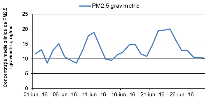
Figura 1.1.2.4.4 Evoluția mediilor zilnice de PM 2,5 în luna iunie
