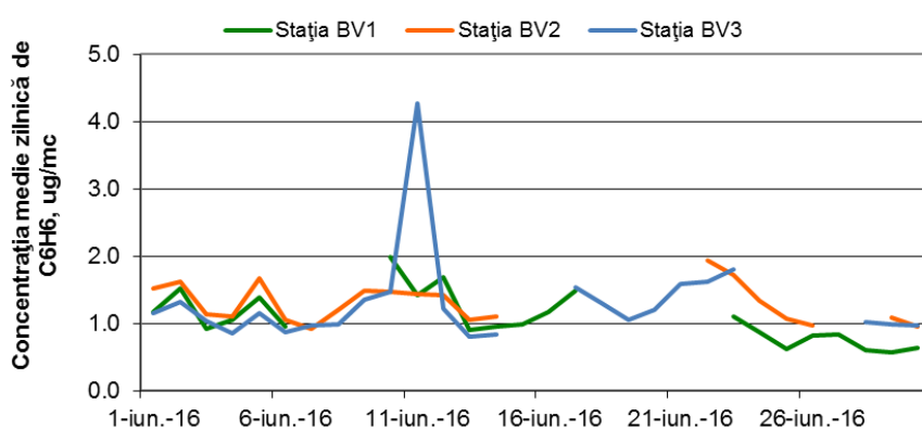
Figura 1.1.2.6.1: Evoluția mediilor zilnice de benzen în luna iunie
