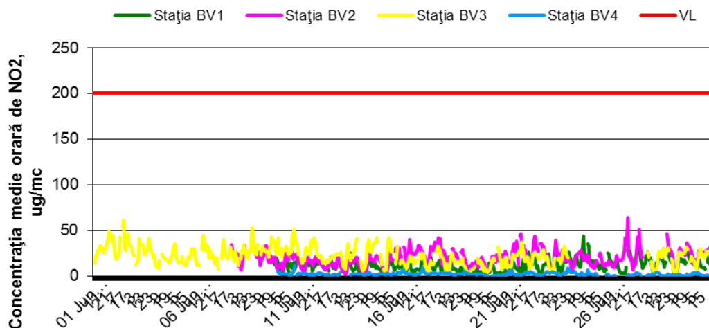
Figura 1.1.2.2.1. Evoluția mediilor orare de \text{NO}_2 în luna iunie
