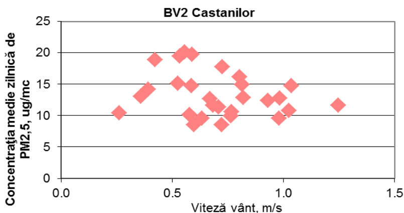
Figura 1.1.2.4.5. Evoluția mediilor zilnice de PM2,5 în funcție de viteza vântului la BV2
