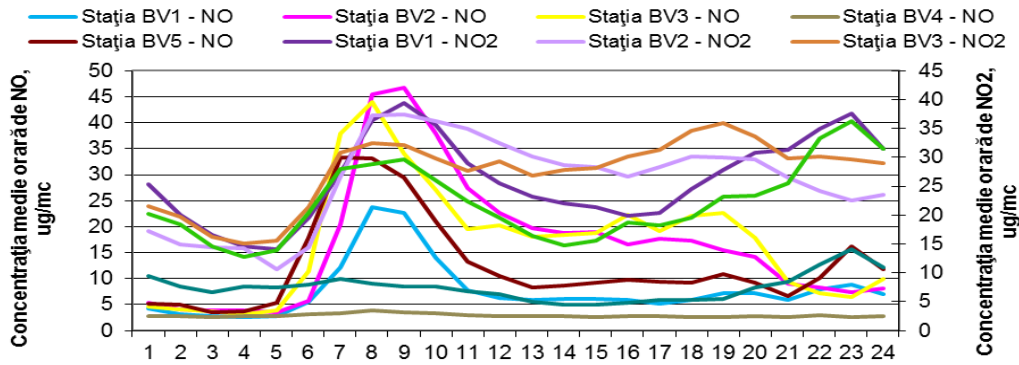
Figura 1.1.2.2.2. Ciclul zilnic al NO 2 și NO
