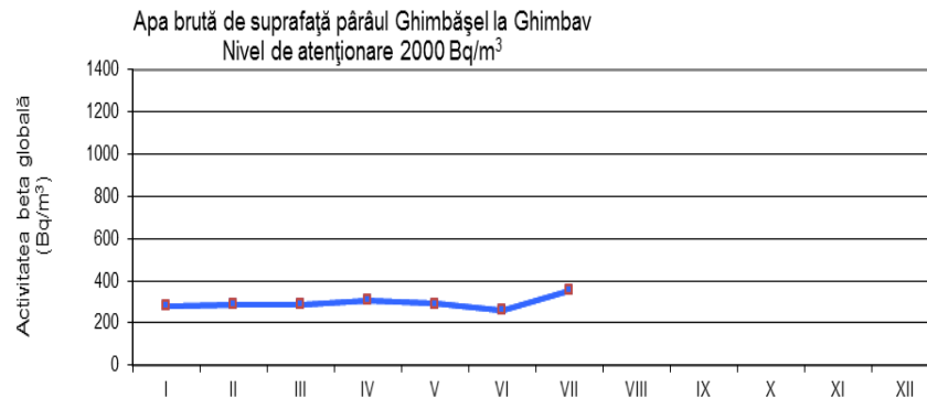
Fig. 1.3.5. Activitatea beta globală imediată pentru apa de suprafață Pârâu Ghimbășel
