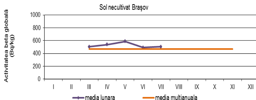
Fig. 1.3.8. Activitatea beta globală – la 5 zile - pentru sol necultivat Brașov.
