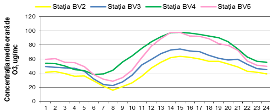
Figura 1.1.2.3.2. Ciclul zilnic al ozonului
