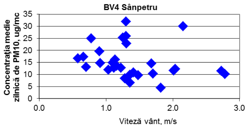
Figura 1.1.2.4.2. Evoluția mediilor zilnice de PM 10 în funcție de viteza vântului la stațiile BV2, BV3 și BV4
