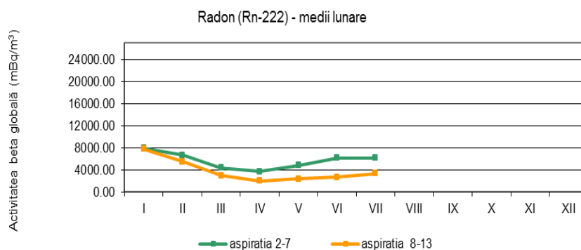
Fig. 1.3.2. Activitatea calculată a Radonului
