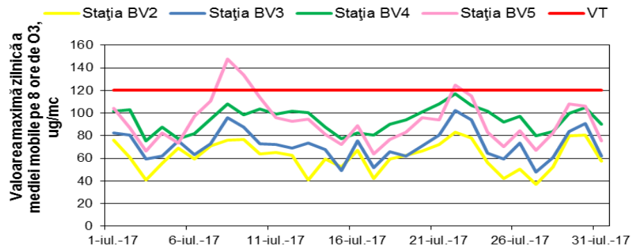
Figura 1.1.2.3.1. Evoluția maximelor zilnice ale mediilor mobile pe 8 ore de O 3 în luna iulie
