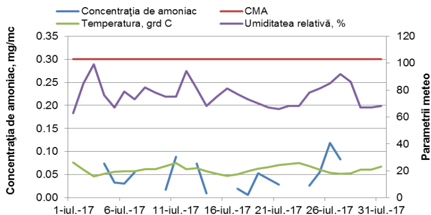
Figura 1.1.1.1.1. Evoluția mediilor de scurtă durată de amoniac în luna iulie 2017
