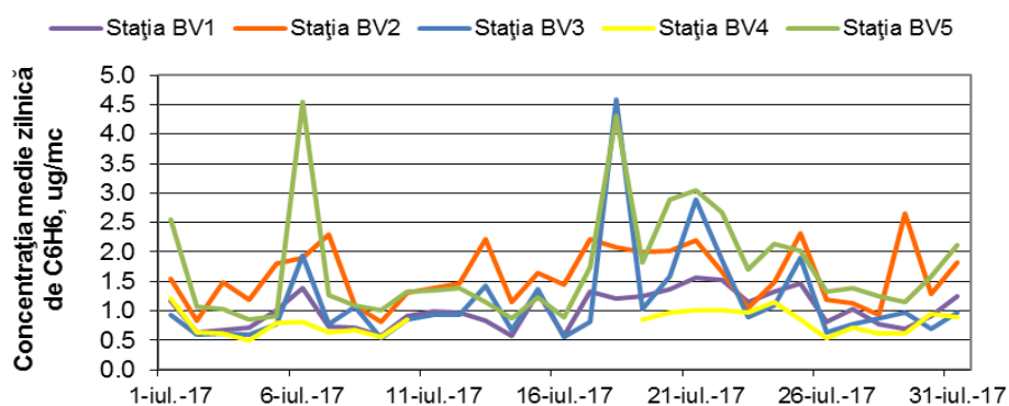
Figura 1.1.2.6.1: Evoluția mediilor zilnice de benzen în luna iulie
