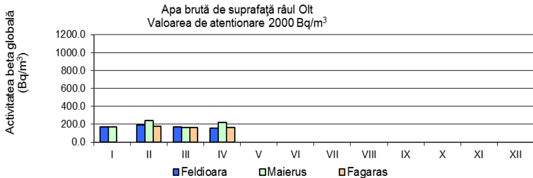
Fig. 1.4.7. Activitatea beta globală – la 5 zile - pentru apa de suprafață Râul OLT
