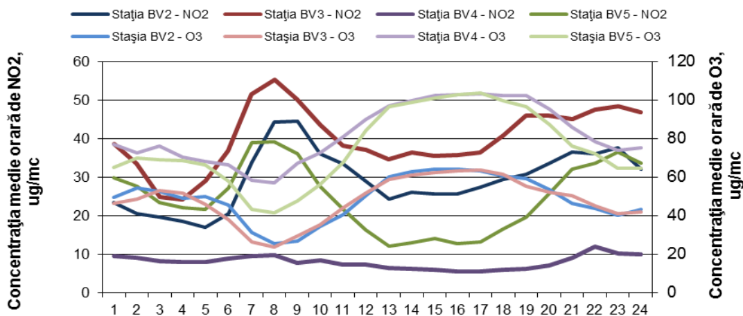
Figura 1.1.2.3.3. Ciclu zilnic al \text{O}_3 și \text{NO}_2
