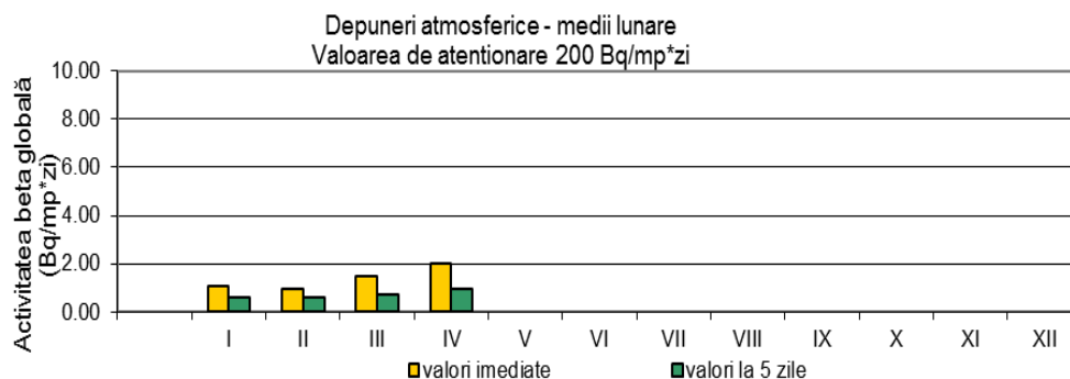
Fig. 1.4.4. Activitatea beta globală pentru depuneri atmosferice
