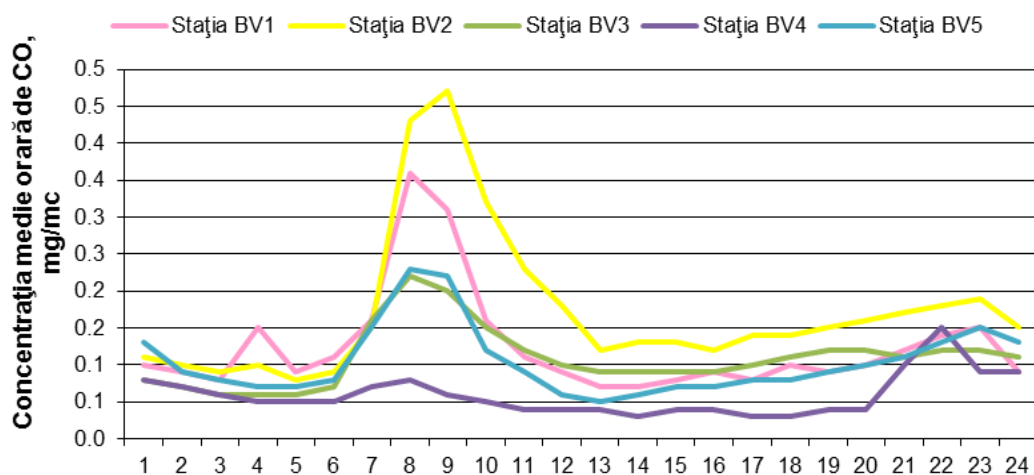
Figura 1.1.2.5.2. Ciclul zilnic al CO
