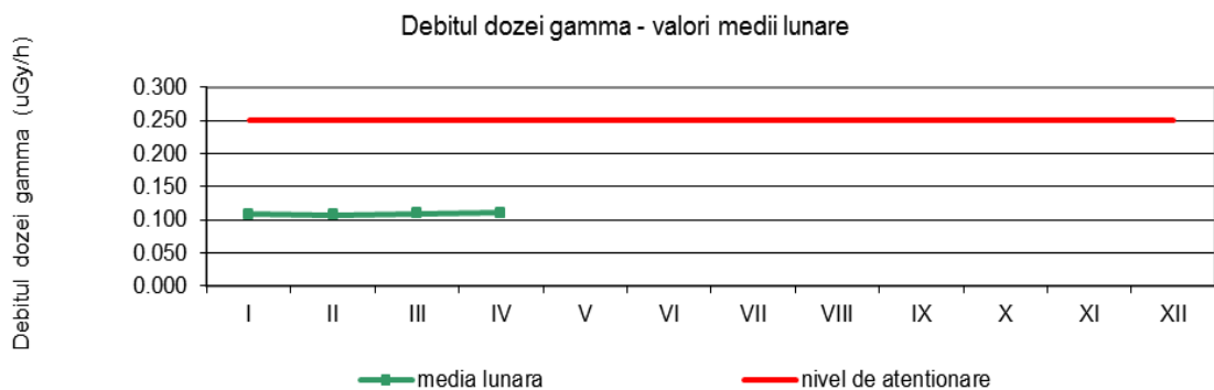
Fig. 1.4.3. Debitul dozei gamma în aer
