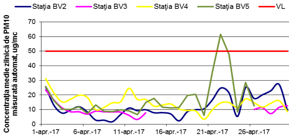
Figura 1.1.2.4.1. Evoluția mediilor zilnice de PM 10 în luna aprilie
