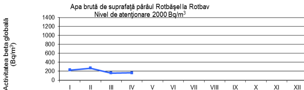
Fig. 1.4.6. Activitatea beta globală – la 5 zile-pentru apa de suprafață-Pârâu Rotbășel
