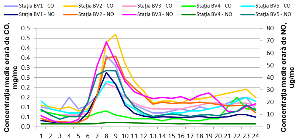
Figura 1.1.2.2.4. Ciclul zilnic al NO și CO
