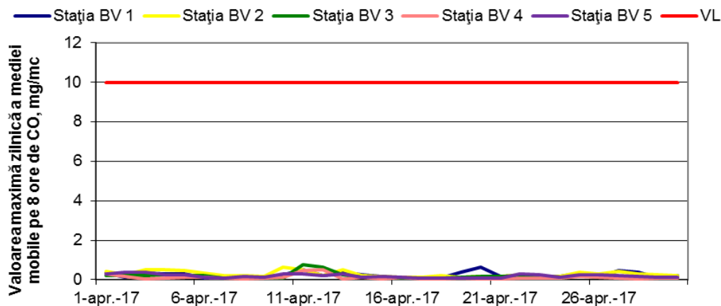
Figura 1.1.2.5.1. Evoluția maximelor zilnice ale mediei mobile de CO în luna aprilie
