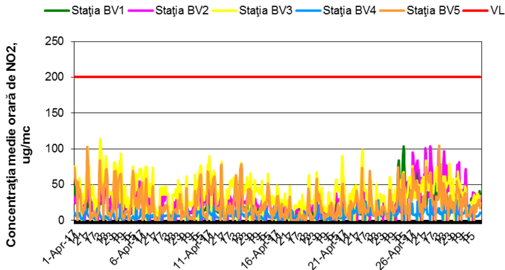
Figura 1.1.2.2.1. Evoluția mediilor orare de \text{NO}_2 în luna aprilie
