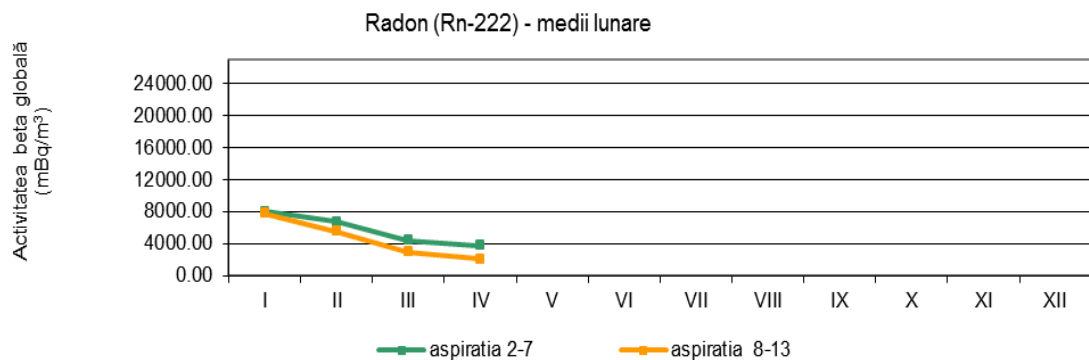
Fig. 1.4.2. Activitatea calculată a Radonului
