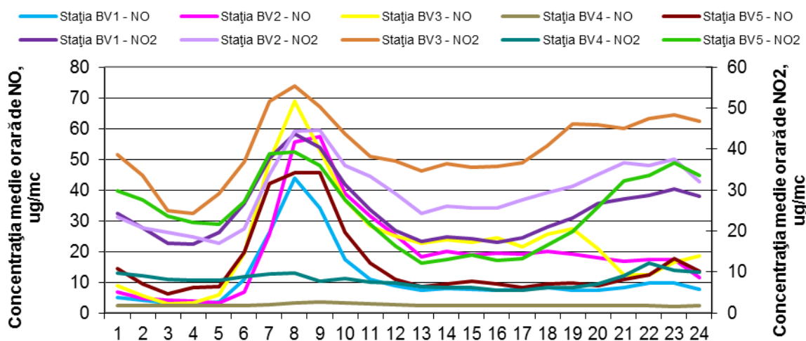
Figura 1.1.2.2.2. Ciclul zilnic al \text{NO}_2 și \text{NO}
