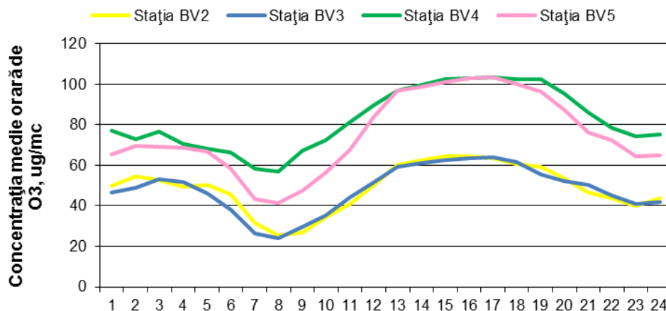
Figura 1.1.2.3.2. Ciclu zilnic al ozonului
