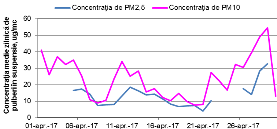
Figura 1.1.2.4.4 Evoluția mediilor zilnice de PM 2,5 și PM 10 în luna aprilie
