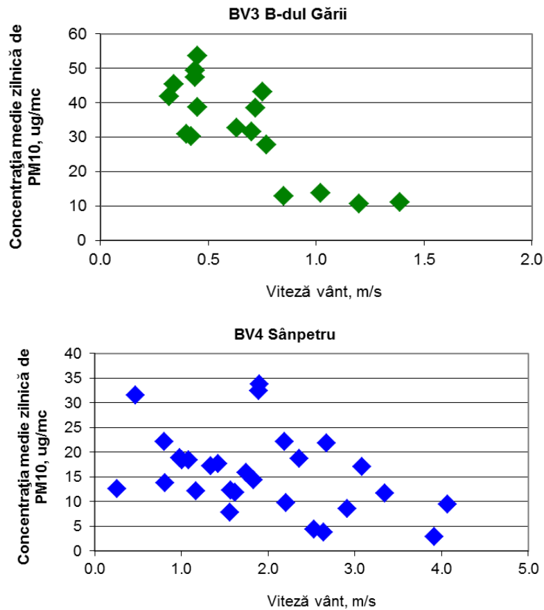
Figura 1.1.2.4.2. Evoluția mediilor zilnice de PM 10 în funcție de viteza vântului la stațiile BV2, BV3 și BV4
