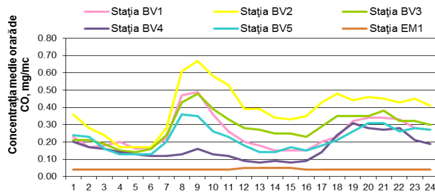
Figura 1.1.2.5.2. Ciclul zilnic al CO
