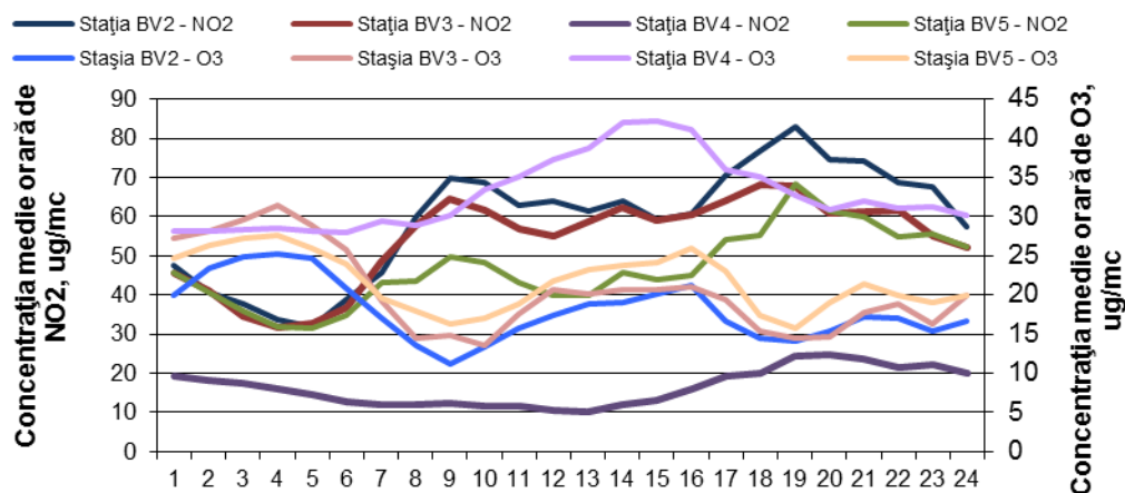
Figura 1.1.2.3.3. Ciclul zilnic al O 3 și NO 2
