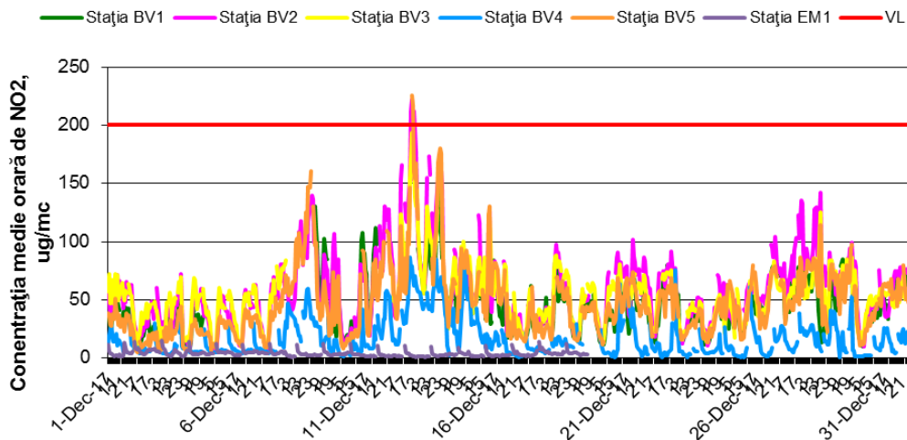
Figura 1.1.2.2.1. Evoluția mediilor orare de NO 2 în luna decembrie
