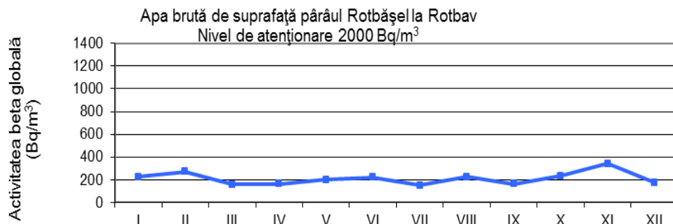
Fig. 1.3.6. Activitatea beta globală la 5 zile pentru apa de suprafață-Pârâu Rotbășel
