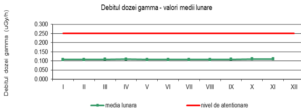
Fig. 1.3.3. Debitul dozei gamma în aer
