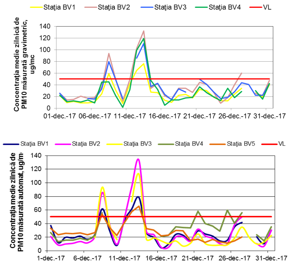
Figura 1.1.2.4.1. Evoluția mediilor zilnice de PM 10 în luna decembrie
