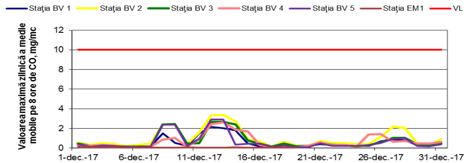
Figura 1.1.2.5.1. Evoluția maximelor zilnice ale mediei mobile de CO în luna decembrie
