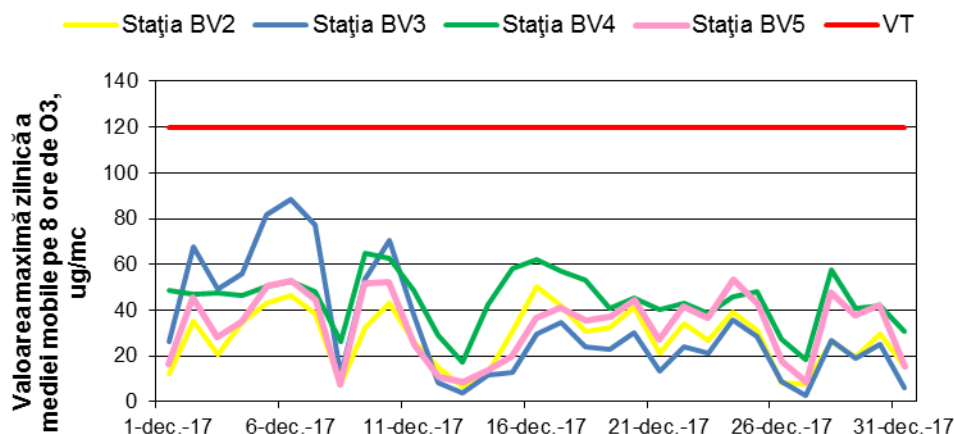
Figura 1.1.2.3.1. Evoluția maximelor zilnice ale mediilor mobile pe 8 ore de O 3 în luna decembrie
