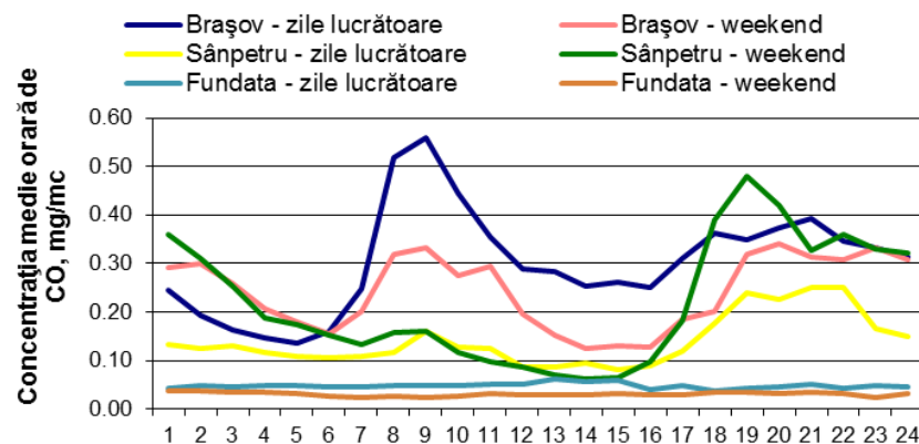
Figura 1.1.2.5.3. Ciclul zilnic al CO în timpul săptămânii
