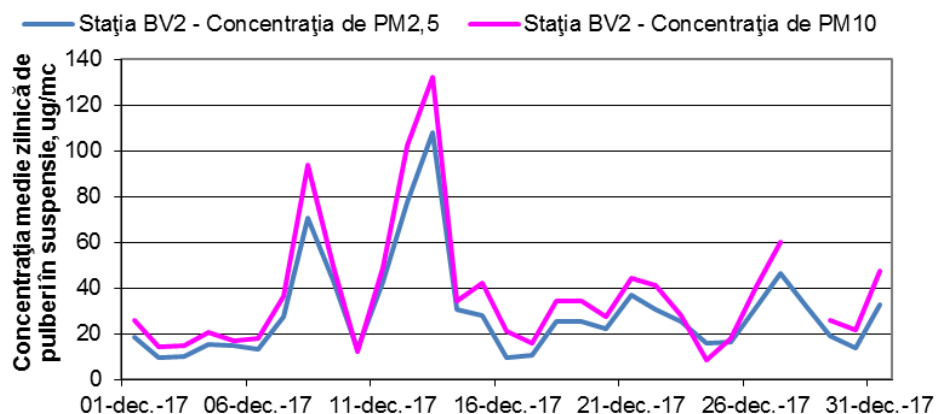
Figura 1.1.2.4.4 Evoluția mediilor zilnice de PM 2,5 și PM10 în luna decembrie
