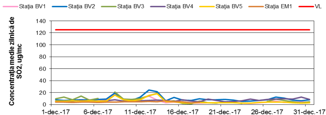
Figura 1.1.2.1.1. Evoluția mediilor zilnice de \text{SO}_2 în luna decembrie
