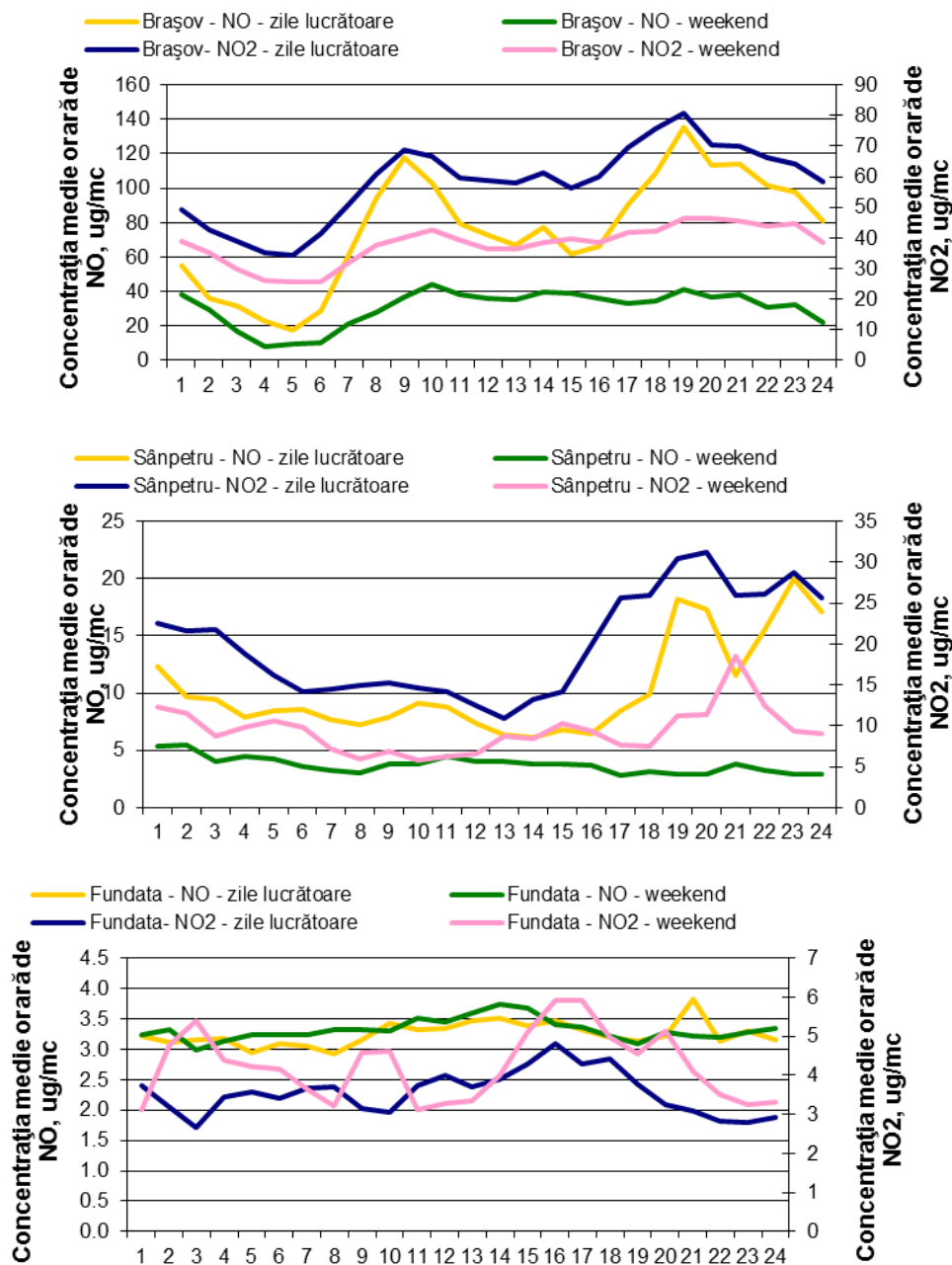
Figura 1.1.2.2.3. Ciclul zilnic al oxizilor de azot în timpul săptămânii
