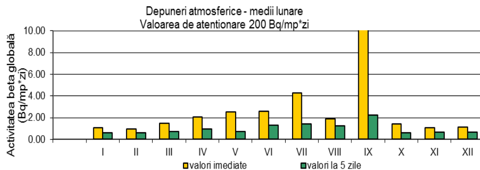
Fig. 1.3.4. Activitatea beta globală pentru depuneri atmosferice
