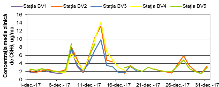
Figura 1.1.2.6.1: Evoluția mediilor zilnice de benzen în luna decembrie
