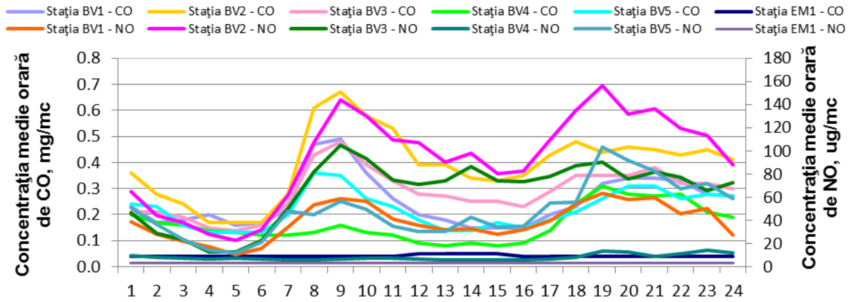
Figura 1.1.2.2.4. Ciclul zilnic al NO și CO
