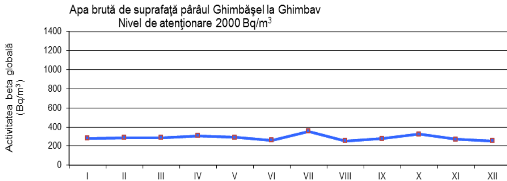
Fig. 1.3.5. Activitatea beta globală imediată pentru apa de suprafață Pârâu Ghimbășel
