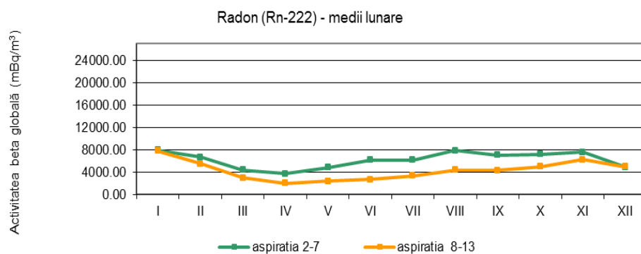
Fig. 1.3.2. Activitatea calculată a Radonului
