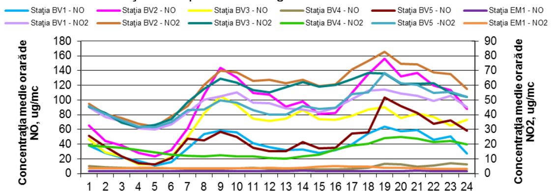
Figura 1.1.2.2.2. Ciclul zilnic al NO 2 și NO
