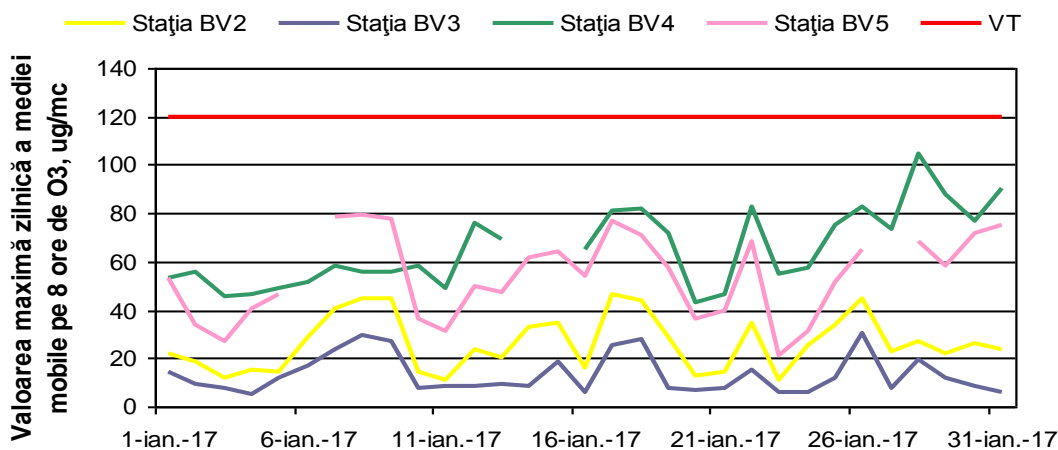
Figura 1.1.2.3.1. Evoluția maximelor zilnice ale mediilor mobile pe 8 ore de O 3 în luna ianuarie
