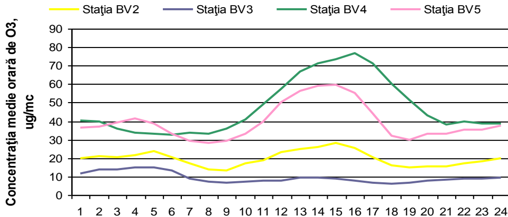
Figura 1.1.2.3.2. Ciclul zilnic al ozonului
