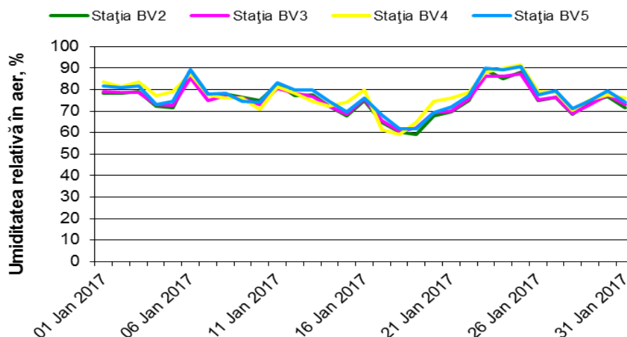
Figura 1.1.2.8.3. Evoluția zilnică a umidității relative înregistrate în luna ianuarie în stațiile de monitorizare BV2, BV3 și BV5 din Brașov și BV4 din Sânpetru
