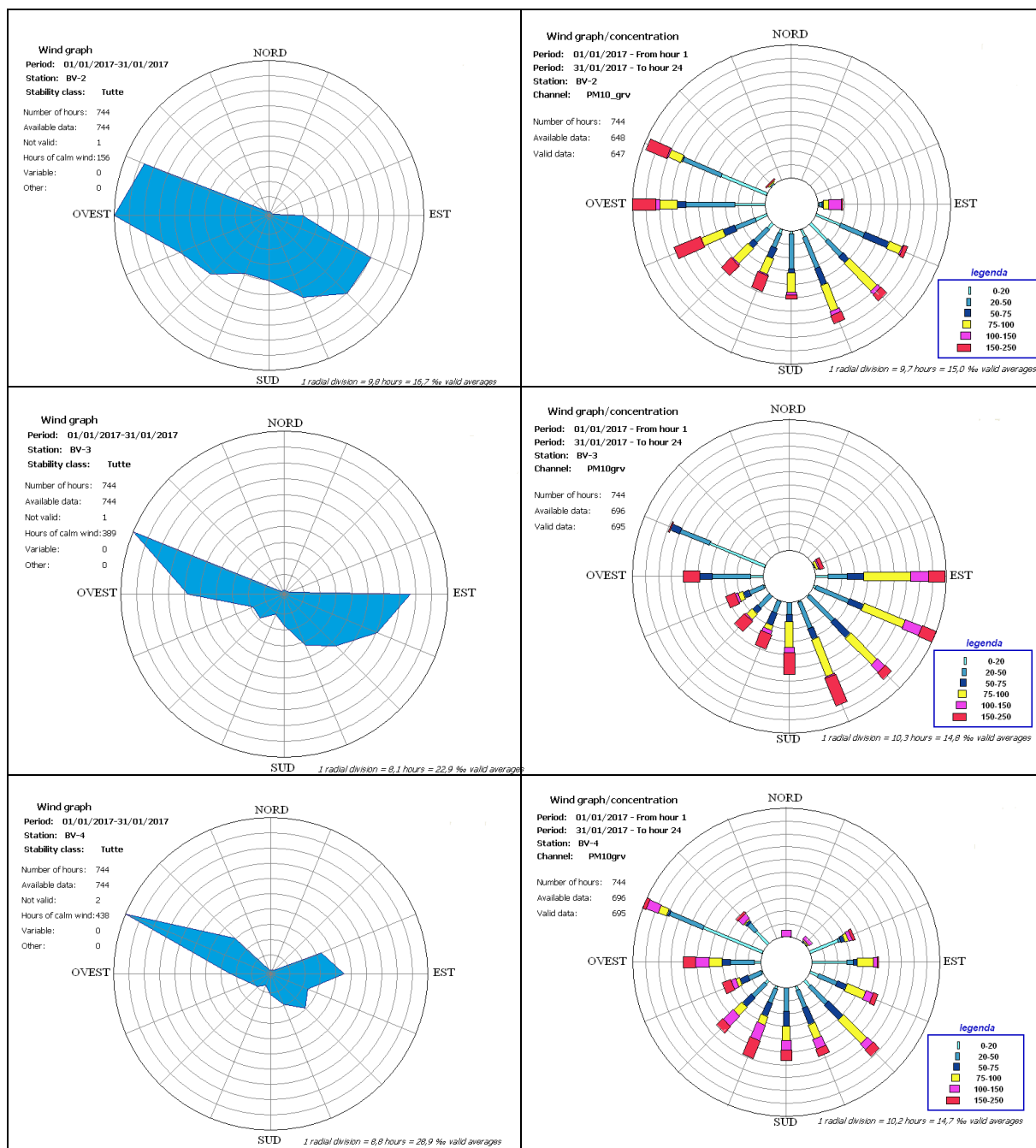
Figura 1.1.2.8.7. Grafic vânt și vânt – concentrație de PM10 la stația BV2, BV3 și BV4 în luna ianuarie 2017
