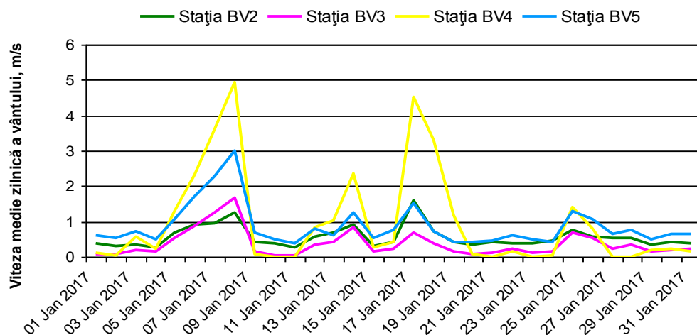
Figura 1.1.2.8.6. Viteza vântului înregistrată în luna ianuarie la stațiile de monitorizare BV2, BV3 și BV5 din Brașov și BV4 din Sânpetru
