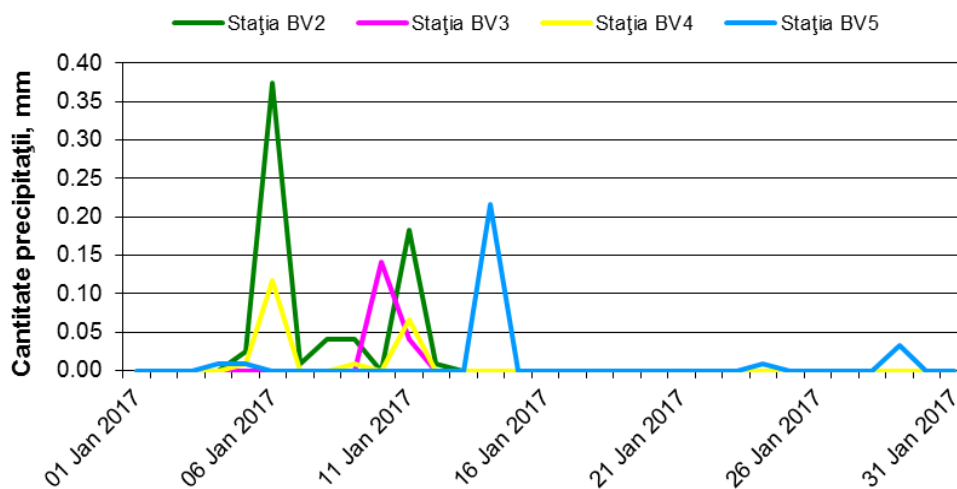
Figura 1.1.2.8.4. Evoluția zilnică a precipitațiilor înregistrate în luna ianuarie în stațiile de monitorizare BV2, BV3 și BV5 din Brașov și BV4 din Sânpetru
