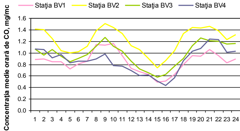
Figura 1.1.2.5.2. Ciclul zilnic al CO
