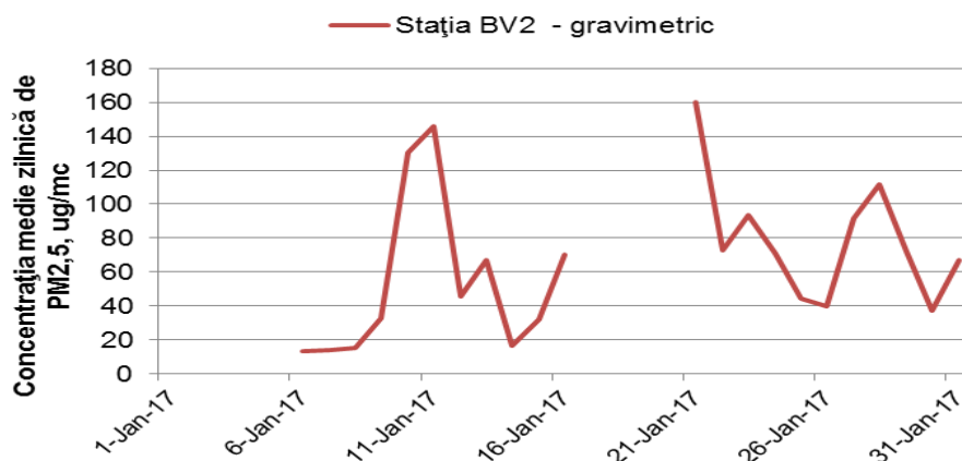
Figura 1.1.2.4.3 Evoluția mediilor zilnice de PM 2,5 în luna ianuarie
