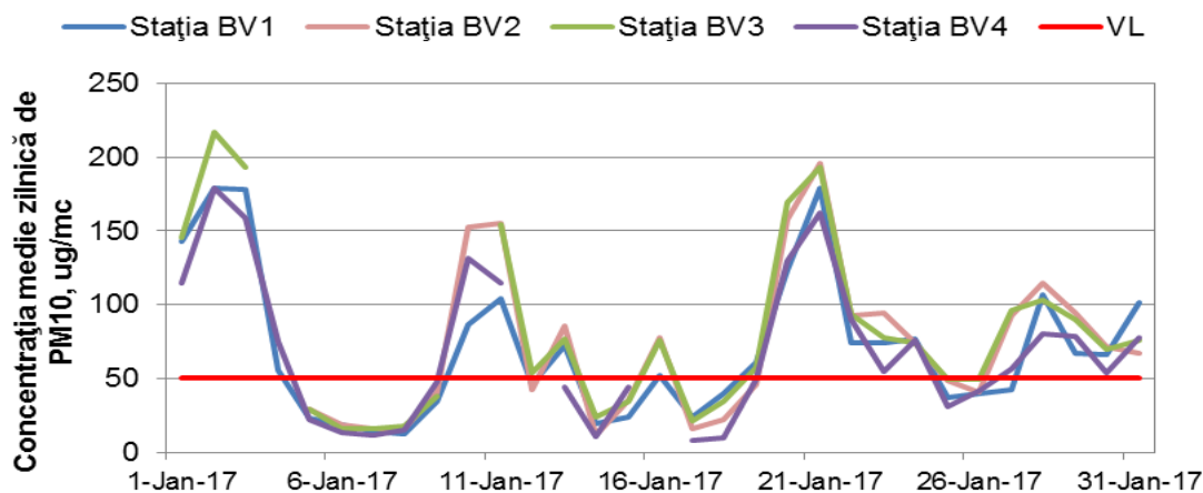
Figura 1.1.2.4.1. Evoluția mediilor zilnice de PM 10 în luna ianuarie
