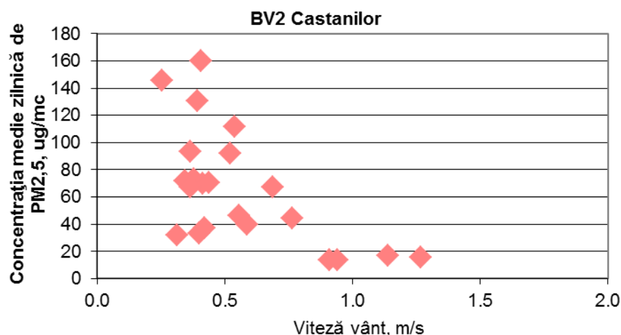
Figura 1.1.2.4.3. Evoluția mediilor zilnice de PM 2,5 în funcție de viteza vântului
