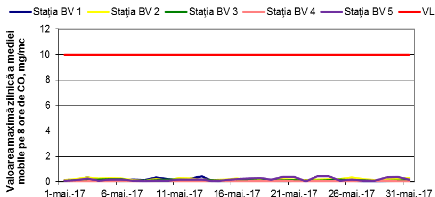
Figura 1.1.2.5.1. Evoluția maximelor zilnice ale mediei mobile de CO în luna mai
