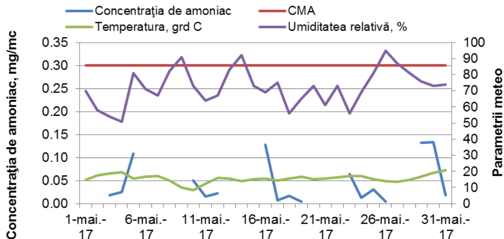
Figura 1.1.1.1.1. Evoluția mediilor de scurtă durată de amoniac în luna mai 2017
