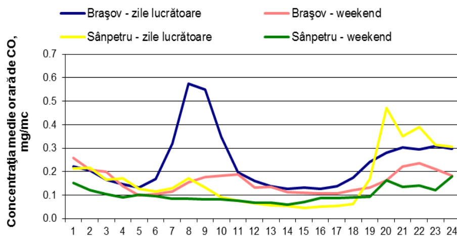
Figura 1.1.2.5.3. Ciclul zilnic al CO în timpul săptămânii
