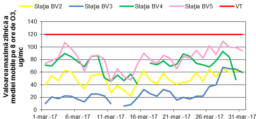
Figura 1.1.2.3.1. Evoluția maximelor zilnice ale mediilor mobile pe 8 ore de O 3 în luna martie
