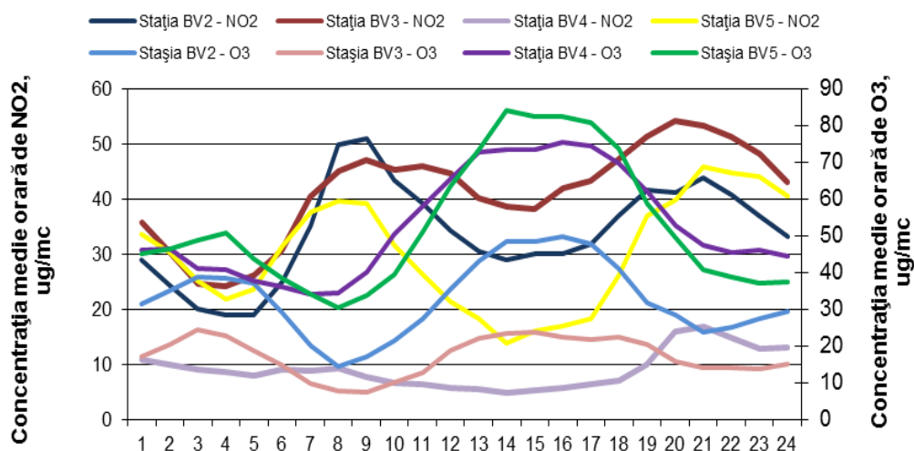
Figura 1.1.2.3.3. Ciclu zilnic al \text{O}_3 și \text{NO}_2
