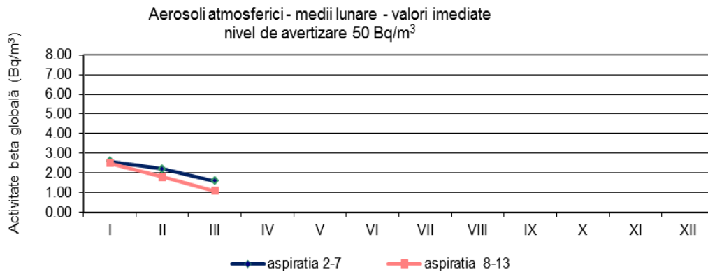
Fig. 1.4.1. Activitatea beta globală pentru aerosoli atmosferici
