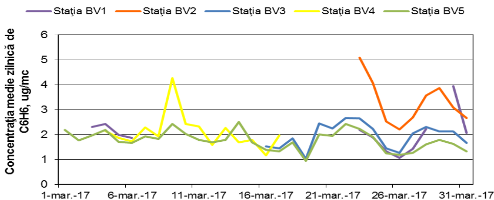
Figura 1.1.2.6.1: Evoluția mediilor zilnice de benzen în luna martie
