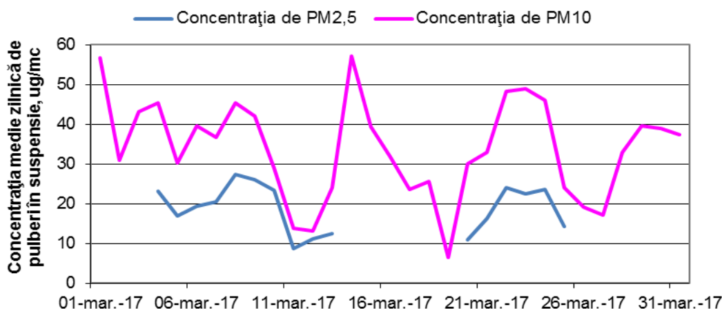
Figura 1.1.2.4.3 Evoluția mediilor zilnice de PM 2,5 și PM10 în luna martie
