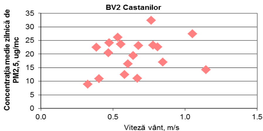
Figura 1.1.2.4.3. Evoluția mediilor zilnice de PM 2,5 în funcție de viteza vântului
