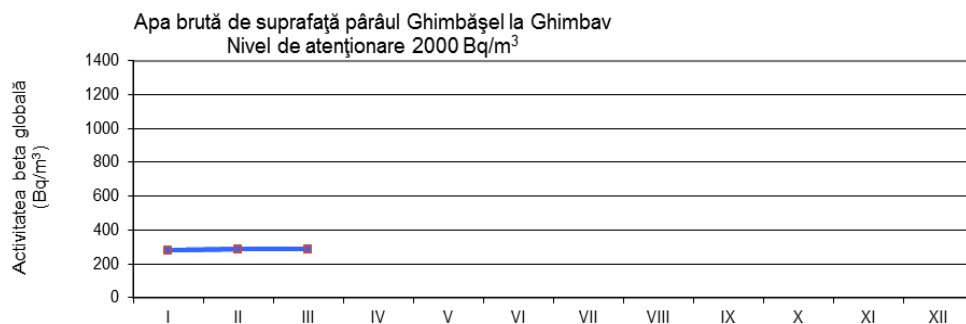
Fig. 1.4.5. Activitatea beta globală imediată pentru apa de suprafață Pârâu Ghimbășel
