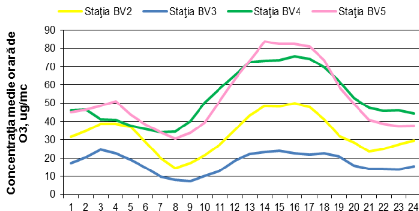
Figura 1.1.2.3.2. Ciclu zilnic al ozonului
