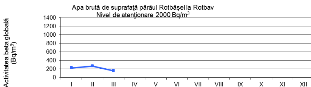
Fig. 1.4.6. Activitatea beta globală – la 5 zile-pentru apa de suprafață-Pârâu Rotbășel
