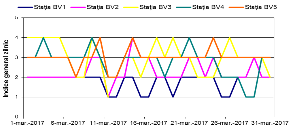
Figura 1.1.2.7.1. Indicele general zilnic de calitatea aerului
