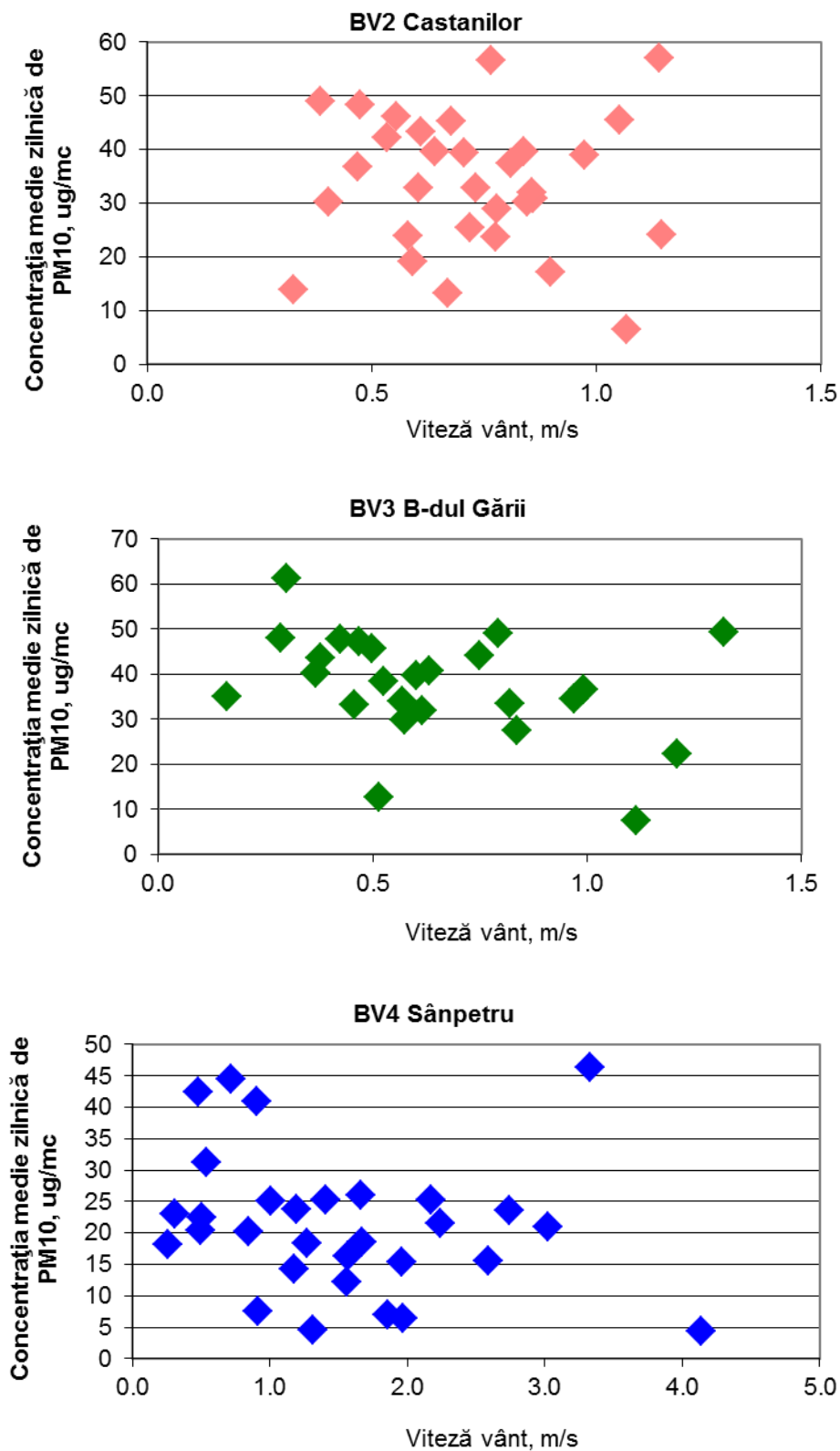
Figura 1.1.2.4.2. Evoluția mediilor zilnice de PM 10 în funcție de viteza vântului la stațiile BV2, BV3 și BV4
