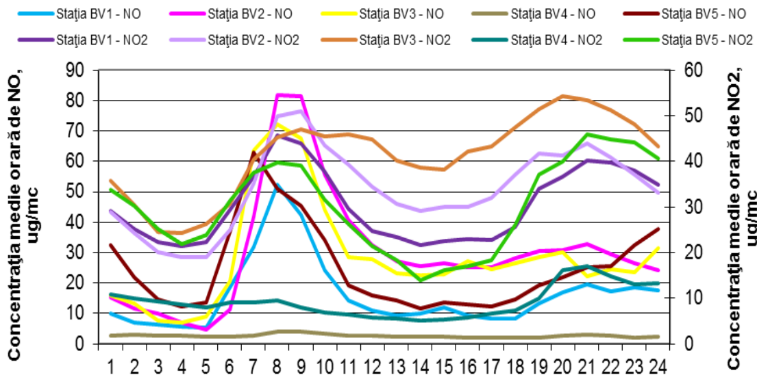
Figura 1.1.2.2.2. Ciclul zilnic al \text{NO}_2 și \text{NO}
