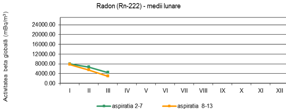
Fig. 1.4.2. Activitatea calculată a Radonului
