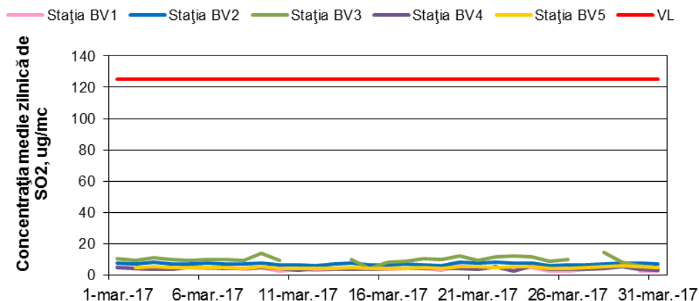
Figura 1.1.2.1.1. Evoluția mediilor zilnice de \text{SO}_2 în luna martie
