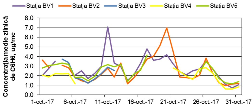
Figura 1.1.2.6.1: Evoluția mediilor zilnice de benzen în luna octombrie
