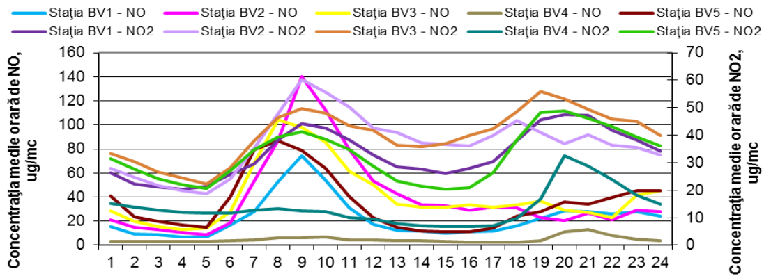
Figura 1.1.2.2.2. Ciclul zilnic al NO 2 și NO
