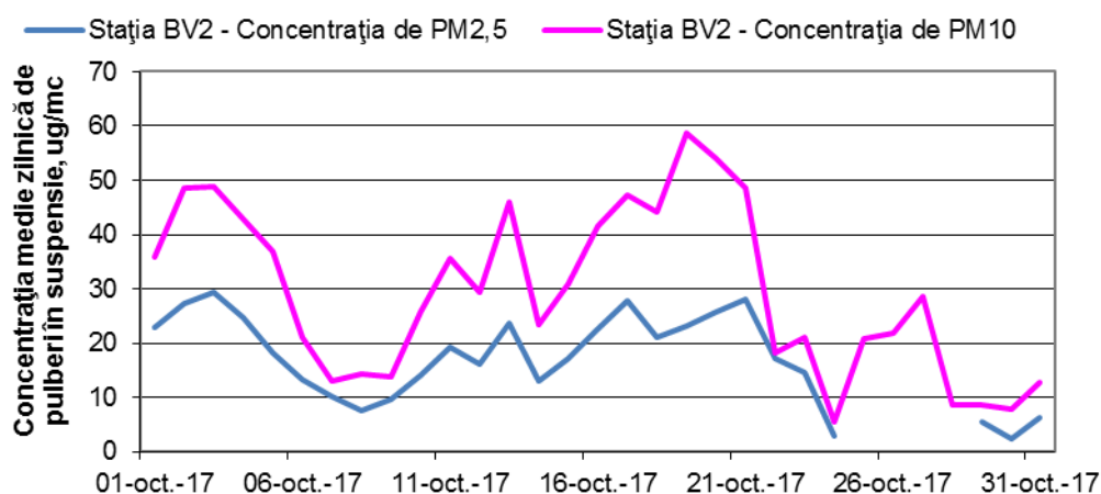
Figura 1.1.2.4.4 Evoluția mediilor zilnice de PM 2,5 și PM10 în luna octombrie
