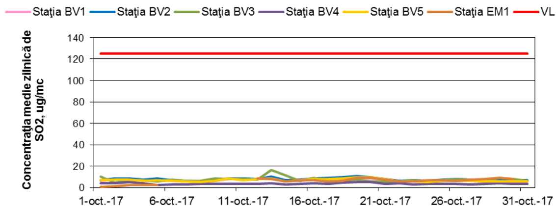
Figura 1.1.2.1.1. Evoluția mediilor zilnice de \text{SO}_2 în luna octombrie
