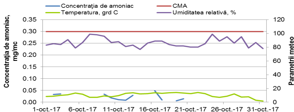
Figura 1.1.1.1.1. Evoluția mediilor de scurtă durată de amoniac în luna octombrie 2017
