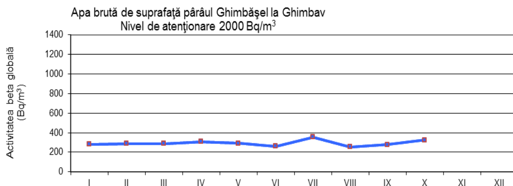
Fig. 1.3.5. Activitatea beta globală imediată pentru apa de suprafață Pârâu Ghimbășel
