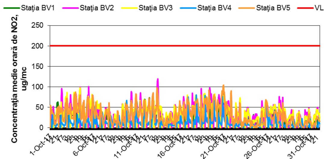
Figura 1.1.2.2.1. Evoluția mediilor orare de \text{NO}_2 în luna octombrie
