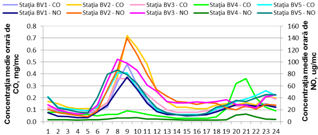
Figura 1.1.2.2.4. Ciclul zilnic al NO și CO
