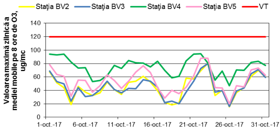
Figura 1.1.2.3.1. Evoluția maximelor zilnice ale mediilor mobile pe 8 ore de \text{O}_3 în luna octombrie
