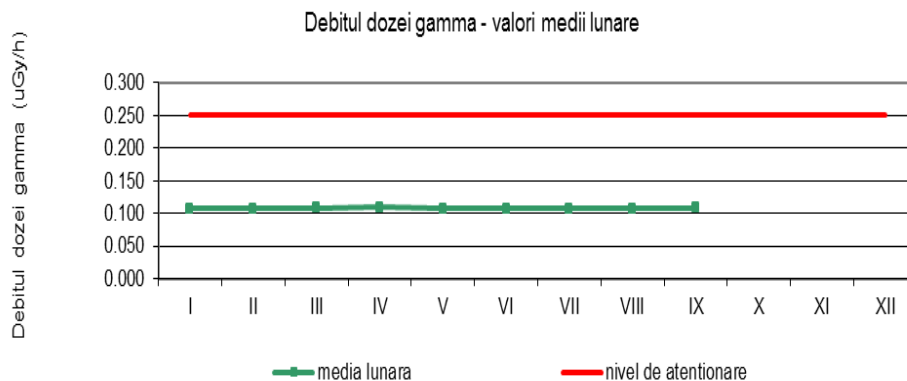
Fig. 1.3.3. Debitul dozei gamma în aer
