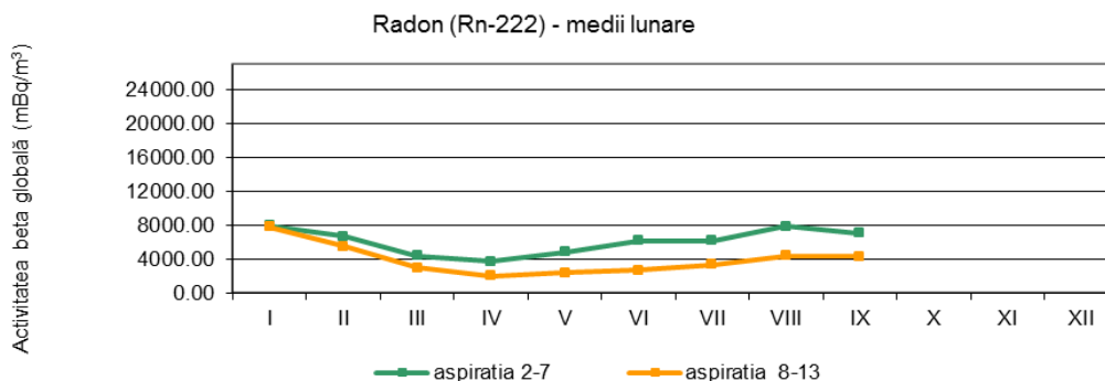
Fig. 1.3.2. Activitatea calculată a Radonului
