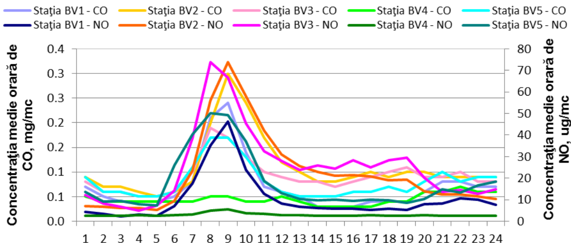
Figura 1.1.2.2.4. Ciclul zilnic al NO și CO
