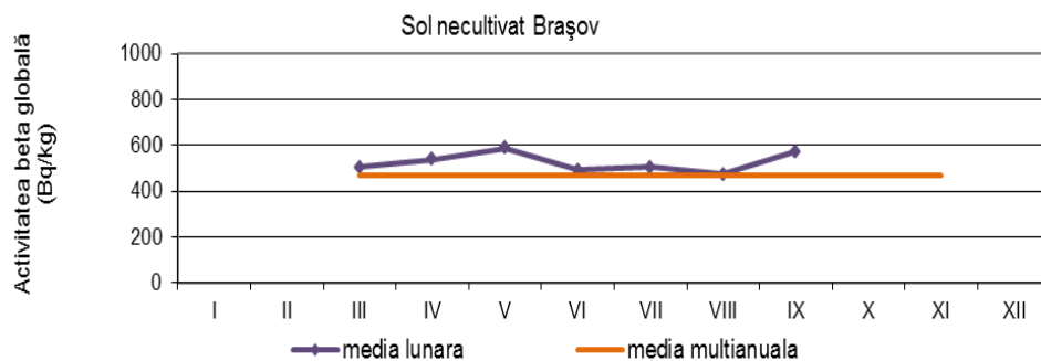
Fig. 1.3.8. Activitatea beta globală – la 5 zile - pentru sol necultivat Brașov.
