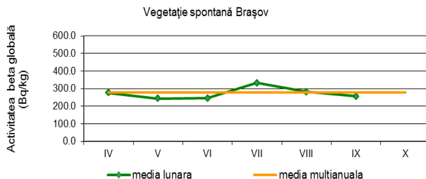
Fig. 1.3.9. Activitatea beta globală – la 5 zile - pentru vegetație Brașov.
