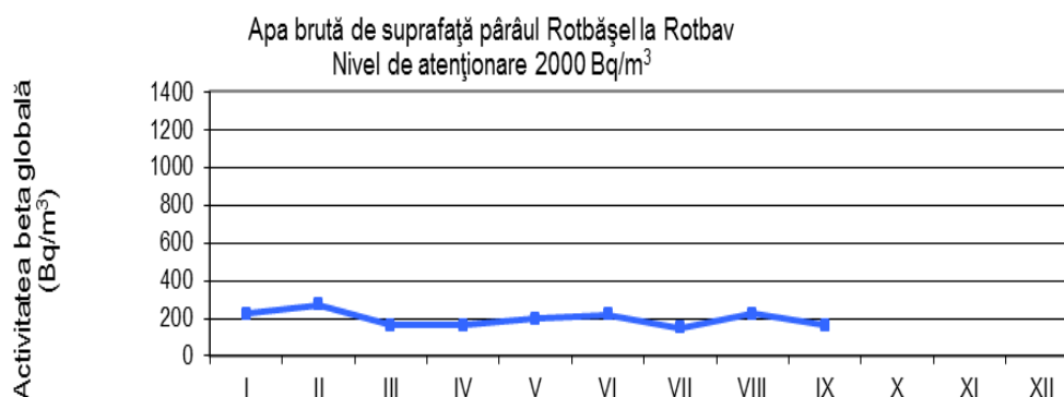
Fig. 1.3.6. Activitatea beta globală – la 5 zile-pentru apa de suprafață-Pârâu Rotbășel
