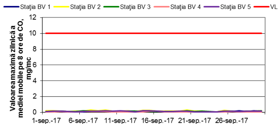
Figura 1.1.2.5.1. Evoluția maximelor zilnice ale mediei mobile de CO în luna septembrie
