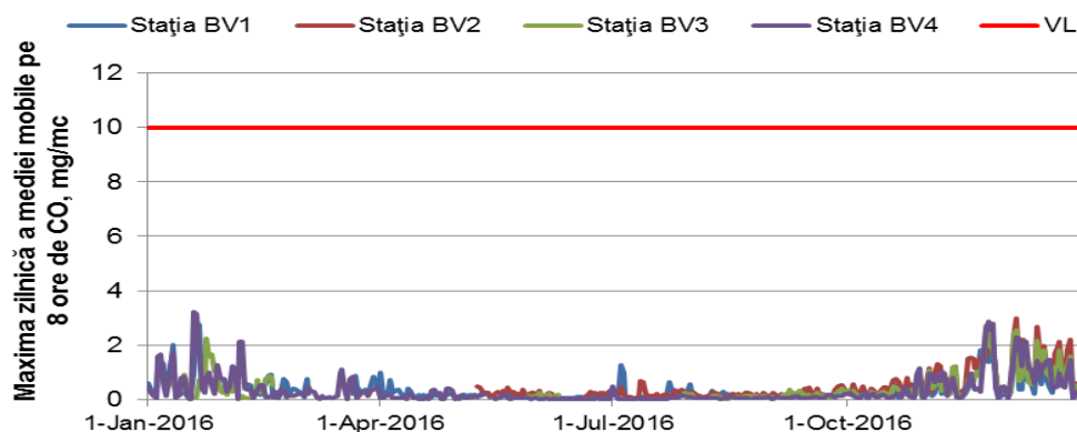
Figura 17: Evoluția valorilor maxime zilnice a mediilor mobile pe 8 ore de CO în anul 2016
