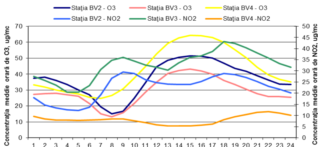
Figura 9: Ciclul zilnic al O_3 și NO_2
