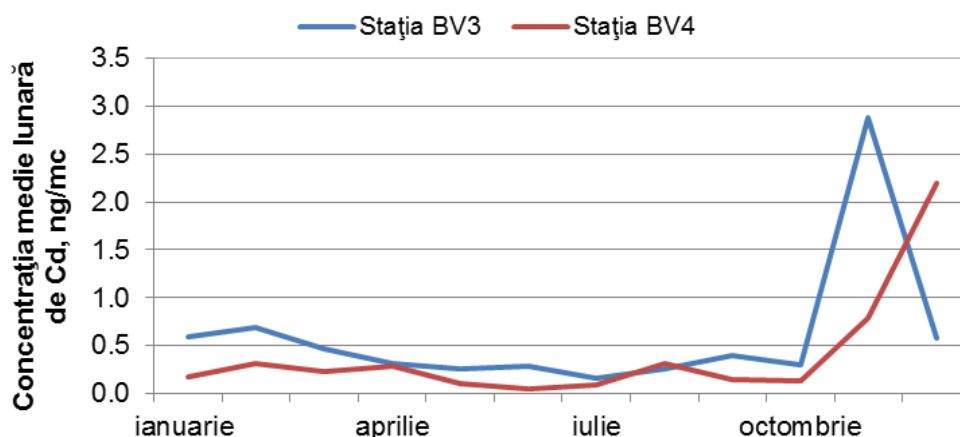
Figura 22: Evoluția mediilor lunare de cadmiu în anul 2016
