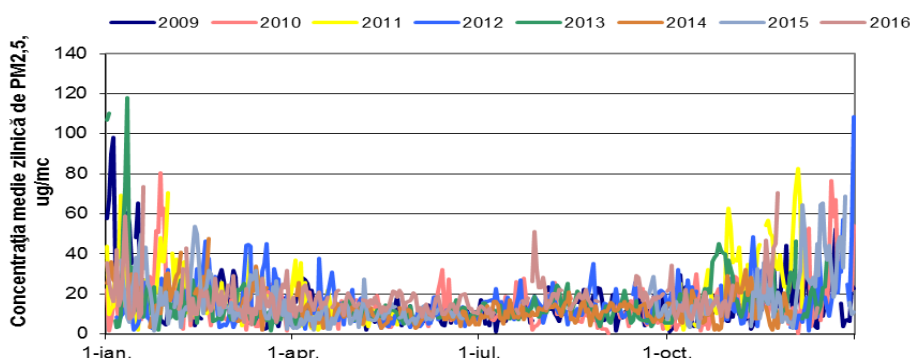
Figura 4: Evoluția mediilor zilnice de PM 2,5
