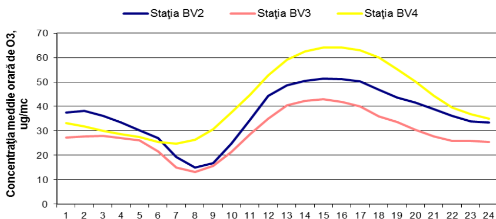
Figura 8: Ciclul zilnic al O_3
