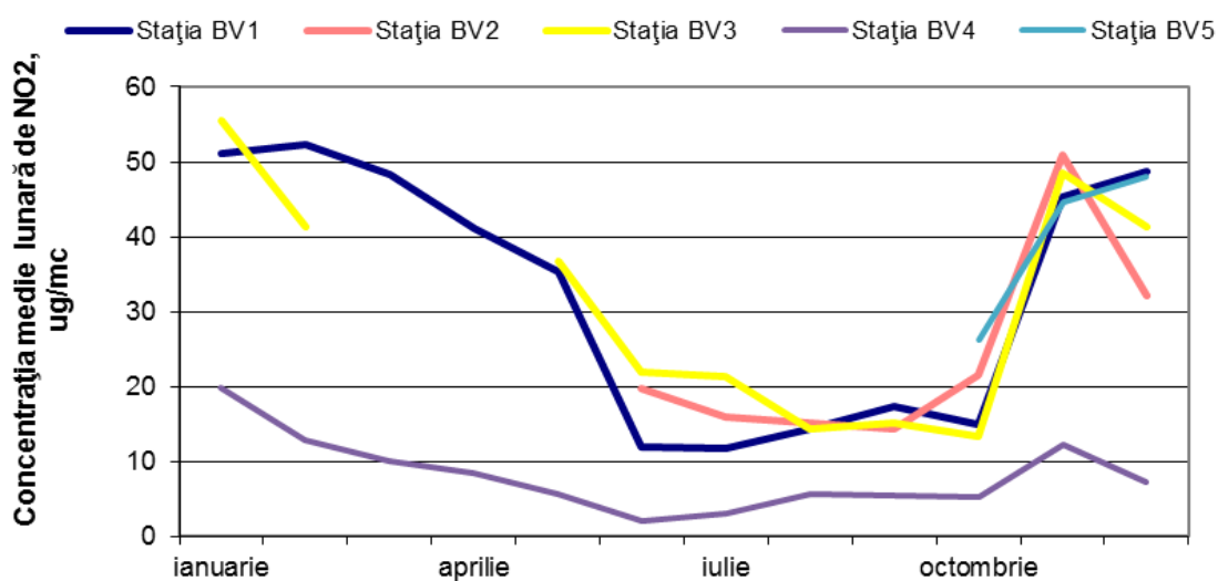
Figura 11: Evoluția concentrației medii lunare de NO 2 în anul 2016
