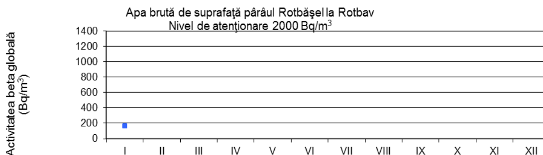
Fig. 1.3.6. Activitatea beta globală la 5 zile pentru apa de suprafață-Pârâu Rotbășel
