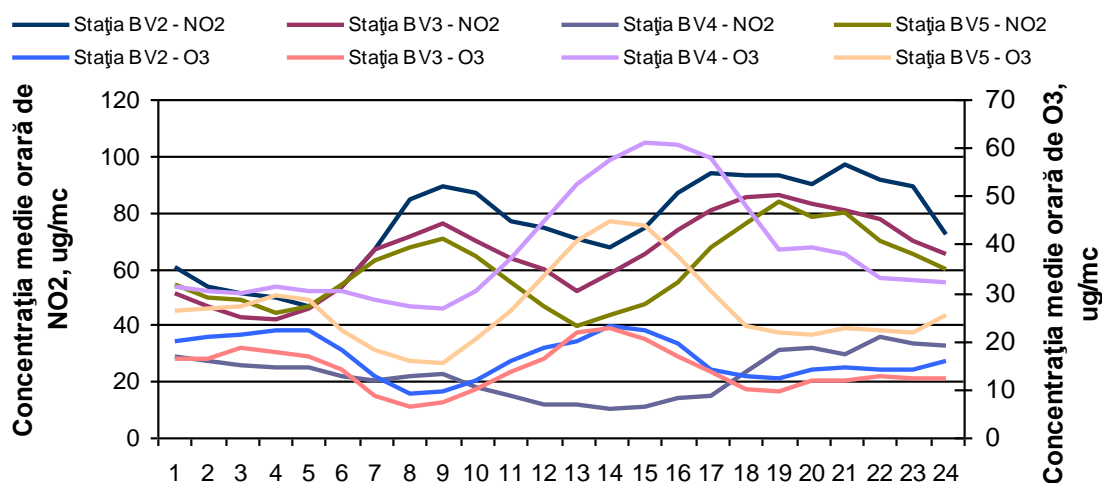
Figura 1.1.2.3.3. Ciclu zilnic al O_3 și NO_2
