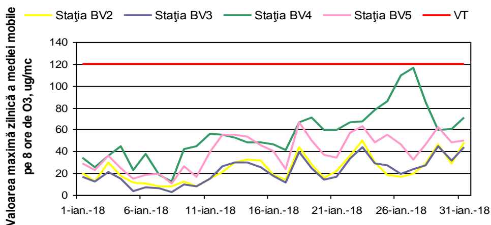
Figura 1.1.2.3.1. Evoluția maximelor zilnice ale mediilor mobile pe 8 ore de \text{O}_3 în luna ianuarie
