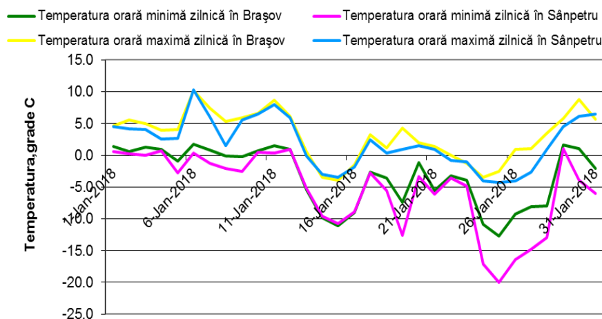
Figura 1.1.2.8.1. Evoluția zilnică a temperaturilor înregistrate în luna ianuarie în stațiile de monitorizare BV2, BV3 și BV5 din Brașov ( 555 m altitudine) și BV4 din Sânpetru ( 515 m altitudine)
