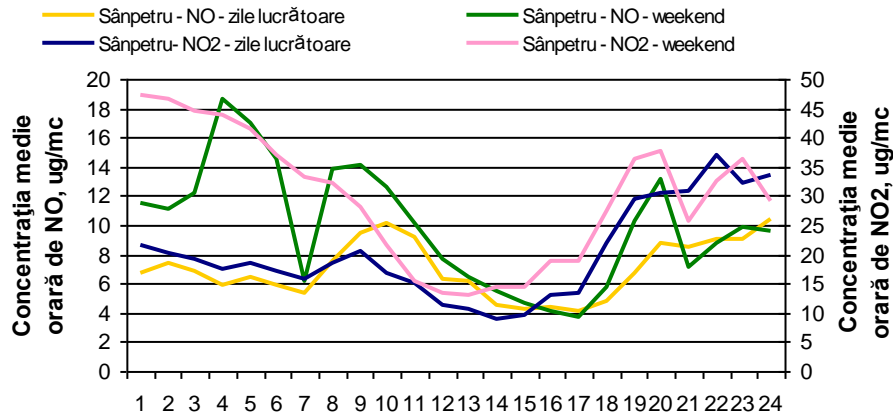
Figura 1.1.2.2.3. Ciclu zilnic al oxizilor de azot în timpul săptămânii
