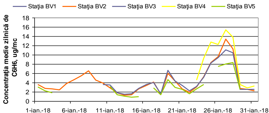
Figura 1.1.2.6.1: Evoluția mediilor zilnice de benzen în luna ianuarie
