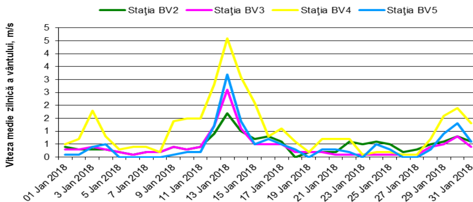
Figura 1.1.2.8.5. Viteza vântului înregistrată în luna ianuarie la stațiile de monitorizare BV2, BV3 și BV5 din Brașov și BV4 din Sânpetru
