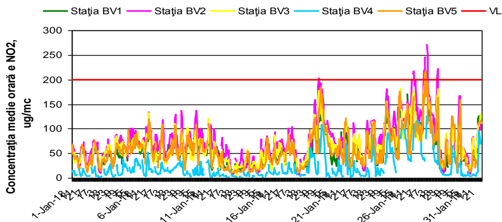
Figura 1.1.2.2.1. Evoluția mediilor orare de NO 2 în luna ianuarie
