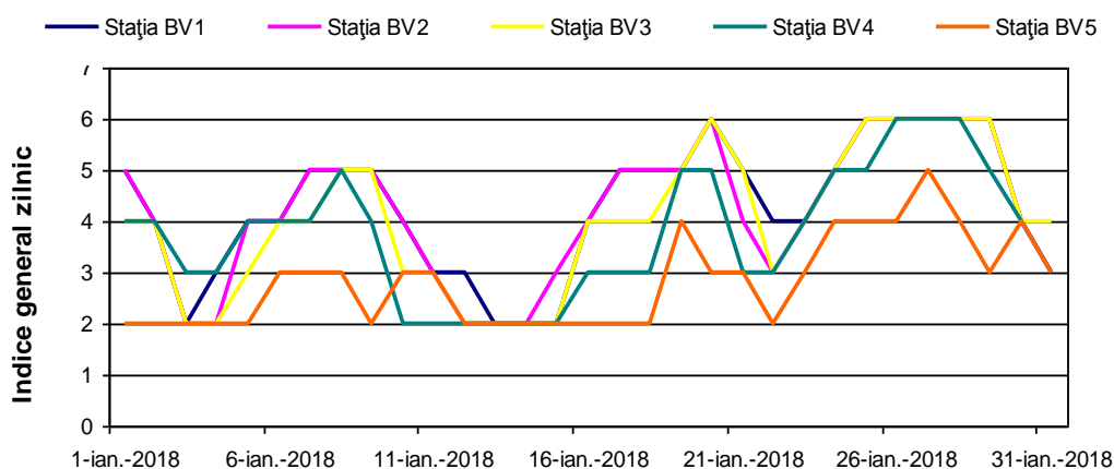
Figura 1.1.2.7.1. Indicele general zilnic de calitatea aerului
