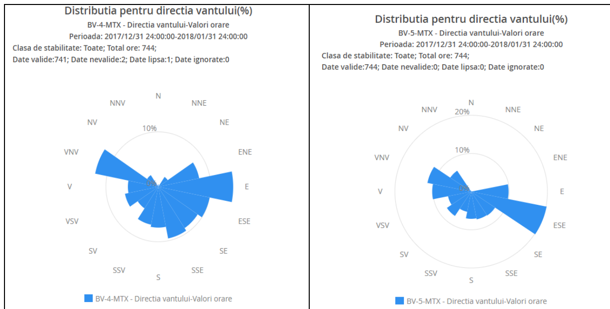
Figura 1.1.2.8.4. Direcția vântului înregistrată în luna ianuarie la stațiile de monitorizare BV2, BV3 și BV5 din Brașov și BV4 din Sânpetru
