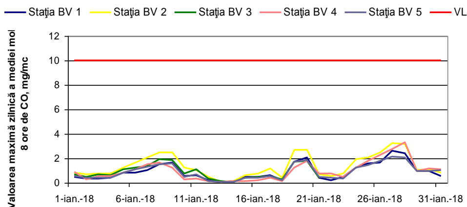
Figura 1.1.2.5.1. Evoluția maximelor zilnice ale mediei mobile de CO în luna ianuarie
