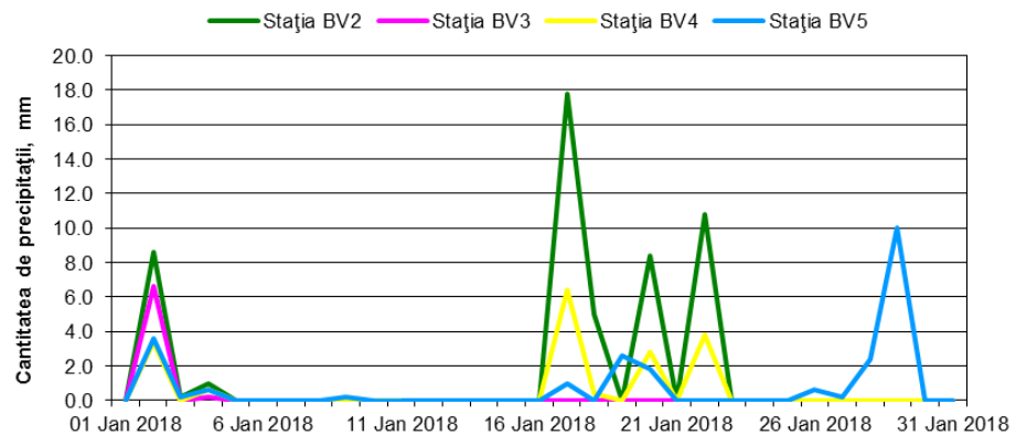
Figura 1.1.2.8.3. Evoluția zilnică a precipitațiilor înregistrate în luna ianuarie în stațiile de monitorizare BV2, BV3 și BV5 din Brașov și BV4 din Sânpetru
