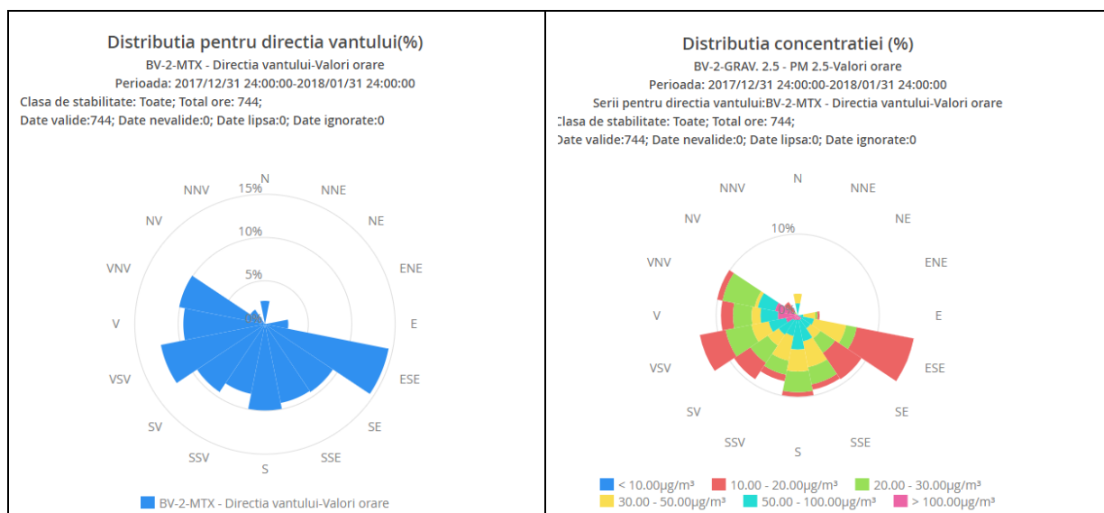
Figura 1.1.2.8.7. Grafic vânt și vânt – concentrație de PM 2,5 la stația BV2 în luna ianuarie 2018
