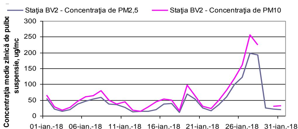
Figura 1.1.2.4.4 Evoluția mediilor zilnice de PM 2,5 și PM10 în luna ianuarie
