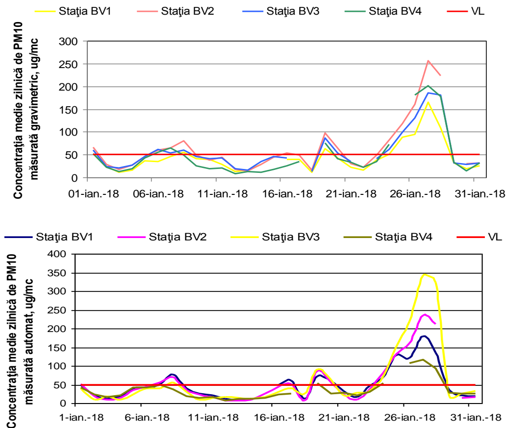
Figura 1.1.2.4.1. Evoluția mediilor zilnice de PM 10 în luna ianuarie
