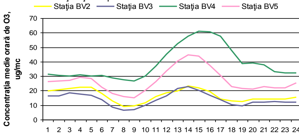
Figura 1.1.2.3.2. Ciclul zilnic al ozonului
