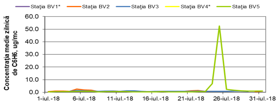
Figura 1.1.2.6.1: Evoluția mediilor zilnice de benzen în luna iulie
