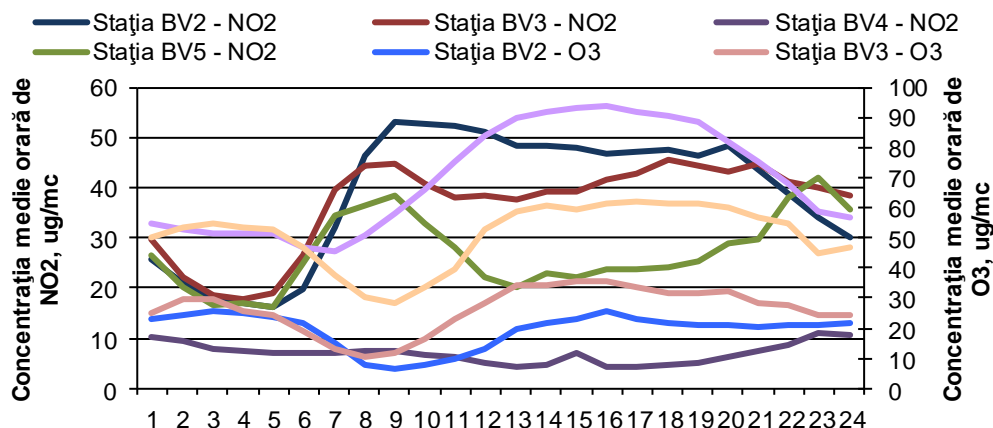
Figura 1.1.2.3.3. Ciclu zilnic al O 3 și NO 2
