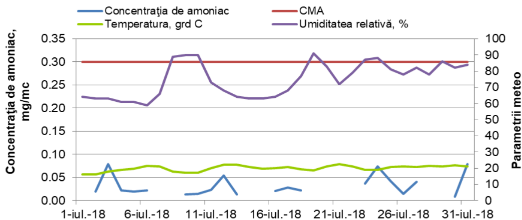
Figura 1.1.1.1.1. Evoluția mediilor de scurtă durată de amoniac în luna iulie 2018
