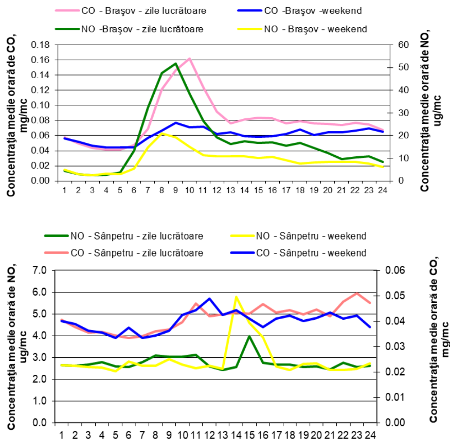
Figura 1.1.2.2.5. Ciclul zilnic al NO și CO în timpul săptămânii
