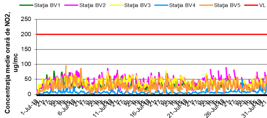
Figura 1.1.2.2.1. Evoluția mediilor orare de NO 2 în luna iulie
