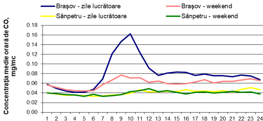
Figura 1.1.2.5.3. Ciclul zilnic al CO în timpul săptămânii
