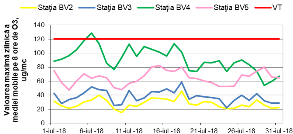
Figura 1.1.2.3.1. Evoluția maximelor zilnice ale mediilor mobile pe 8 ore de \text{O}_3 în luna iulie
