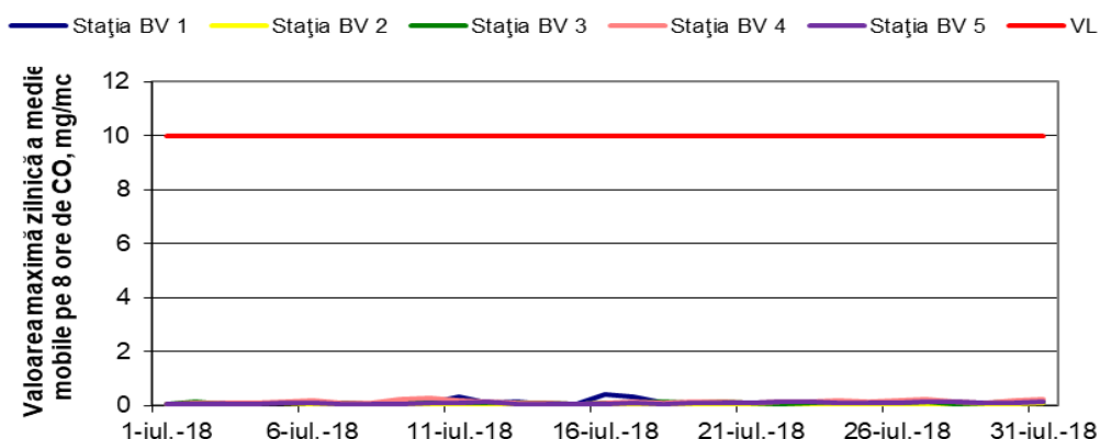
Figura 1.1.2.5.1. Evoluția maximelor zilnice ale mediei mobile de CO în luna iulie
