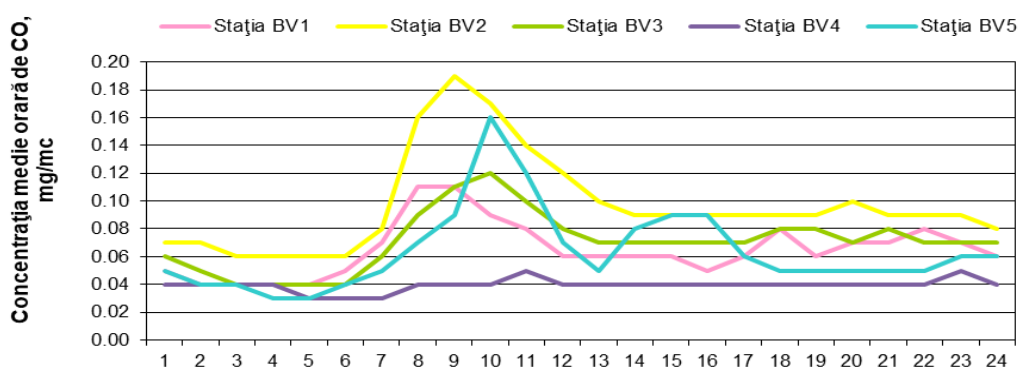
Figura 1.1.2.5.2. Ciclul zilnic al CO
