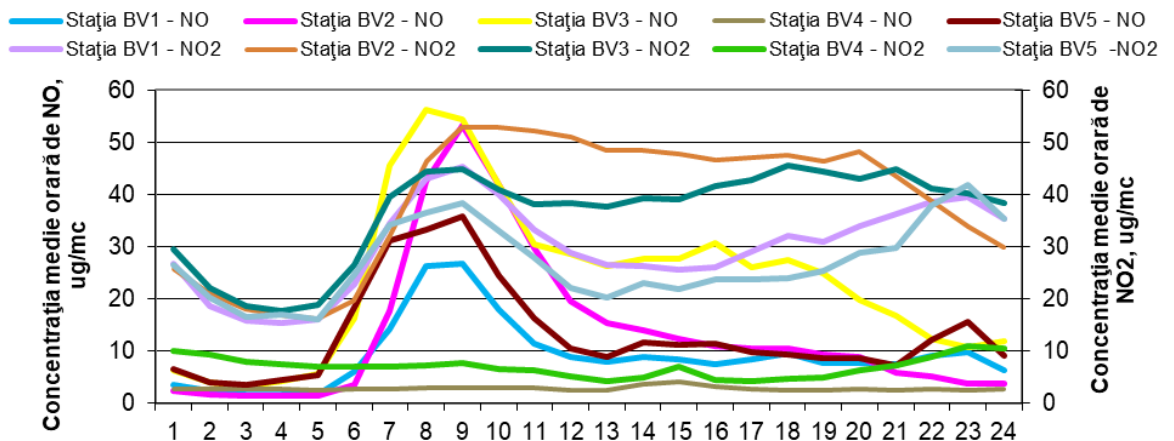
Figura 1.1.2.2.2. Ciclul zilnic al NO 2 și NO
