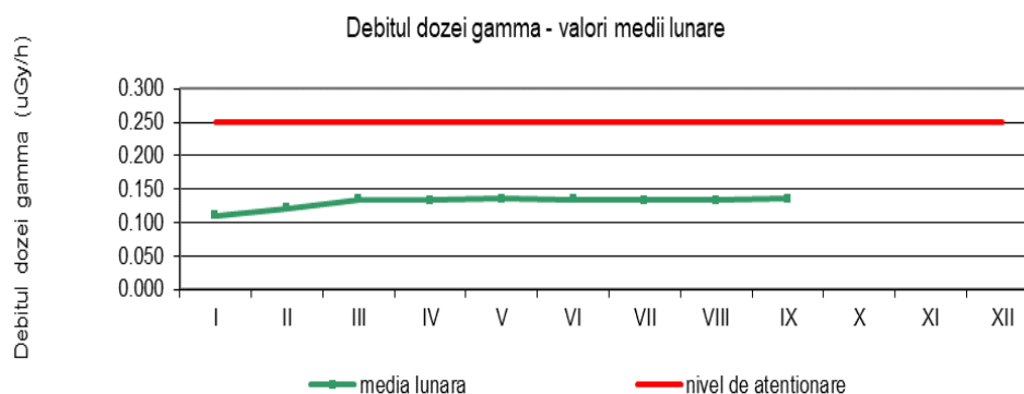
Fig. 1.3.3. Debitul dozei gamma în aer
