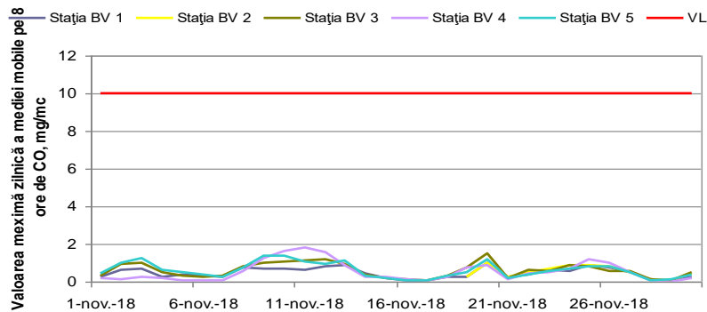
Figura 1.1.2.5.1. Evoluția maximelor zilnice ale mediei mobile de CO în luna noiembrie
