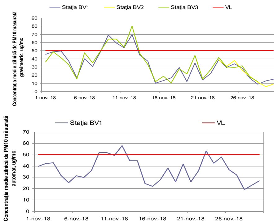
Figura 1.1.2.4.1. Evoluția mediilor zilnice de PM 10 în luna noiembrie
