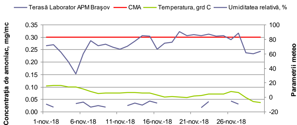
Figura 1.1.1.1.1. Evoluția mediilor de scurtă durată de amoniac în luna noiembrie 2018
