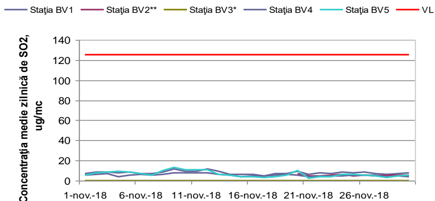
Figura 1.1.2.1.1. Evoluția mediilor zilnice de SO 2 în luna noiembrie
