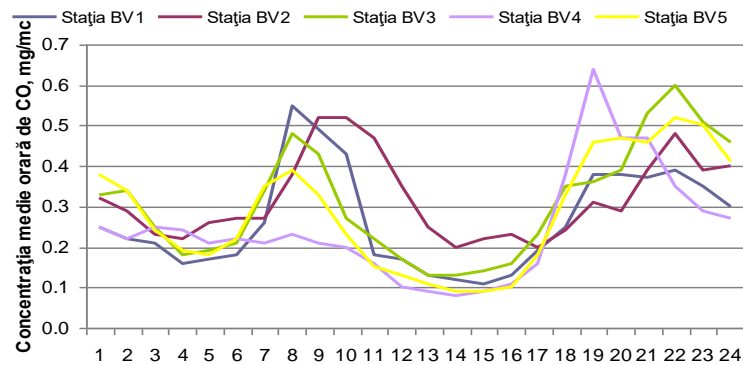
Figura 1.1.2.5.2. Ciclul zilnic al CO
