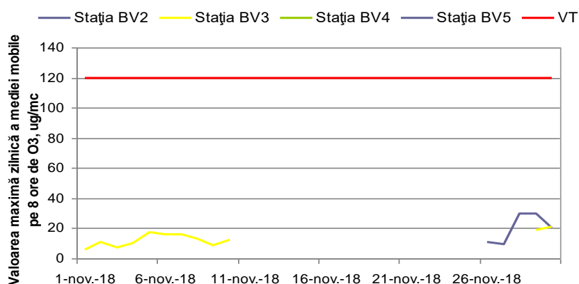
Figura 1.1.2.3.1. Evoluția maximelor zilnice ale mediilor mobile pe 8 ore de \text{O}_3 în luna noiembrie
