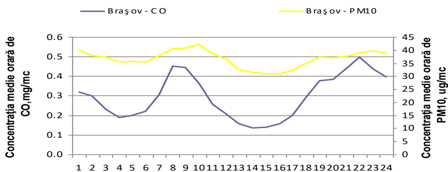
Figura 1.1.2.4.3: Ciclul zilnic al PM 10 și CO
