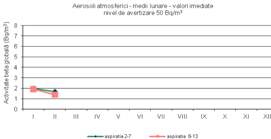
Fig. 1.4.1. Activitatea beta globală pentru aerosoli atmosferici
