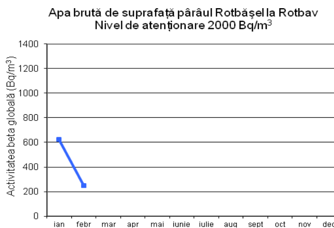
Fig. 1.4.6. Activitatea beta globală –la 5 zile-pentru apa de suprafață-Pârâu Rotbășel
