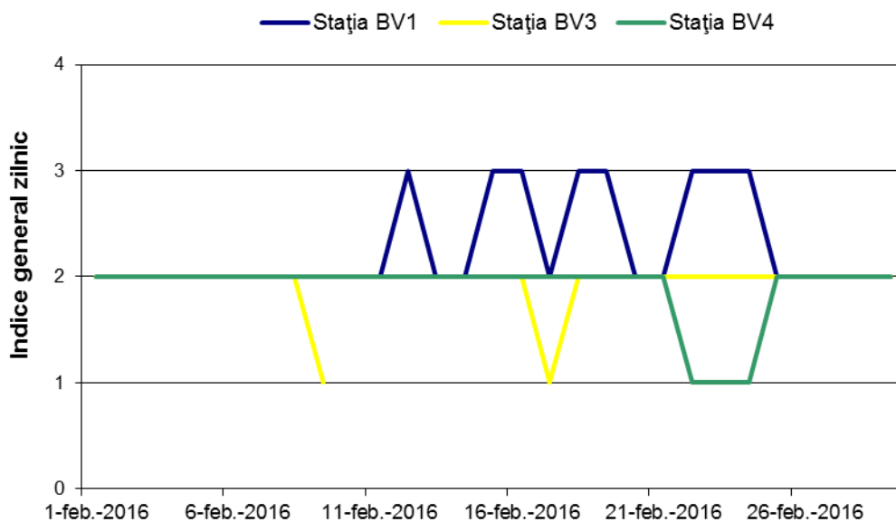
Figura 1.1.2.7.1. Indicele general zilnic de calitatea aerului
