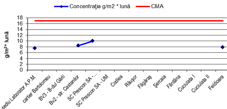
Figura 1.1.1.2. Cantitatea de pulberi sedimentabile în județul Brașov
