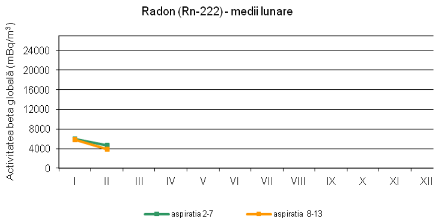
Fig. 1.4.2. Activitatea calculată a Radonului
