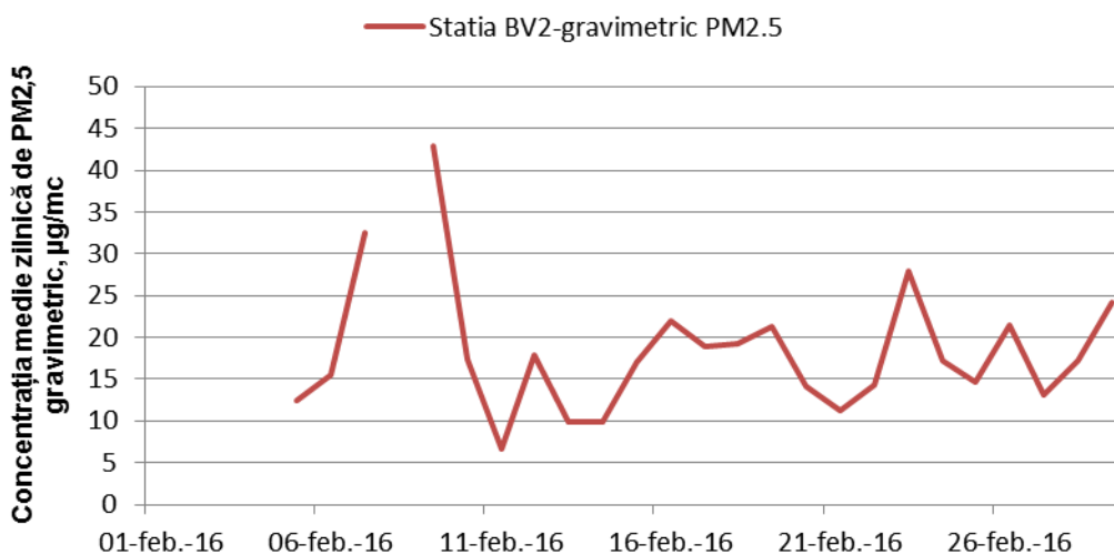
Figura 1.1.2.4.2 Evoluția mediilor zilnice de PM 2,5 în luna februarie
