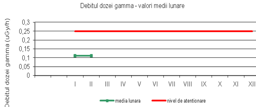
Fig. 1.4.3. Debitul dozei gamma în aer
