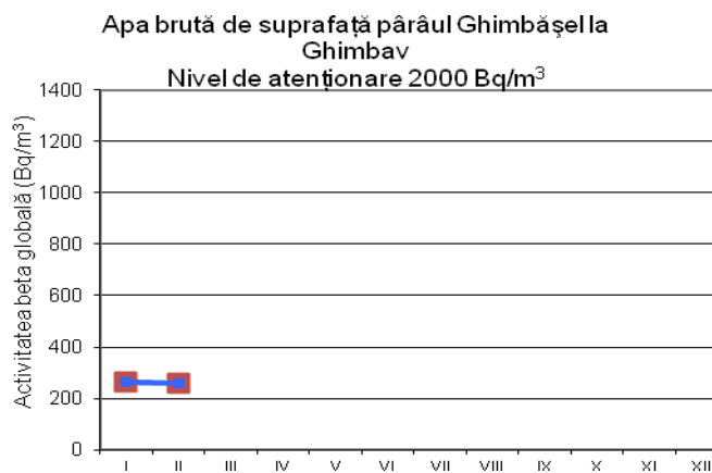
Fig. 1.4.5. Activitatea beta globală imediată pentru apa de suprafață Pârâu Ghimbășel Proba de apă brută de suprafață se prelevează lunar din Pârâul Rotbășel -la Rotbav. Valoarea activității beta globale măsurată în luna februarie este mai mică decât cea măsurată luna trecută, fiind situată sub nivelurile de notificare.
