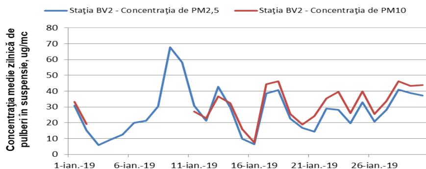
Figura 1.1.2.4.4 Evoluția mediilor zilnice de PM 2,5 și PM10 în luna ianuarie
