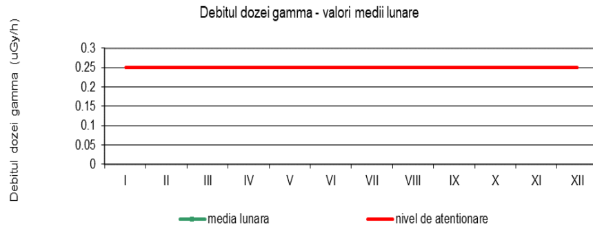
Fig. 1.3.3. Debitul dozei gamma în aer
