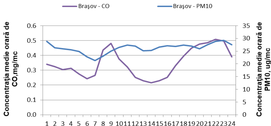
Figura 1.1.2.4.3: Ciclul zilnic al PM10 și CO
