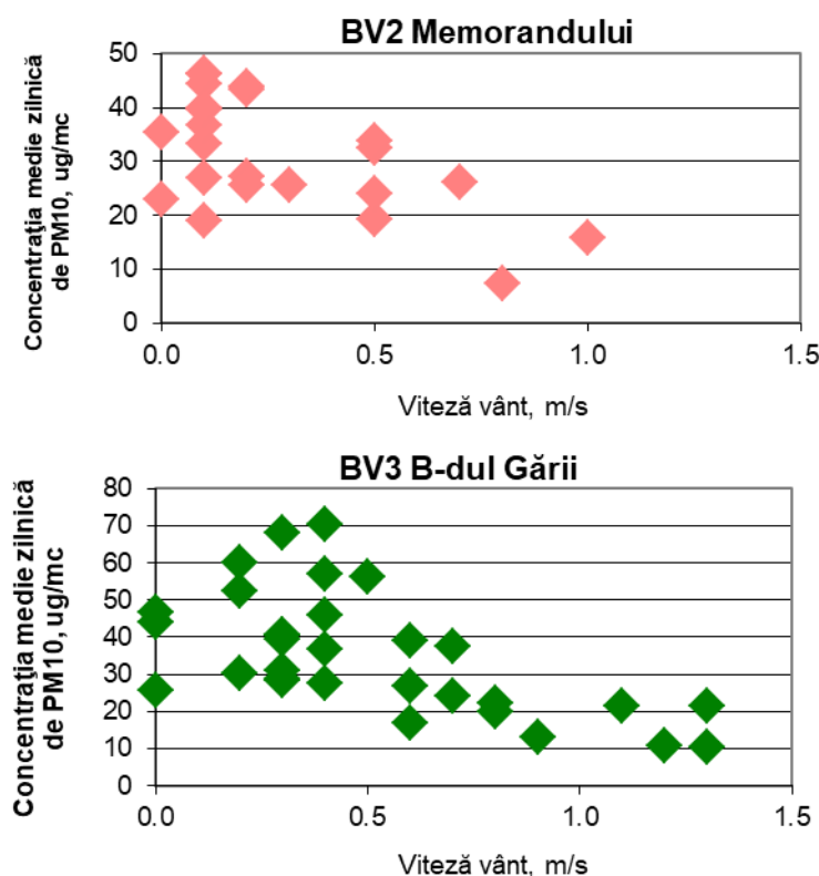
Figura 1.1.2.4.2. Evoluția mediilor zilnice de PM 10 în funcție de viteza vântului la stațiile BV2 și BV3
