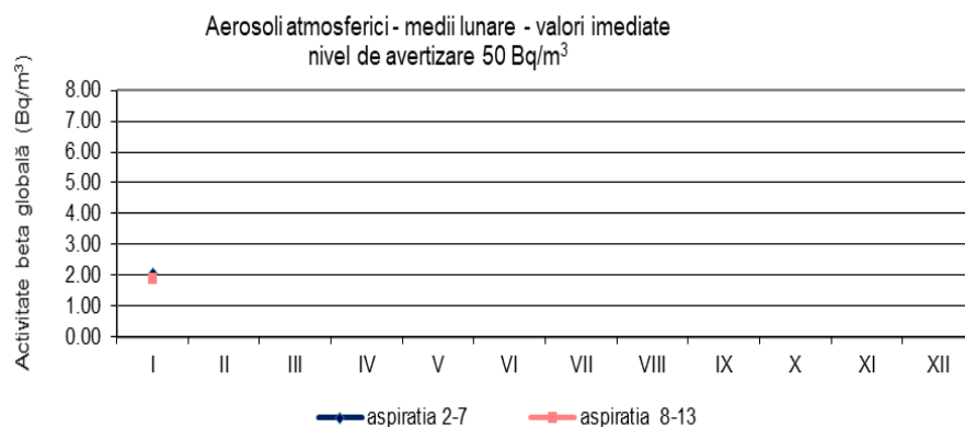
Fig. 1.3.1. Activitatea beta globală pentru aerosoli atmosferici
