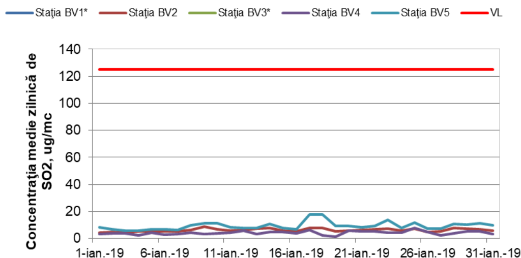
Figura 1.1.2.1.1. Evoluția mediilor zilnice de \text{SO}_2 în luna ianuarie
