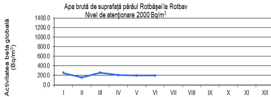
Fig. 1.3.6. Activitatea beta globală la 5 zile pentru apa de suprafață-Pârâul Rotbășel
