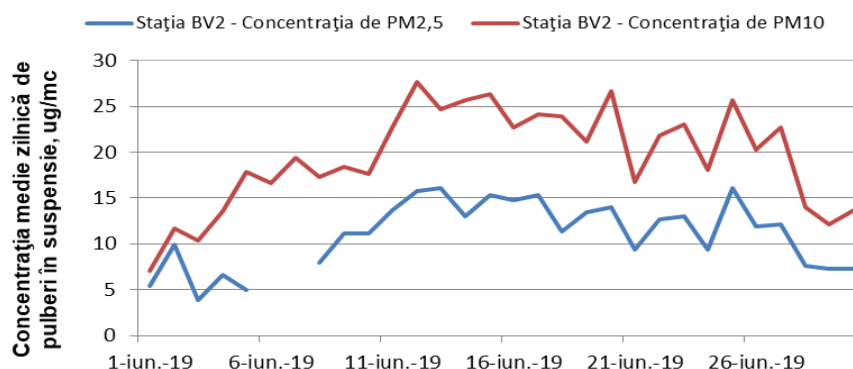
Figura 1.1.2.4.4 Evoluția mediilor zilnice de PM 2,5 și PM 10 în luna iunie
