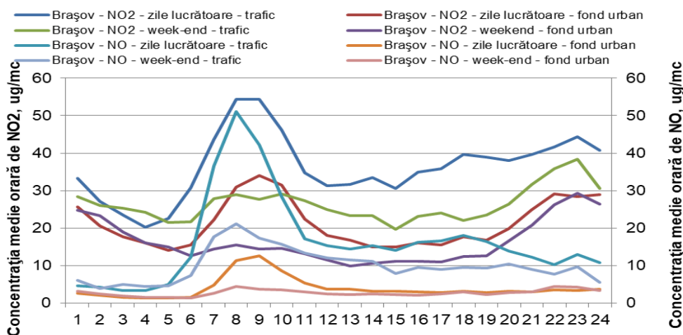
Figura 1.1.2.2.3. Ciclu zilnic al oxizilor de azot în timpul săptămânii
