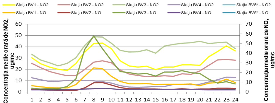
Figura 1.1.2.2.2. Ciclu zilnic al NO 2 și NO
