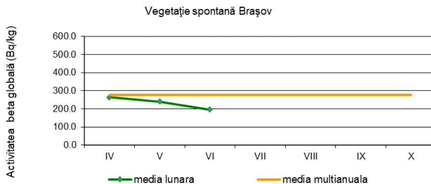
Fig. 1.3.9. Activitatea beta globală la 5 zile pentru vegetația spontană
