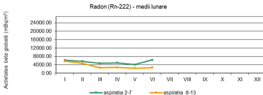
Fig. 1.3.2. Activitatea calculată a Radonului
