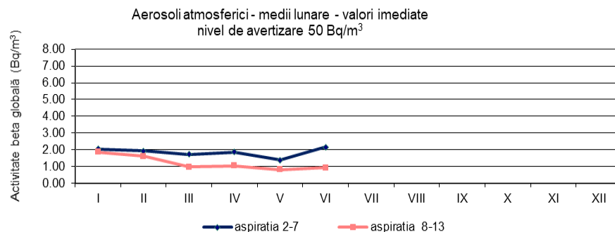
Fig. 1.3.1. Activitatea beta globală pentru aerosoli atmosferici
