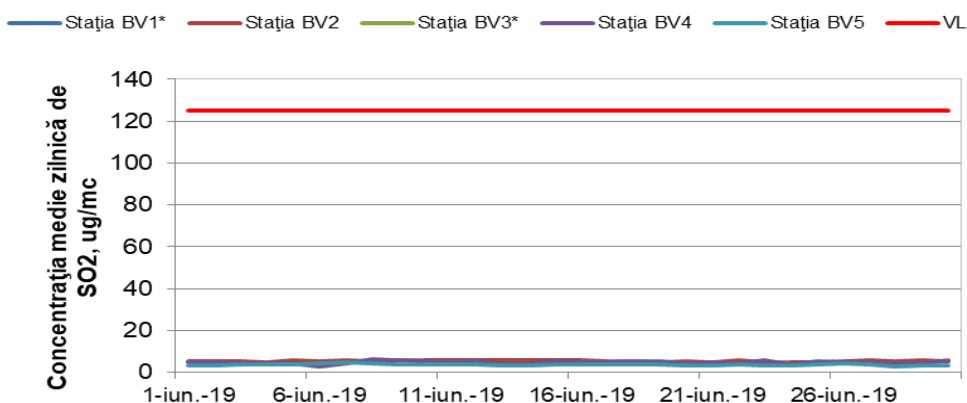
Figura 1.1.2.1.1. Evoluția mediilor zilnice de \text{SO}_2 în luna iunie
