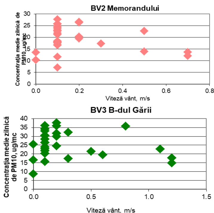
Figura 1.1.2.4.2. Evoluția mediilor zilnice de PM 10 în funcție de viteza vântului la stațiile BV2 și BV3
