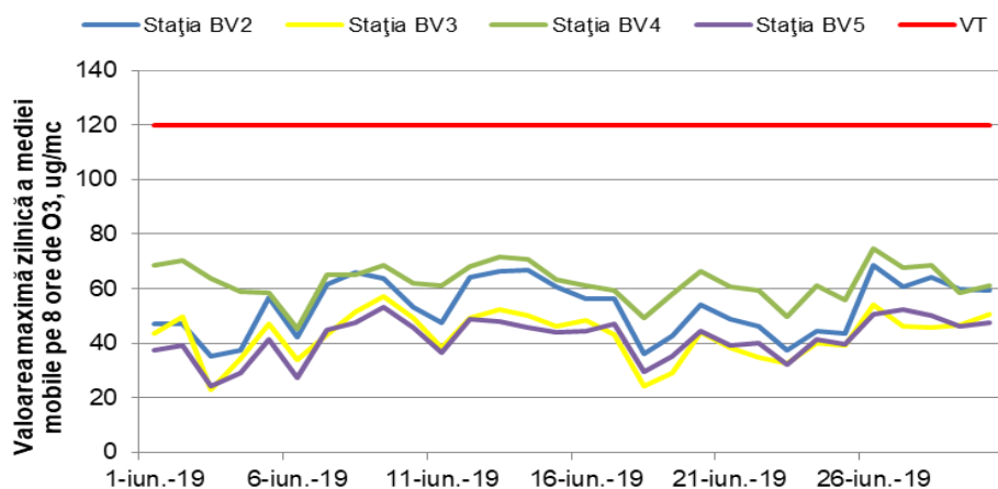
Figura 1.1.2.3.1. Evoluția maximelor zilnice ale mediilor mobile pe 8 ore de O 3 în luna iunie
