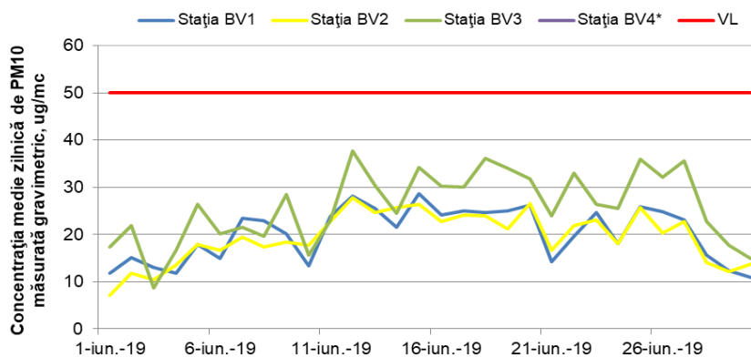
Figura 1.1.2.4.1. Evoluția mediilor zilnice de PM 10 în luna iunie
