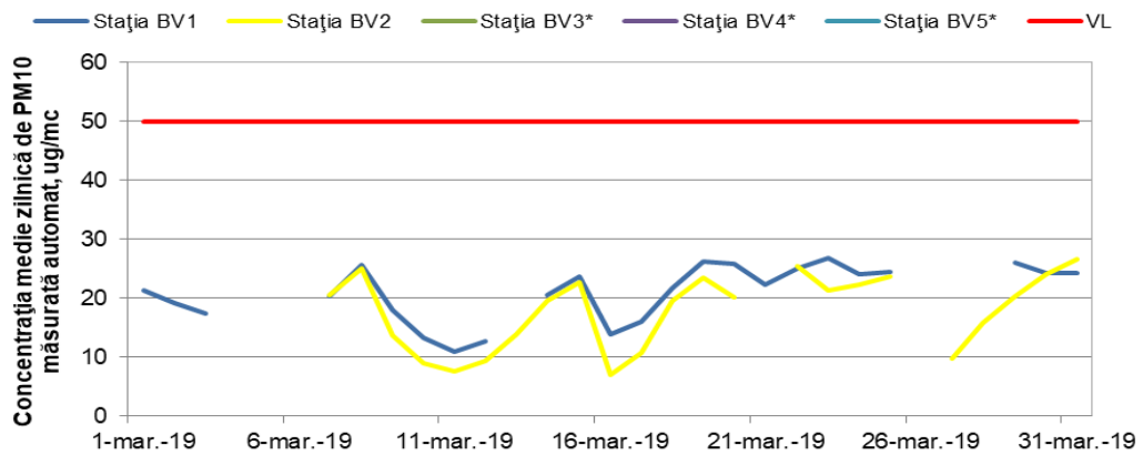
*În stațiile BV3, BV4 și BV5 nu s-au efectuat măsurări automate de PM10 Figura 1.1.2.4.1. Evoluția mediilor zilnice de PM 10 în luna martie
