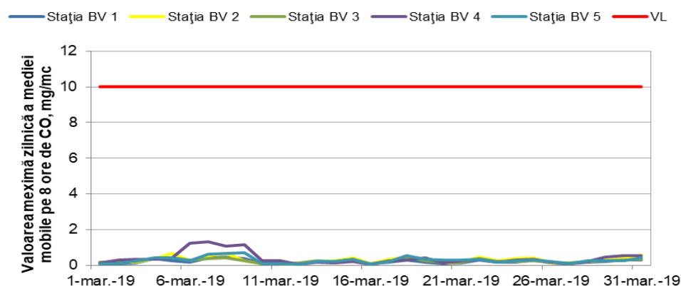
Figura 1.1.2.5.1. Evoluția maximelor zilnice ale mediei mobile de CO în luna martie
