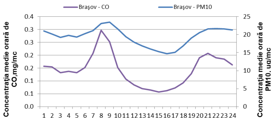
Figura 1.1.2.4.3: Ciclul zilnic al PM10 și CO
