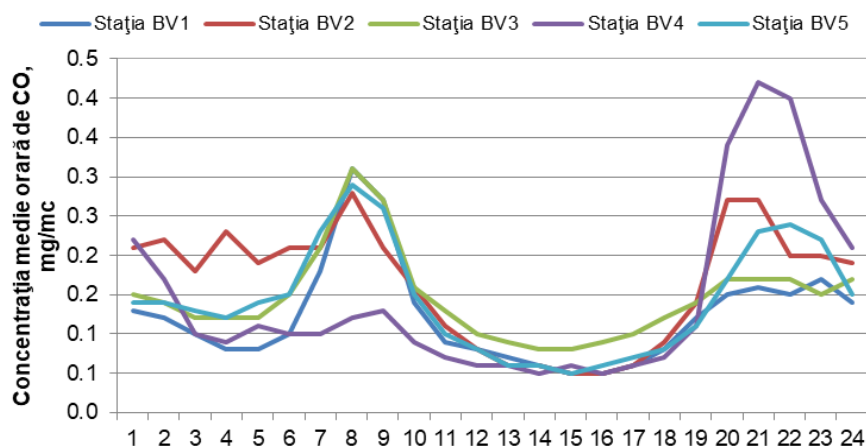
Figura 1.1.2.5.2. Ciclul zilnic al CO
