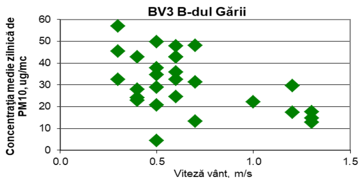
Figura 1.1.2.4.2. Evoluția mediilor zilnice de PM 10 în funcție de viteza vântului la stațiile BV2 și BV3
