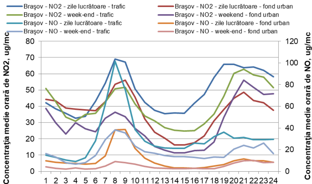
Figura 1.1.2.2.3. Ciclul zilnic al oxizilor de azot în timpul săptămânii
