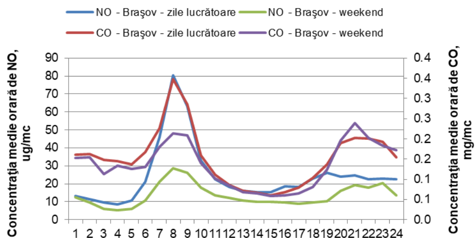
Figura 1.1.2.2.5. Ciclul zilnic al NO și CO în timpul săptămânii
