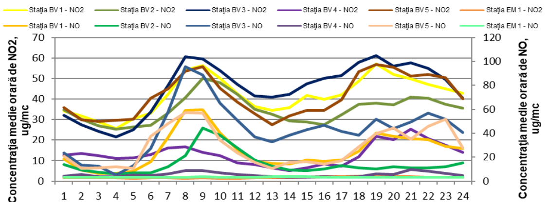
Figura 1.1.2.2.2. Ciclul zilnic al NO 2 și NO
