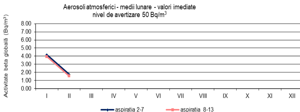
Fig. 1.3.1. Activitatea beta globală pentru aerosoli atmosferici
