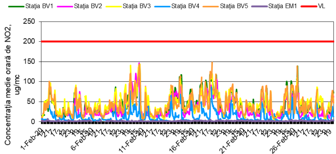
Figura 1.1.2.2.1. Evoluția mediilor orare de NO 2 în luna februarie
