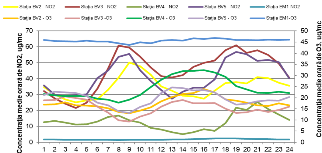
Figura 1.1.2.3.3. Ciclul zilnic al O_3 și NO_2
