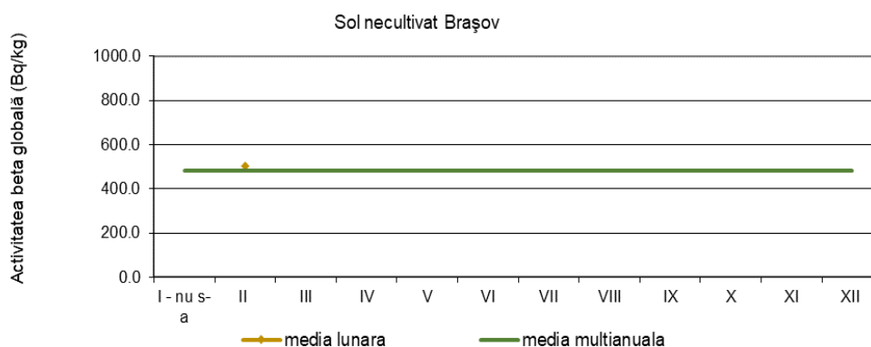
Fig. 1.3.8. Activitatea beta globală la 5 zile pentru solul necultivat
