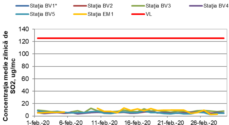
Figura 1.1.2.1.1. Evoluția mediilor zilnice de \text{SO}_2 în luna februarie
