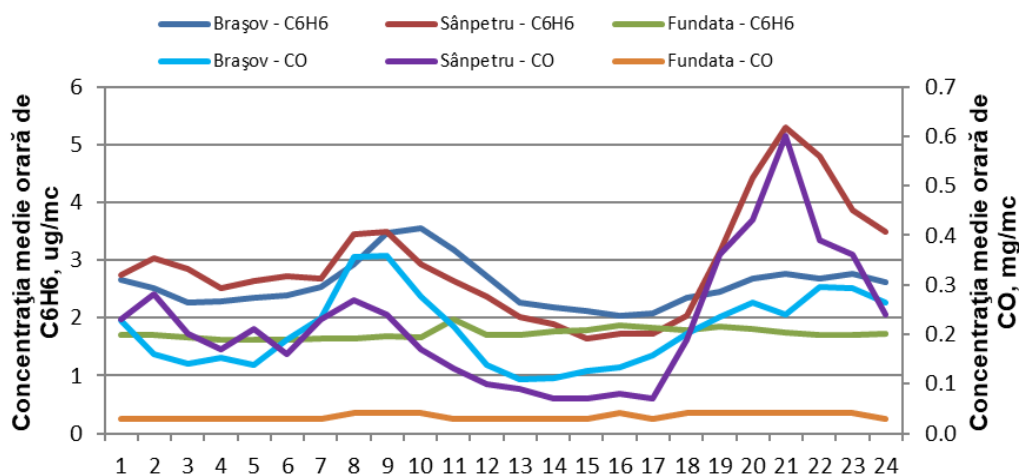
Figura 1.1.2.6.2: Ciclul zilnic al CO și benzenului în Brașov
